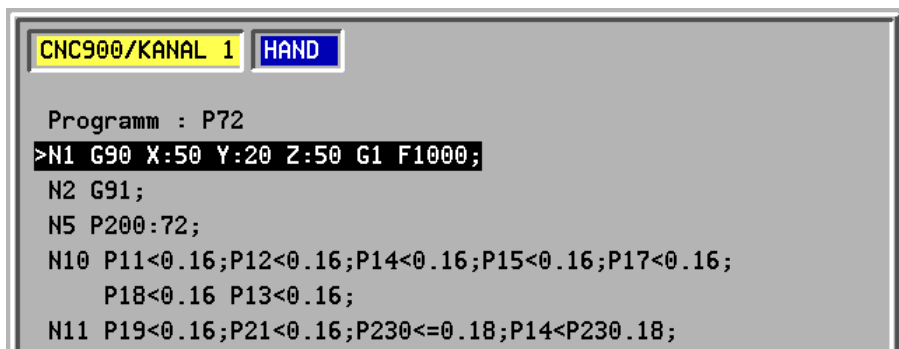
NC-Sätze anwählen
