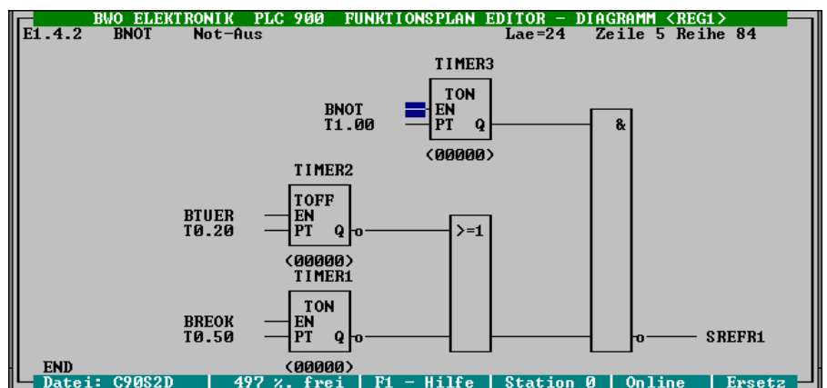
Funktionsplan
