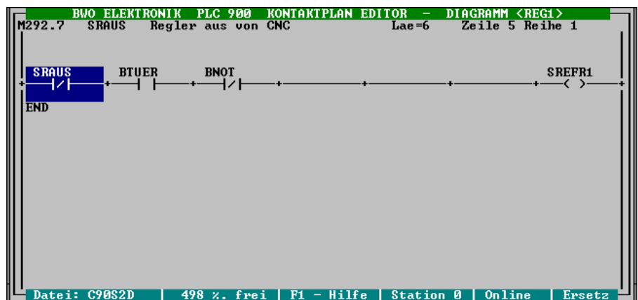
Kontaktplan
