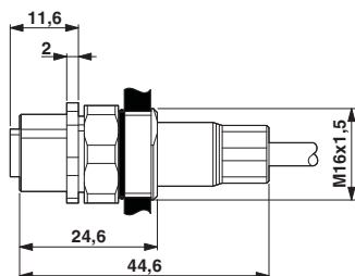
M12-Einbaubuchse, positionierbar
