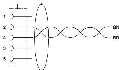
Kontaktbelegung der M12-Buchse
