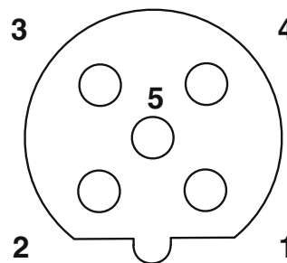
Polbild Buchse M12, 5-polig, B-kodiert, Ansicht Buchsenseite
