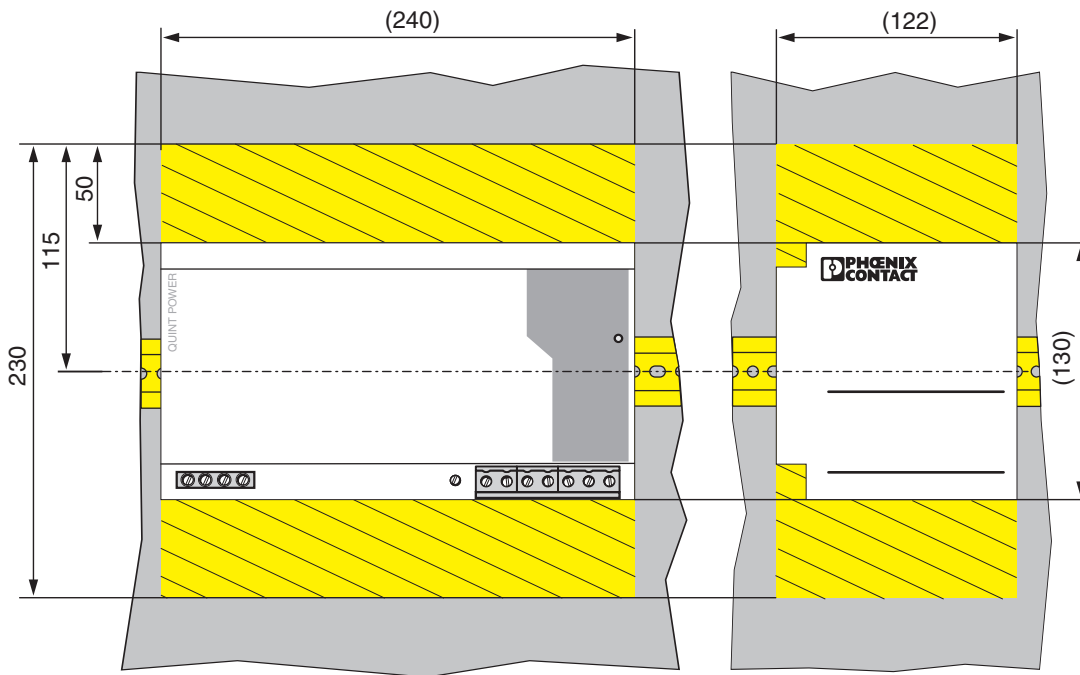
Bild 4 Einbaulage (Maße in mm)
