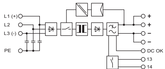
Bild 2 Blockschaltbild
