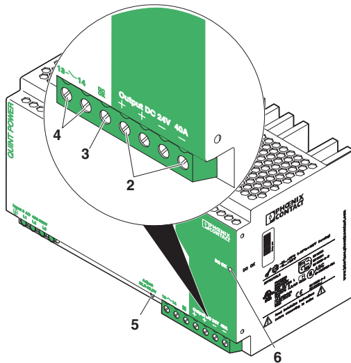
Bild 9 Ausgang
