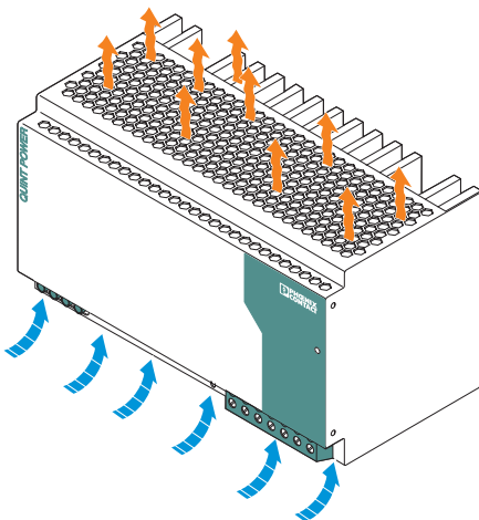
Bild 3 Konvektion
