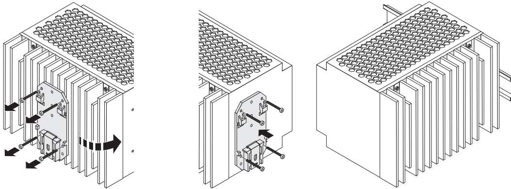
Bild 6 Schmale Einbaulage
