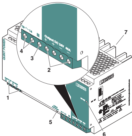
Bild 1 Bedienelemente
