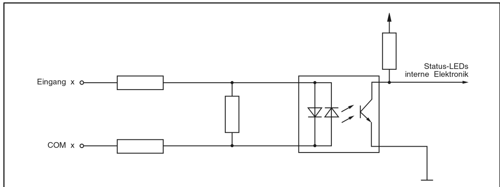
Abbildung 93: DI475 / DI476 Eingangsschema
