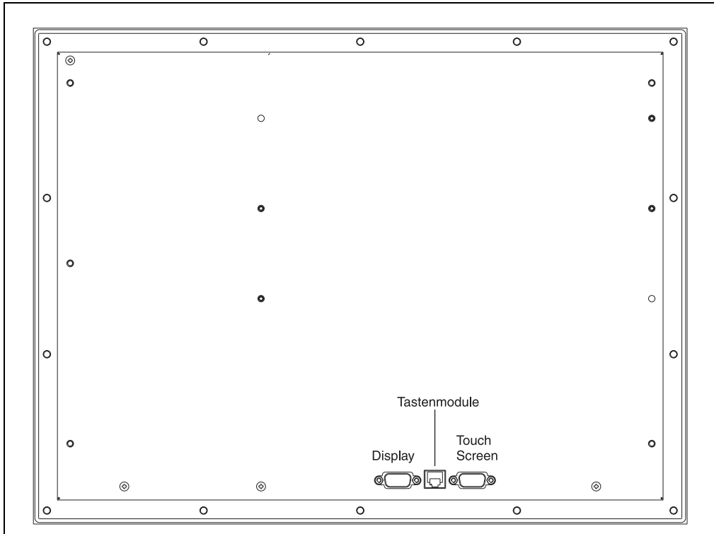
Abbildung 148: Anschlüsse 5D5212.02 Rev. >= 10
