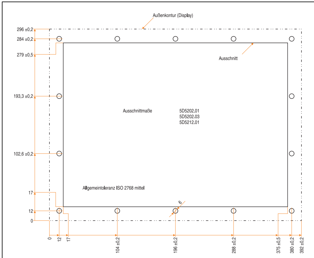
Abbildung 142: Einbau in Wanddurchbrüche 5D5202.01, 5D5202.03 und 5D5212.01
