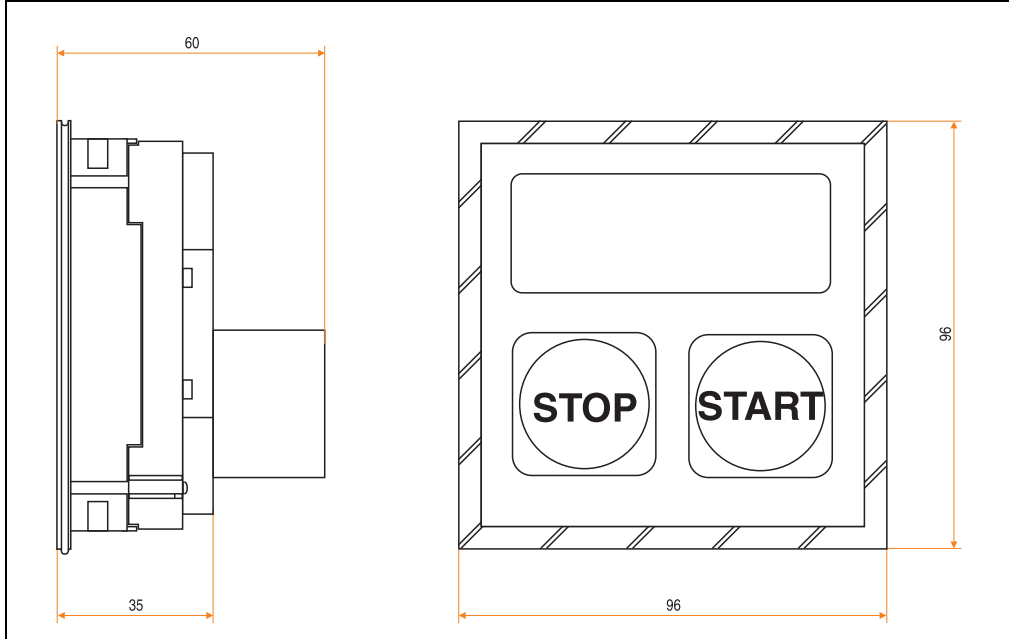
Abbildung 198: Abmessungen Tastenmodul mit Start/Stop-Schalter
