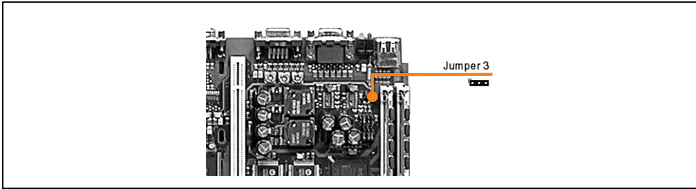
Abbildung 60: Lage des Jumpers für DRAM-Betriebsspannung
