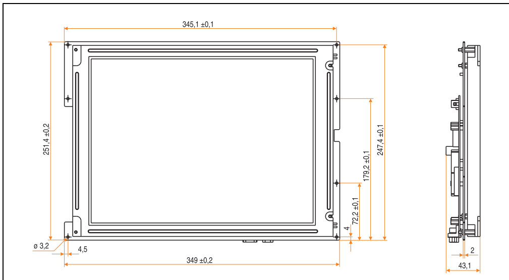
Abbildung 185: Abmessungen 5D5000.18
