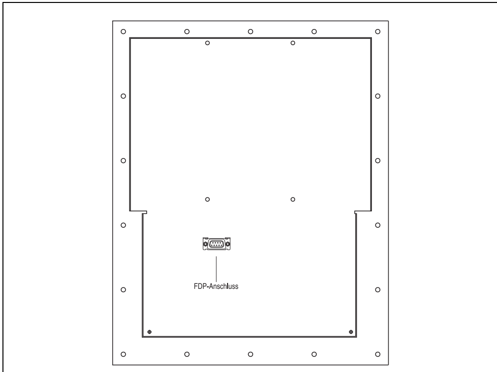
Abbildung 169: Anschlüsse 5D55xx.xx
