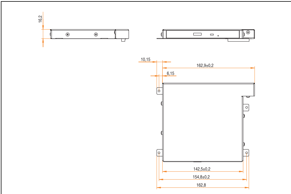
Abbildung 33: Abmessungen Add-On CD RW 5A5009.02
