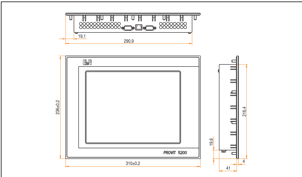
Abbildung 115: Abmessungen 5D5200.01 und 5D5210.01
