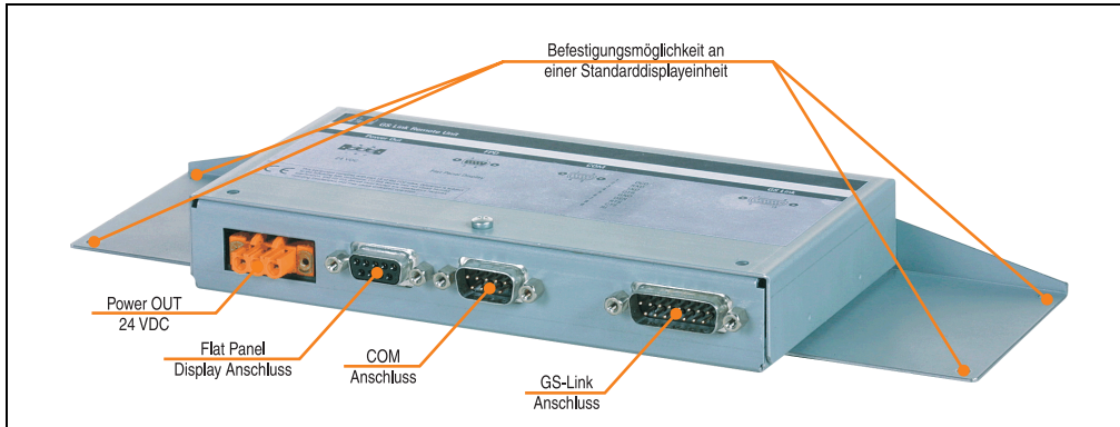
Abbildung 38: GS Link Remote Unit 5A5010.02 Komponenten
