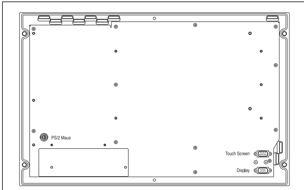
Abbildung 175: Anschlüsse 5D5600.0x und 5D5601.0x
