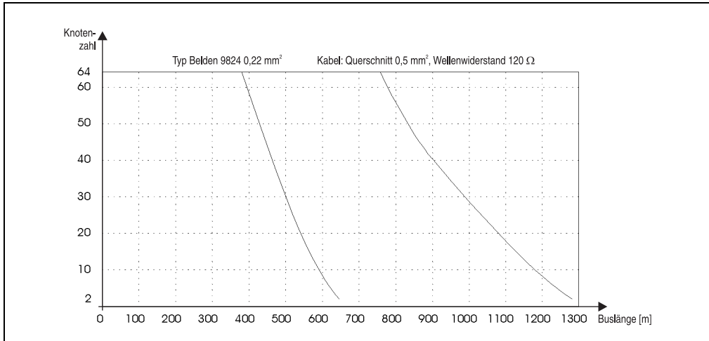
Abbildung 67: CAN Zusammenhang Knotenzahl und Buslänge
