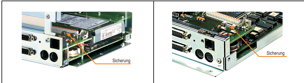
Abbildung 62: Sicherungsposition IPC5000 (links) und IPC5600 (rechts)
