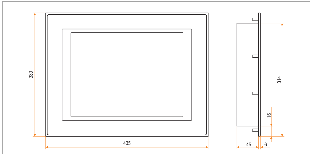
Abbildung 146: Abmessungen 5D5212.02 Rev. < I0
