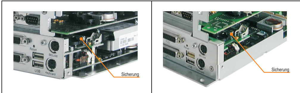
Abbildung 72: Sicherungsposition IPC500C (links) und IPC5600C (rechts)
