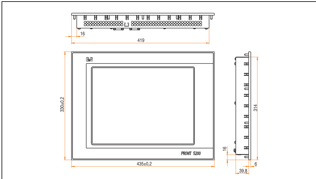
Abbildung 145: Abmessungen 5D5212.02 Rev. >= I0
