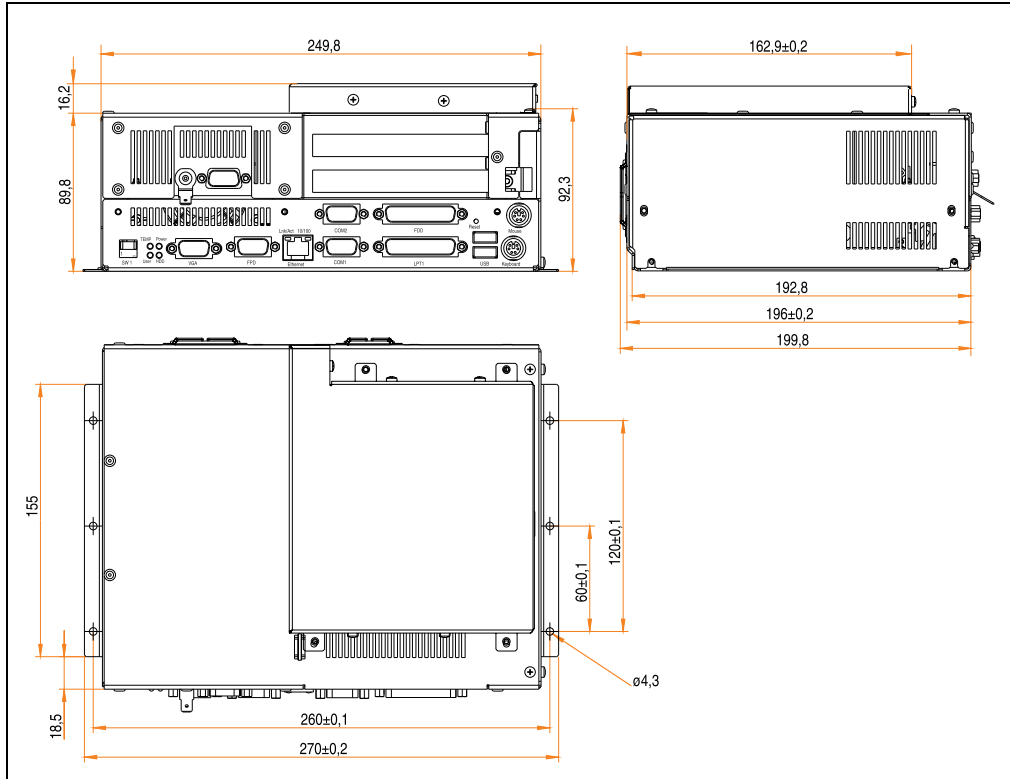
Abbildung 7: Abmessungen IPC5000C (2-Slot-Ausführung mit Add-On-Laufwerk 5A5009.0x)
