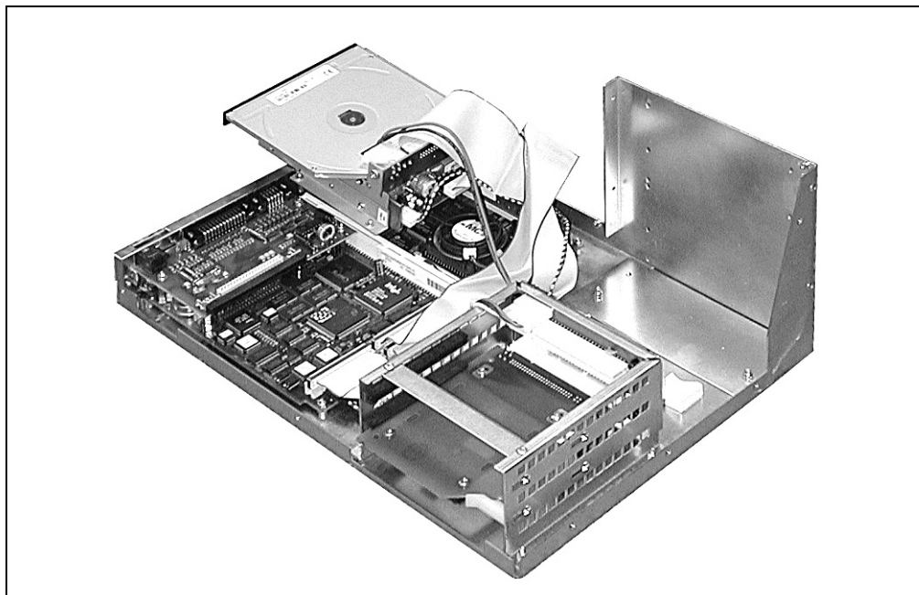
Abbildung 53: Abtrennen der Laufwerke
