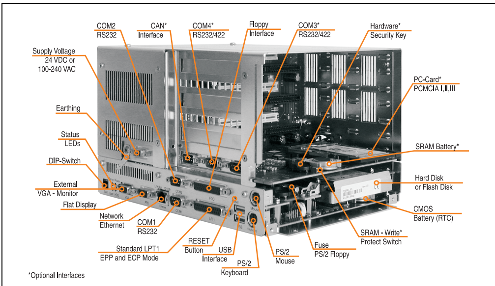
Abbildung 25: Komponenten des IPC5000C (Buseinheit mit 4 Steckplätzen)
