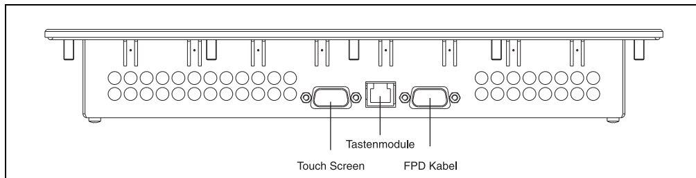
Abbildung 128: Anschlüsse 5D5211.02 Rev. >= F0
