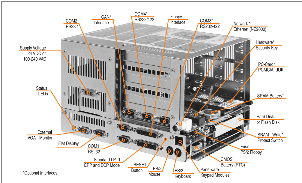
Abbildung 20: Komponenten des IPC5000 (Buseinheit mit 4 Steckplätzen)
