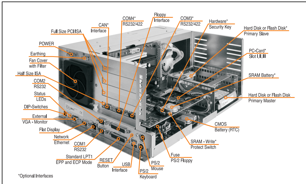
Abbildung 27: Komponenten des IPC5600C (Buseinheit mit 4 Steckplätzen)
