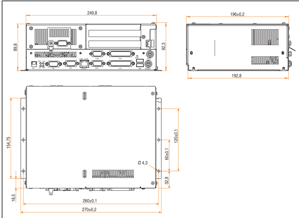
Abbildung 5: IPC5000C (2-Slot-Ausführung)
