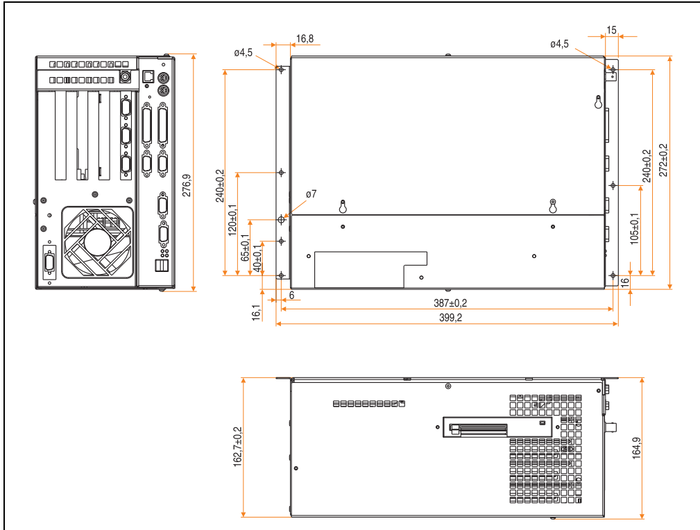
Abbildung 12: Abmessungen IPC5600 (4-Slot-Ausführung)
