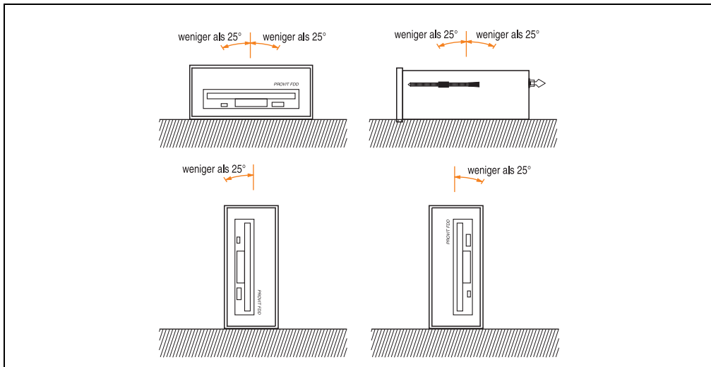
Abbildung 9: Montagevorschriften Externes 3,5“ Diskettenlaufwerk
