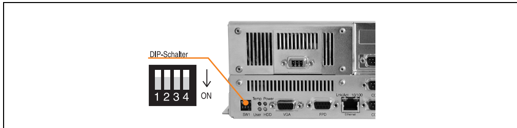
Abbildung 77: DIP-Schalter IPC5000C und IPC5600C
