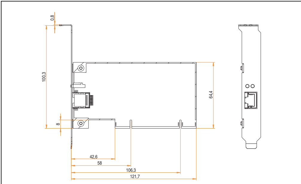
Abbildung 48: Abmessungen - 5ACPCI.ETH1-01
