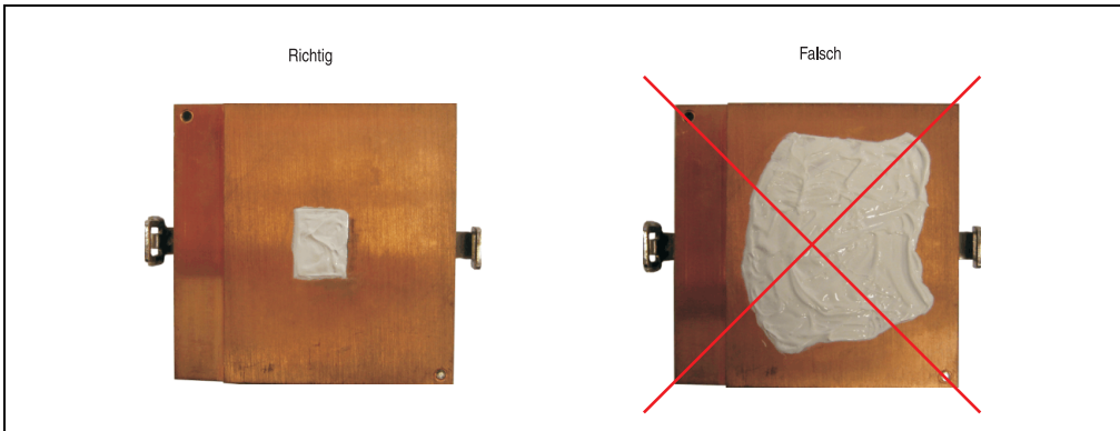
Abbildung 76: Wärmeleitpaste auftragen
