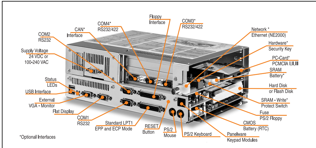
Abbildung 19: Komponenten des IPC5000 (Buseinheit mit 2 Steckplätzen)
