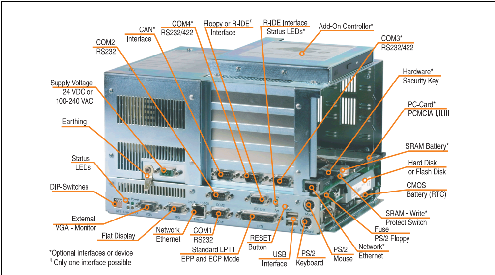
Abbildung 26: Komponenten des IPC5000C (Buseinheit mit 5 Steckplätzen + Add-On Controller)
