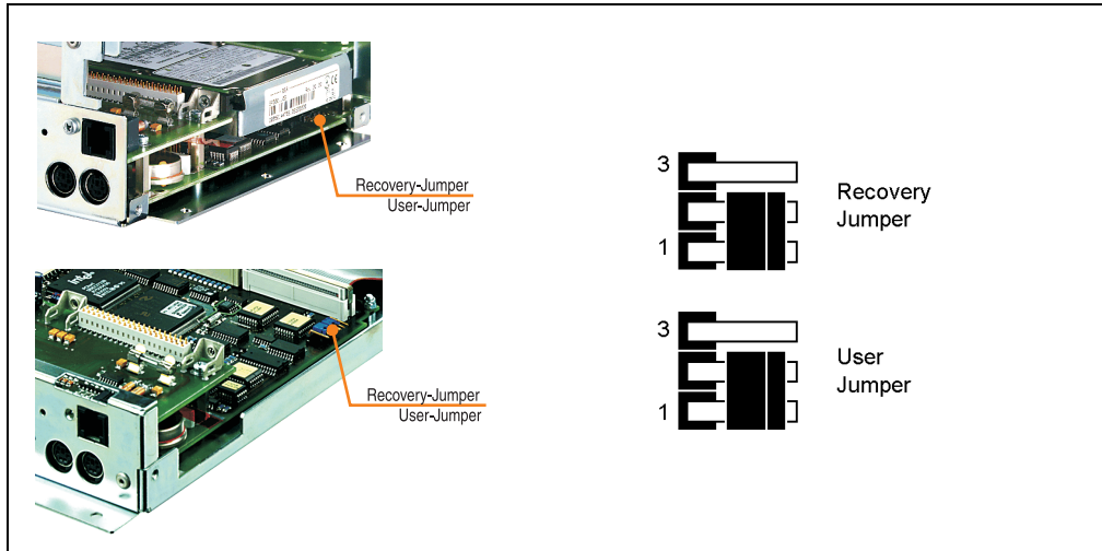
Abbildung 66: Recovery-Jumper / User-Jumper IPC5000 (oben) und IPC5600 (unten)
