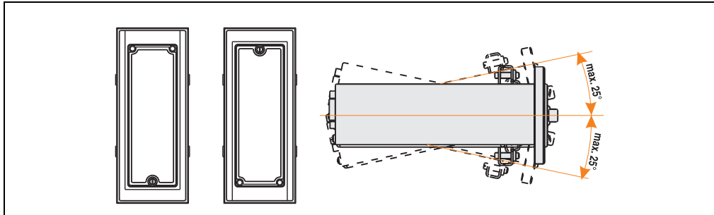
Abbildung 13: Montagevorschriften Controller R-IDE CD-ROM / LS120 Laufwerk (senkrecht / waagrecht)
