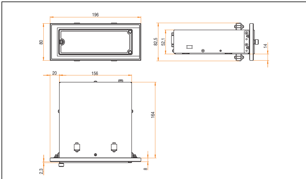
Abbildung 21: Abmessungen 5A5003.08 mit 5A5003.03
