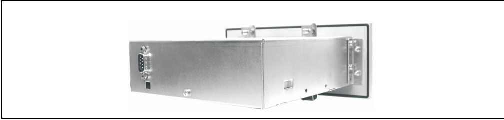
Abbildung 18: Montageart mit Frontplatte
