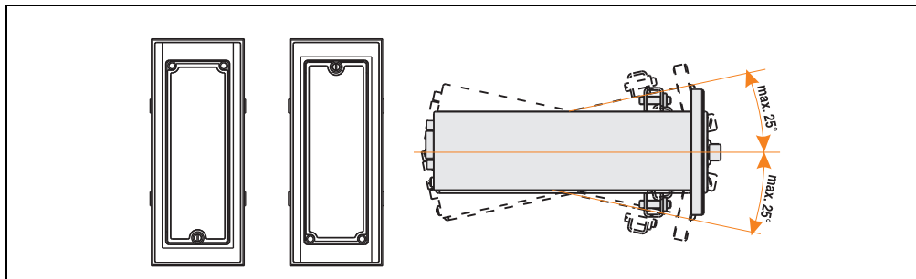
Abbildung 17: Montagevorschriften Controller R-IDE CD-ROM / LS120 Laufwerk (senkrecht / waagrecht)
