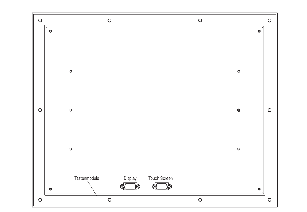
Abbildung 149: Anschlüsse 5D5212.02 Rev. < I0
