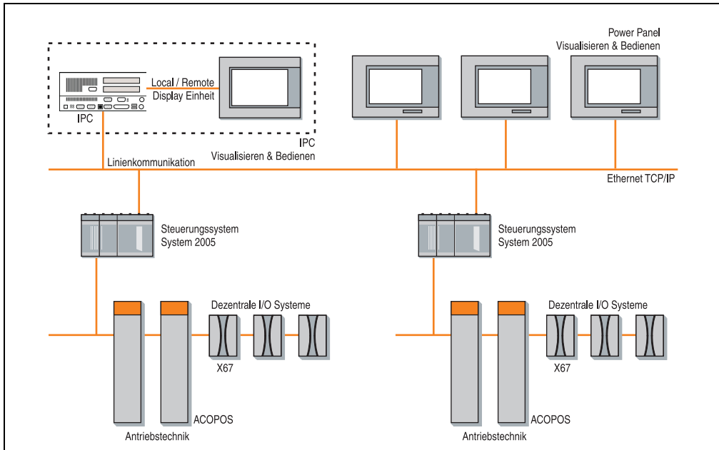
Abbildung 2: Industrie PC als klassisches Visualisierungsgerät
