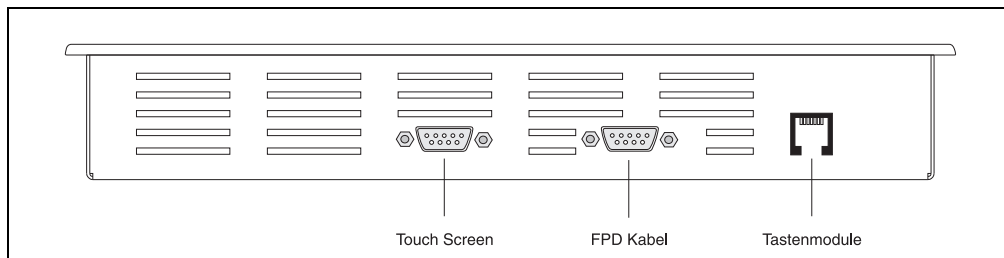
Abbildung 127: Anschlüsse 5D5201.02 und 5D5211.02
