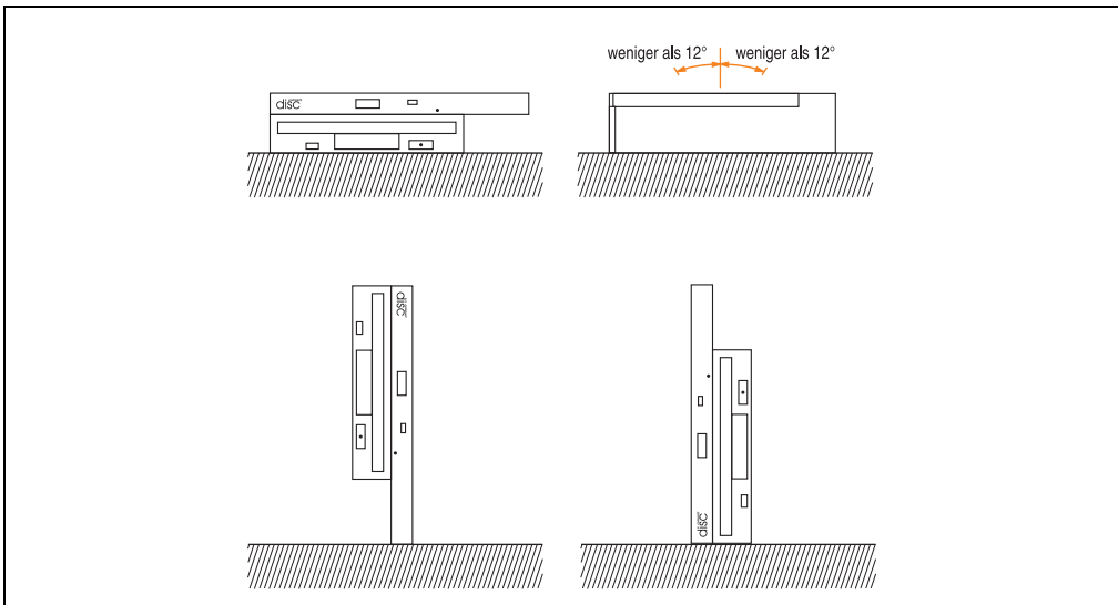
Abbildung 39: Montagevorschriften 5A5600.04
