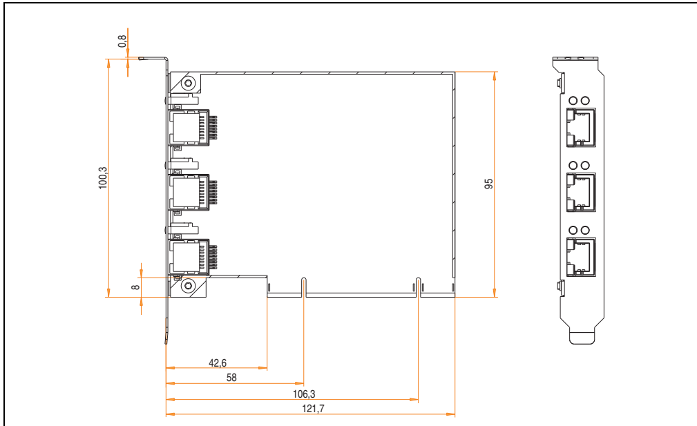
Abbildung 50: Abmessungen - 5ACPCI.ETH3-01
