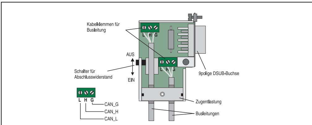
Abbildung 105: CAN-Busstecker 7AC911.9
