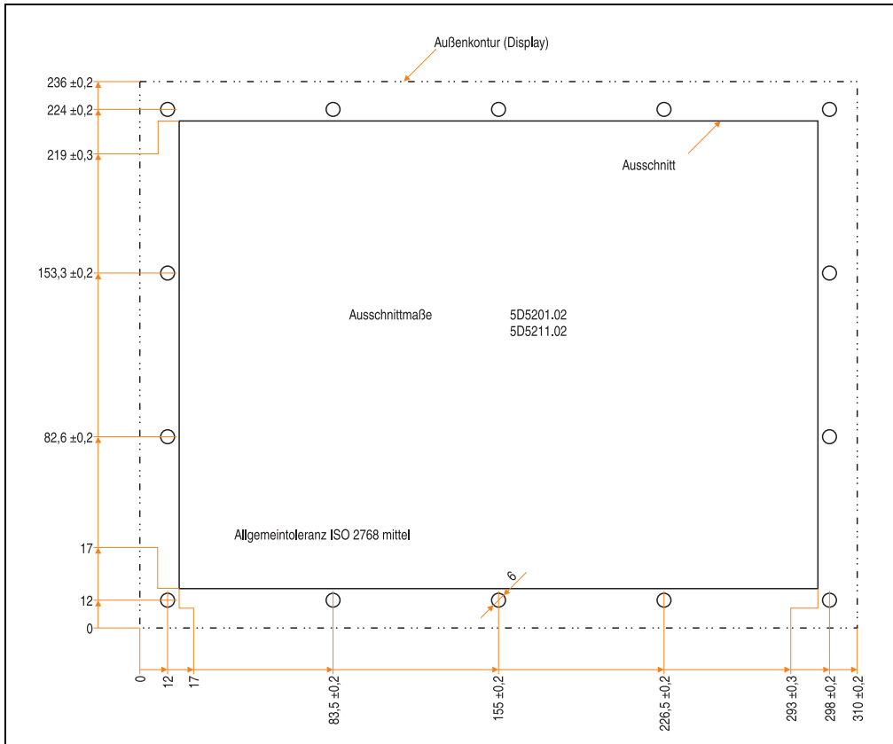
Abbildung 126: Einbau in Wanddurchbrüche 5D5201.02 und 5D5211.02
