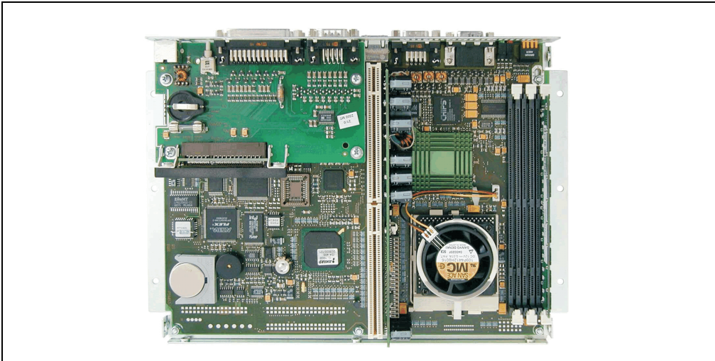
Abbildung 70: Mainboard Systemeinheiten mit Socket 370
