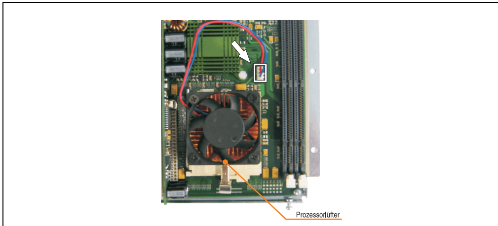
Abbildung 73: Stecker lösen
