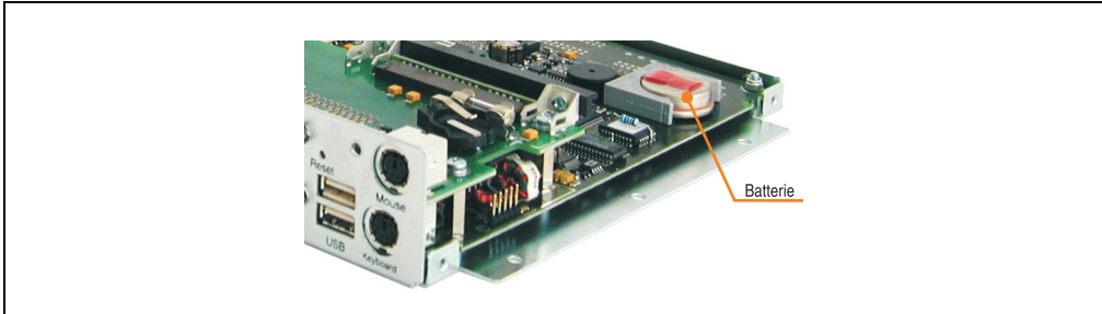
Abbildung 75: Batteriehalter IPC5000C und IPC5600C
