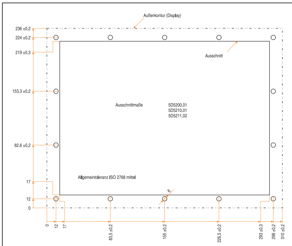
Abbildung 116: Einbau in Wanddurchbrüche 5D5200.01 und 5D5210.01
