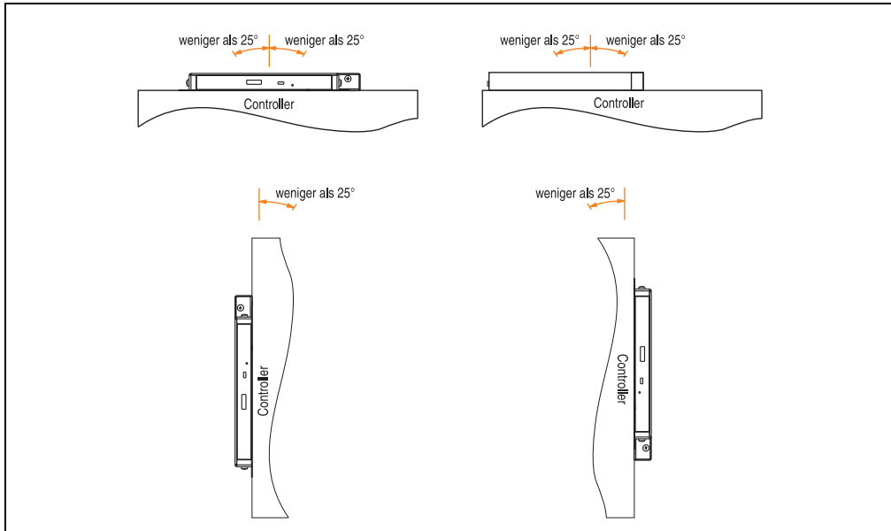
Abbildung 29: Montagevorschriften Add-On CD-ROM mit Controller
