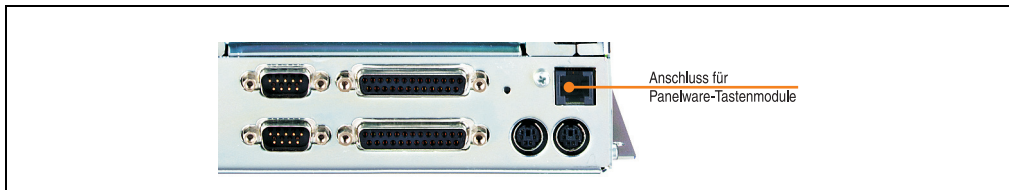
Abbildung 68: Anschluss von Panelware Tastenmodulen
