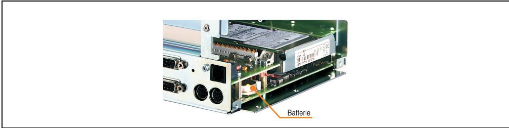
Abbildung 64: Batteriehalterung
