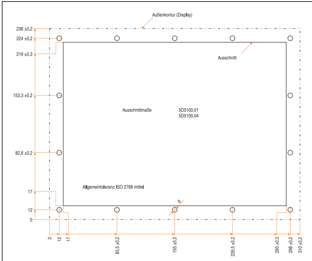
Abbildung 112: Einbau in Wanddurchbrüche 5D5100.01 und 5D5100.04
