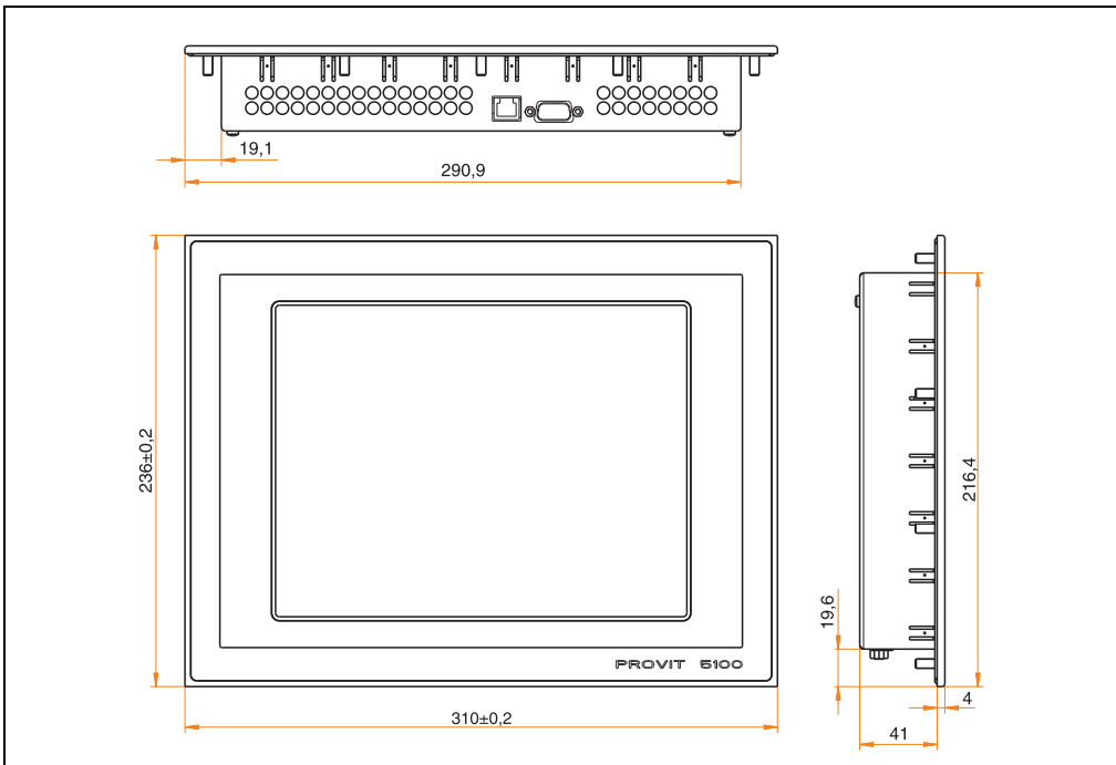
Abbildung 111: Abmessungen 5D5100.01 und 5D5100.04
