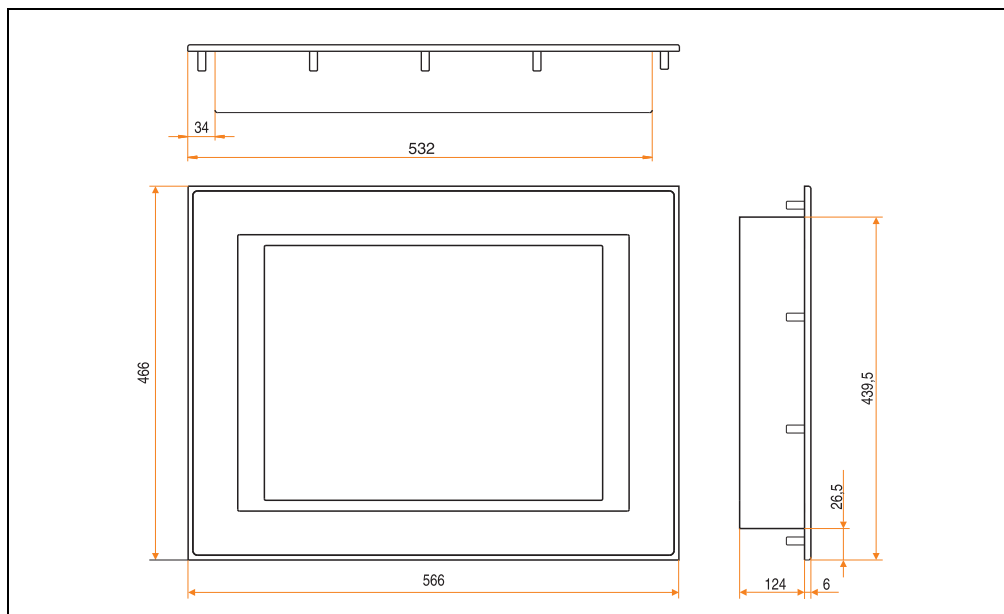
Abbildung 162: Abmessungen 5D9200.01
