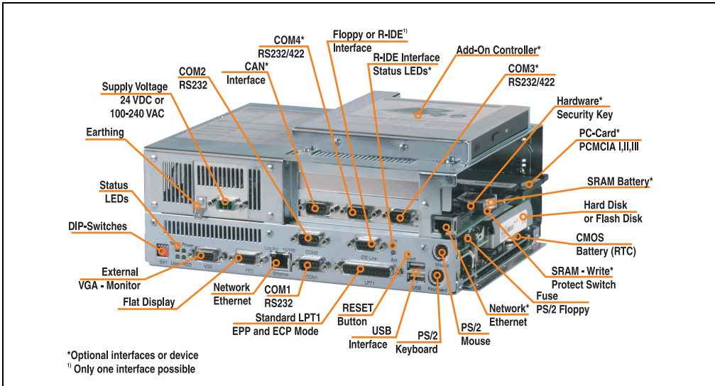
Abbildung 24: Komponenten des IPC5000C (Buseinheit mit 2 Steckplätzen + Add-On Controller)
