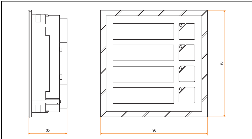
Abbildung 194: Abmessungen Tastenmodul mit 4 Tasten
