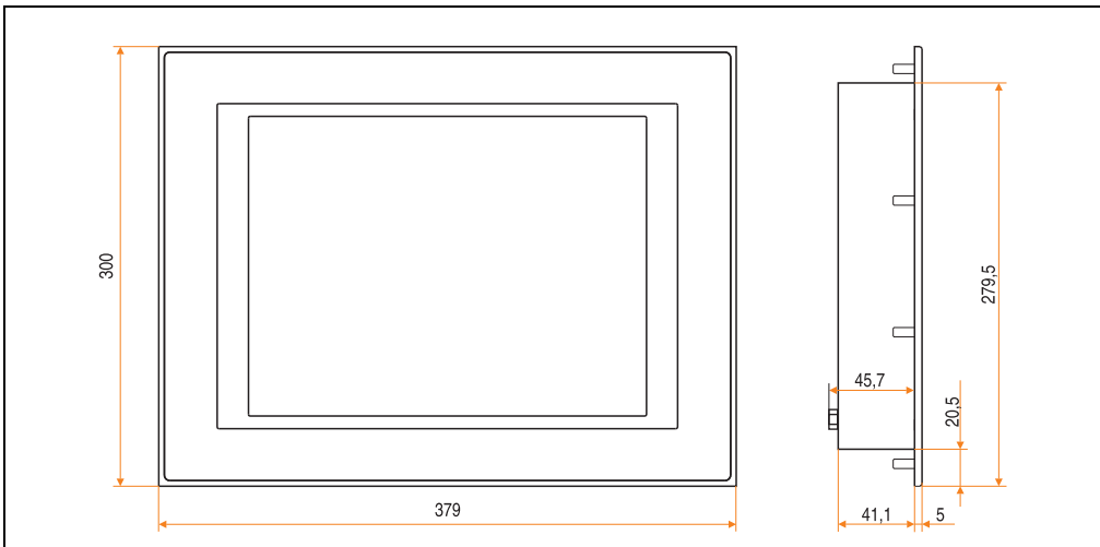
Abbildung 130: Abmessungen 5D5201.03 und 5D5211.03
