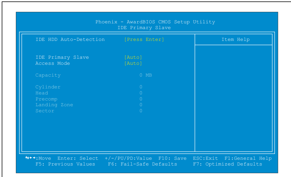
Abbildung 211: IDE Primary Slave Setup
