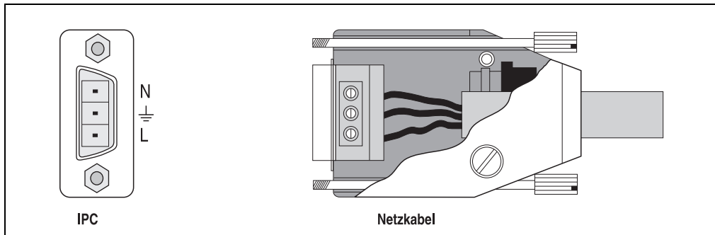
Abbildung 86: Stecker und Buchse (3-polig) für AC-Versorgung
