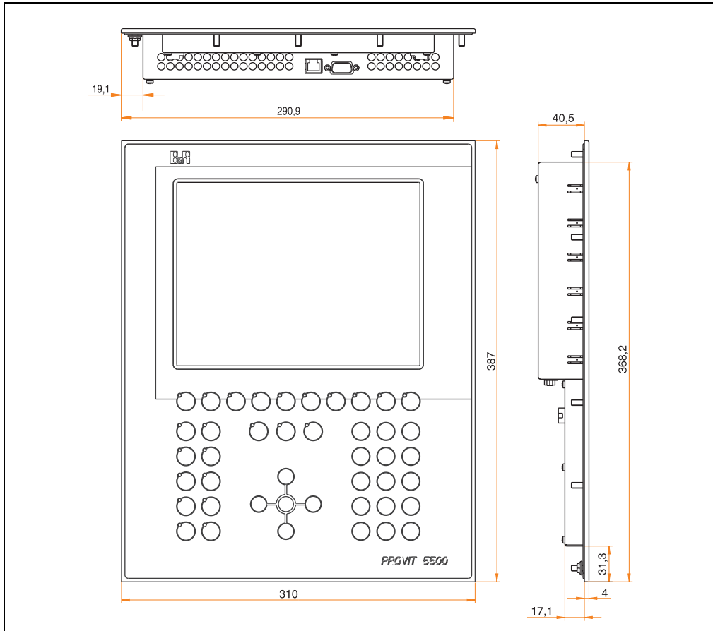
Abbildung 167: Abmessungen 5D5510 ab Rev. F0
