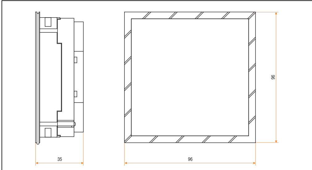
Abbildung 195: Abmessungen Blindmodul
