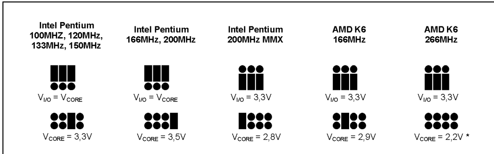
Abbildung 59: Einstellen der Versorgungsspannung des Prozessors (Jumper 2)
