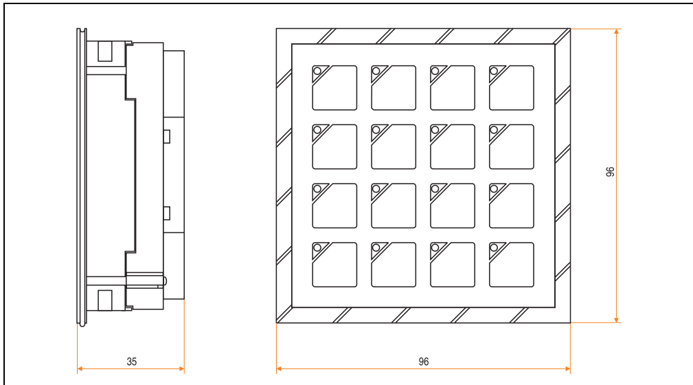
Abbildung 191: Abmessungen Tastenmodul mit 16 Tasten
