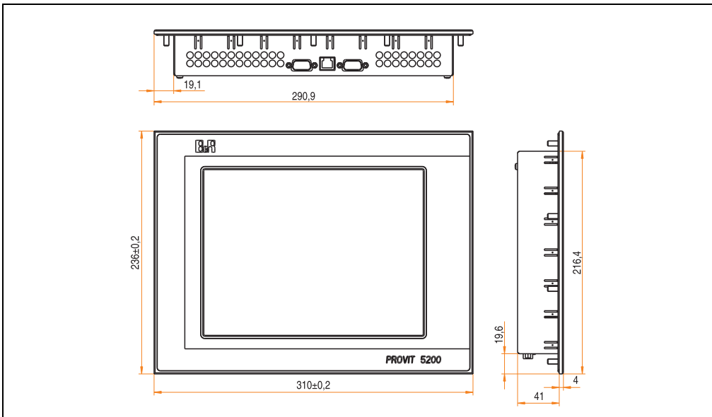
Abbildung 124: Abmessungen 5D5201.02 und 5D5211.02
