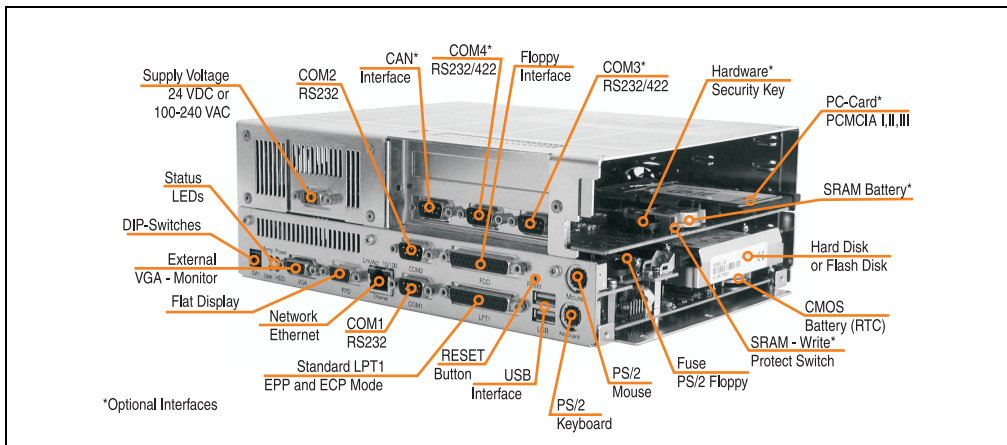
Abbildung 23: Komponenten des IPC5000C (Buseinheit mit 2 Steckplätzen)
