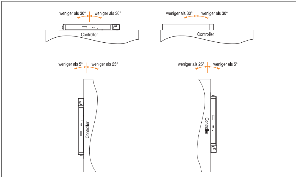
Abbildung 34: Montagevorschriften Add-On CD RW ab Rev. D0 mit Controller
