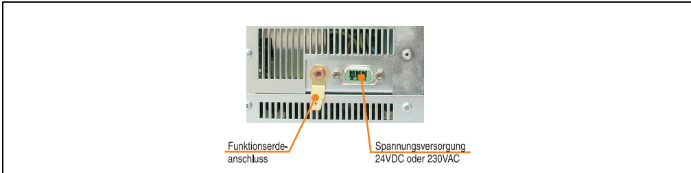
Abbildung 87: Funktionserdeanschluss IPC5000 und IPC5000C (2, 4 und 5 Slot Ausführung)
