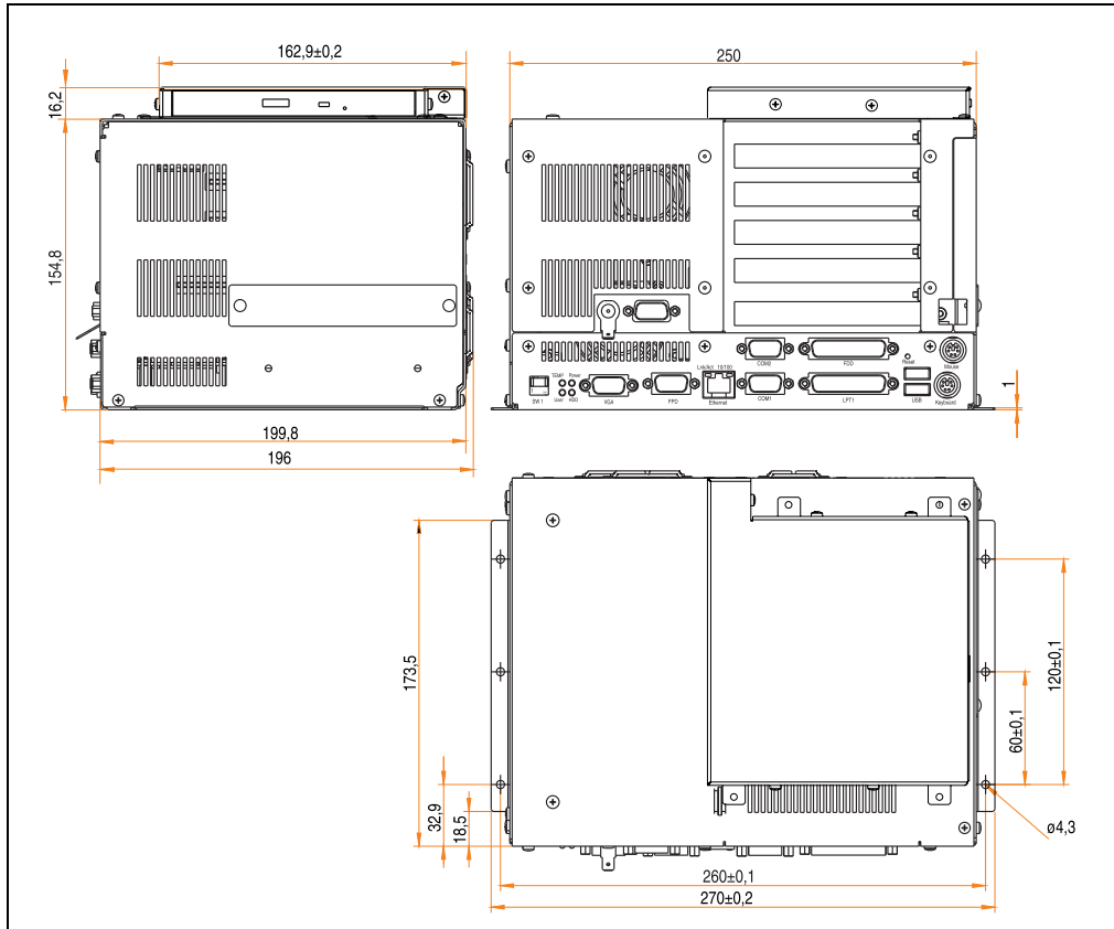
Abbildung 11: Abmessungen IPC5000C (5-Slot-Ausführung + Add-On-Laufwerk 5A5009.0x)
