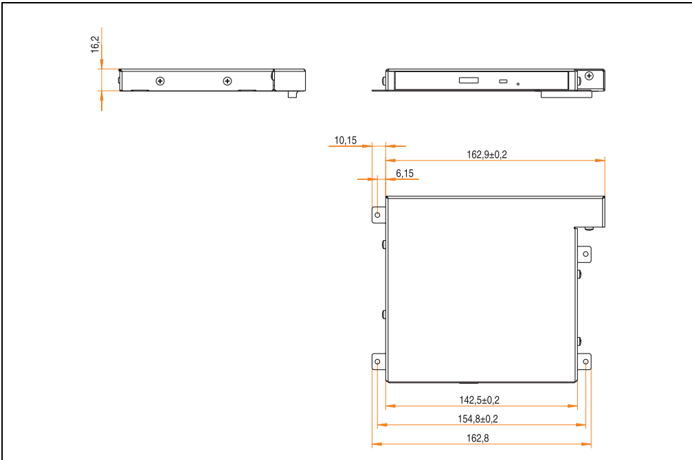
Abbildung 28: Abmessungen Add-On CD ROM 5A5009.01
