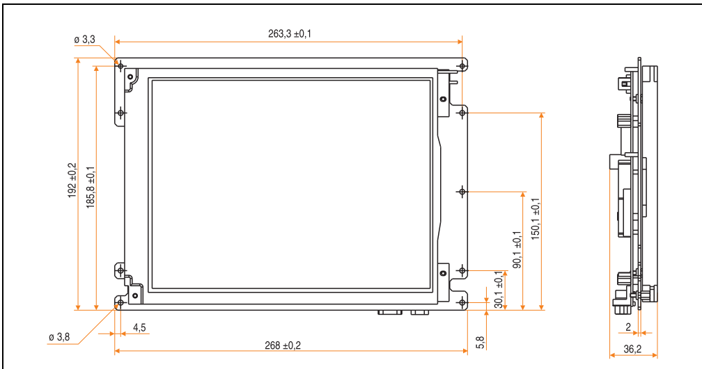
Abbildung 179: Abmessungen 5D5000.03
