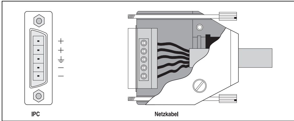
Abbildung 85: Stecker und Buchse (5-polig) für DC-Versorgung
