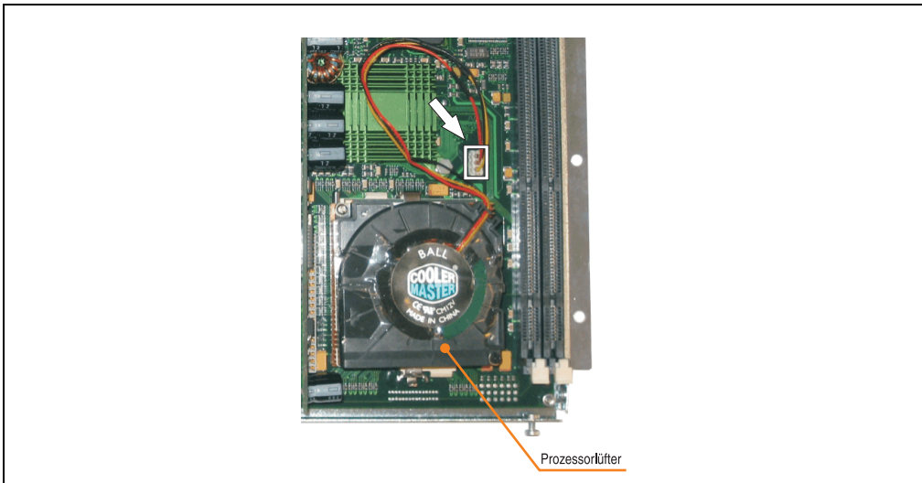
Abbildung 78: Stecker anstecken
