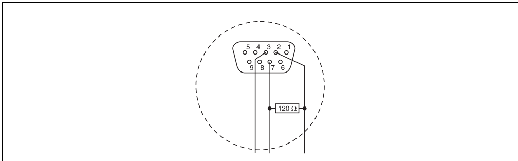
Abbildung 104: Beschaltung des Abschlusswiderstandes für 9poligen DSUB-Stecker
