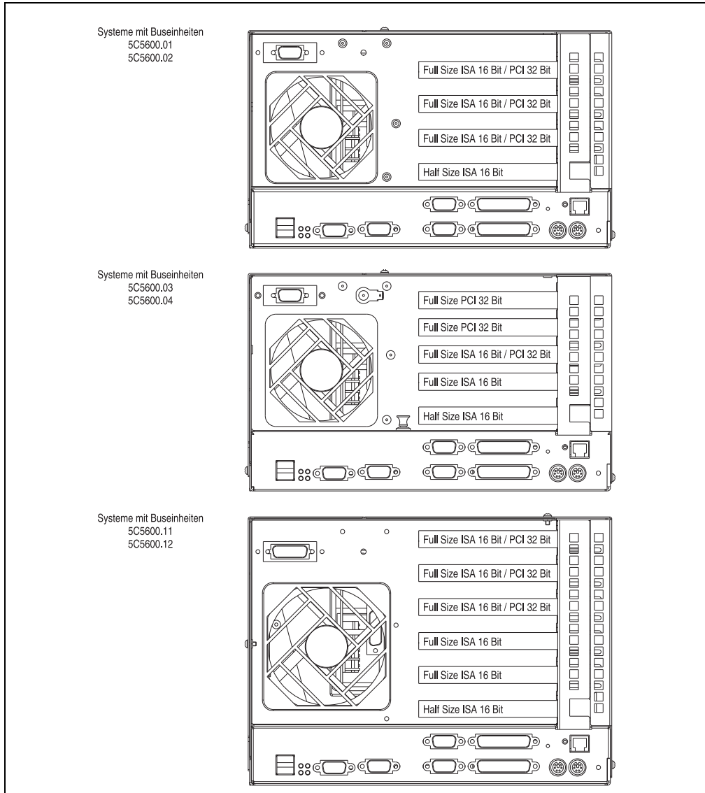
Abbildung 83: Steckplatzbelegung Provit 5600 Einheiten
