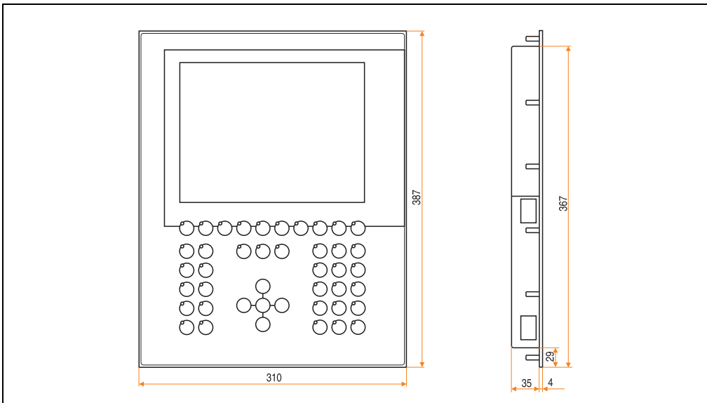
Abbildung 166: Abmessungen 5D55xx.xx
