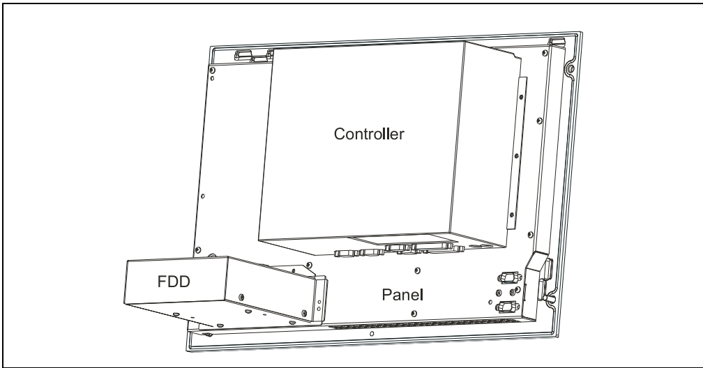
Abbildung 36: Montagebeispiel FDD 5A5600.03 mit Controller auf einem Panel
