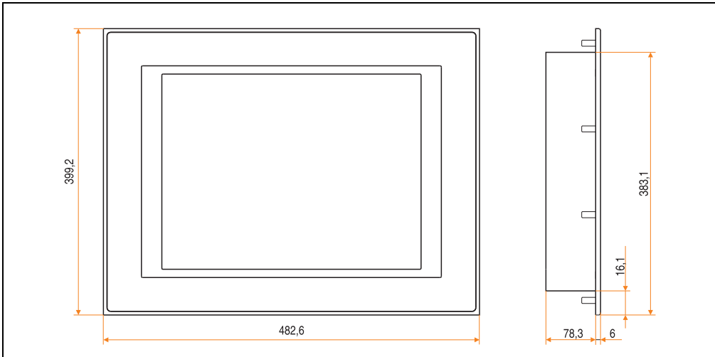
Abbildung 157: Abmessungen 5D5213.01
