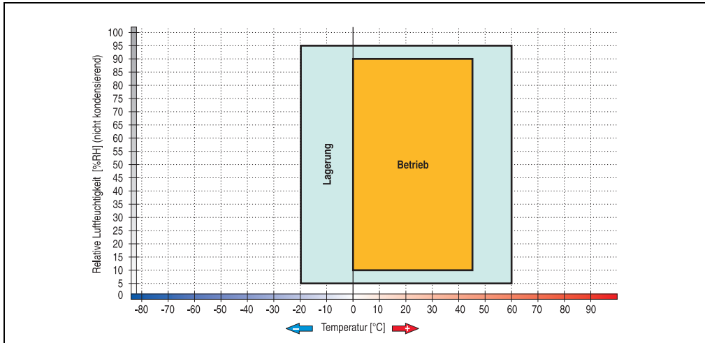
Abbildung 45: Temperatur Luftfeuchtediagramm USB Memory Sticks - 5MMUSB.xxxx-00
