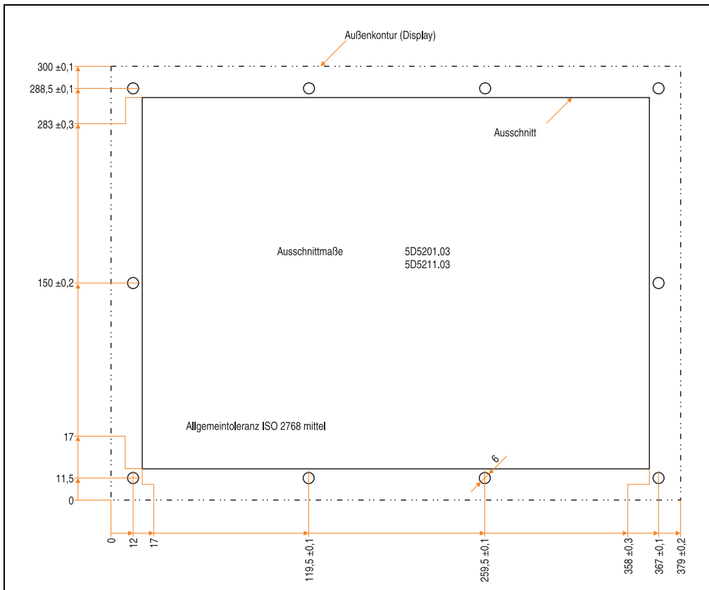
Abbildung 133: Einbau in Wanddurchbrüche 5D5201.03 und 5D5211.03
