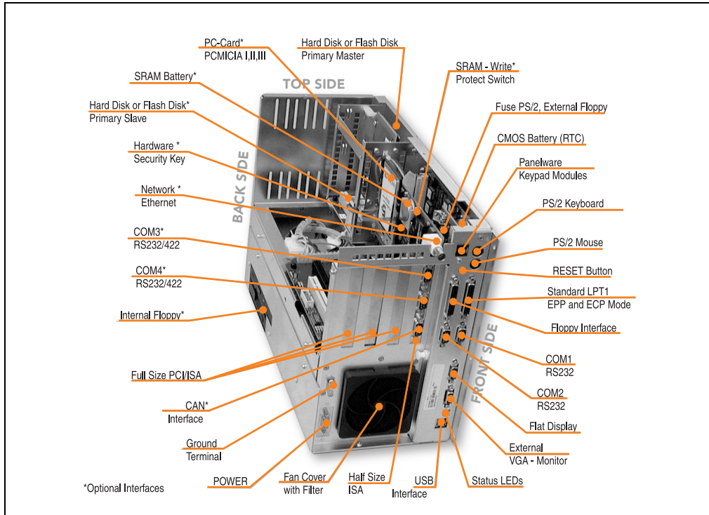
Abbildung 21: Komponenten des IPC5600 (Buseinheit mit 4 Steckplätzen)
