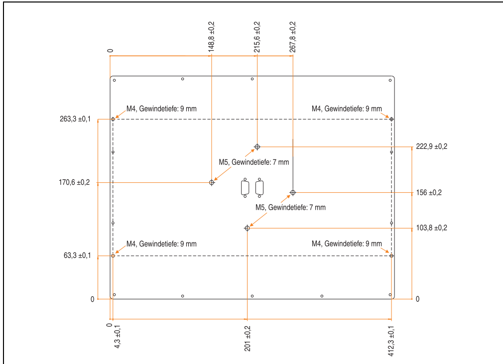
Abbildung 154: Flanschbohrungen für 5D5212.04 ab Rev. G0
