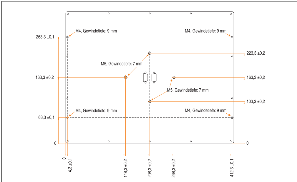
Abbildung 153: Flanschbohrungen für 5D5212.04 ab Rev. J0
