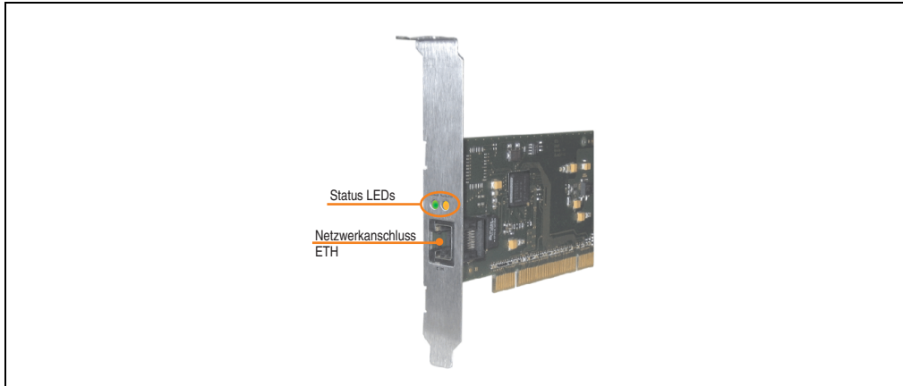
Abbildung 47: PCI Ethernet Card 10/100 - 5ACPCI.ETH1-01
