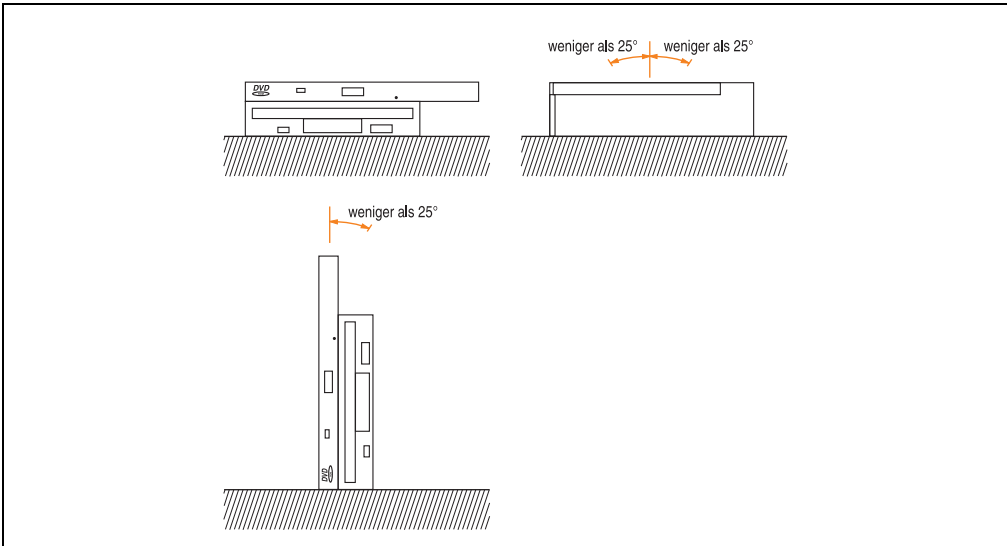
Abbildung 41: Montagevorschriften 5A5600.05
