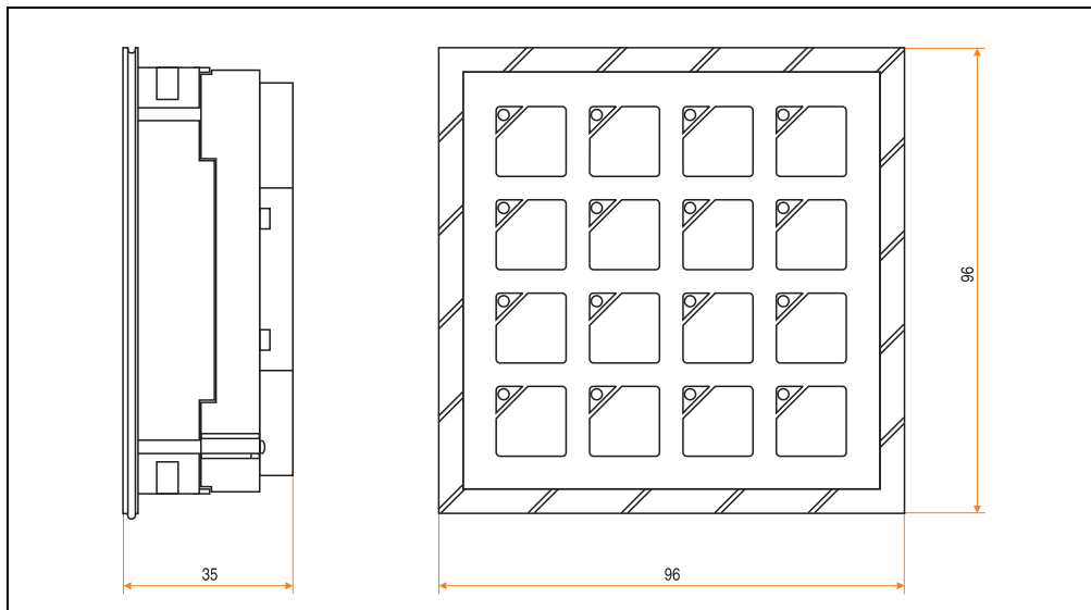
Abbildung 189: Abmessungen Standardtastenmodul
