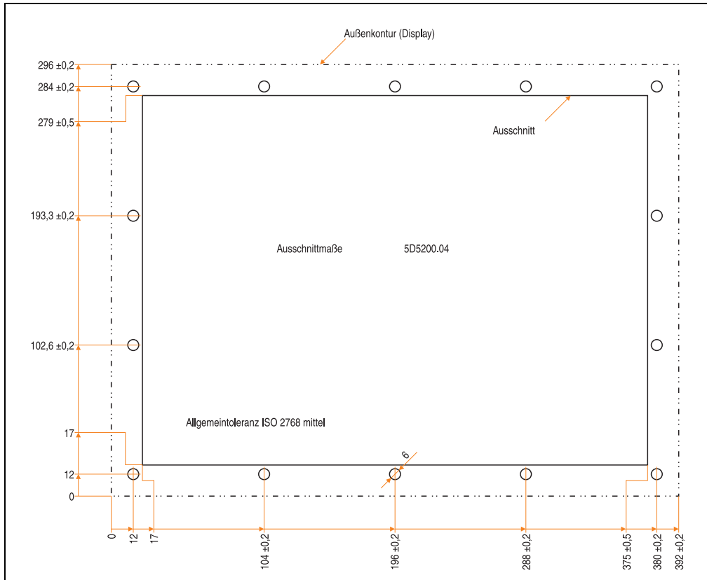
Abbildung 121: Einbau in Wanddurchbrüche 5D5200.04
