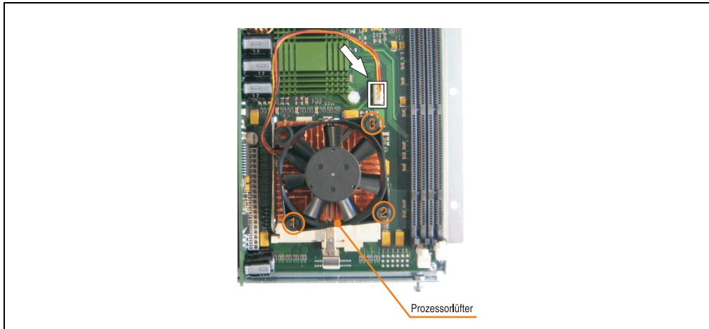
Abbildung 80: Lüfter befestigen und Stecker anstecken
