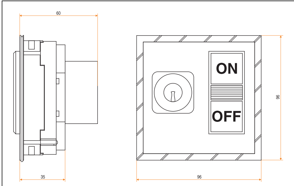
Abbildung 197: Abmessungen Tastenmodul mit Schlüsselschalter
