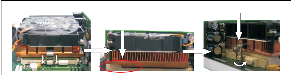
Abbildung 77: Neuen Kühlkörper anbringen
