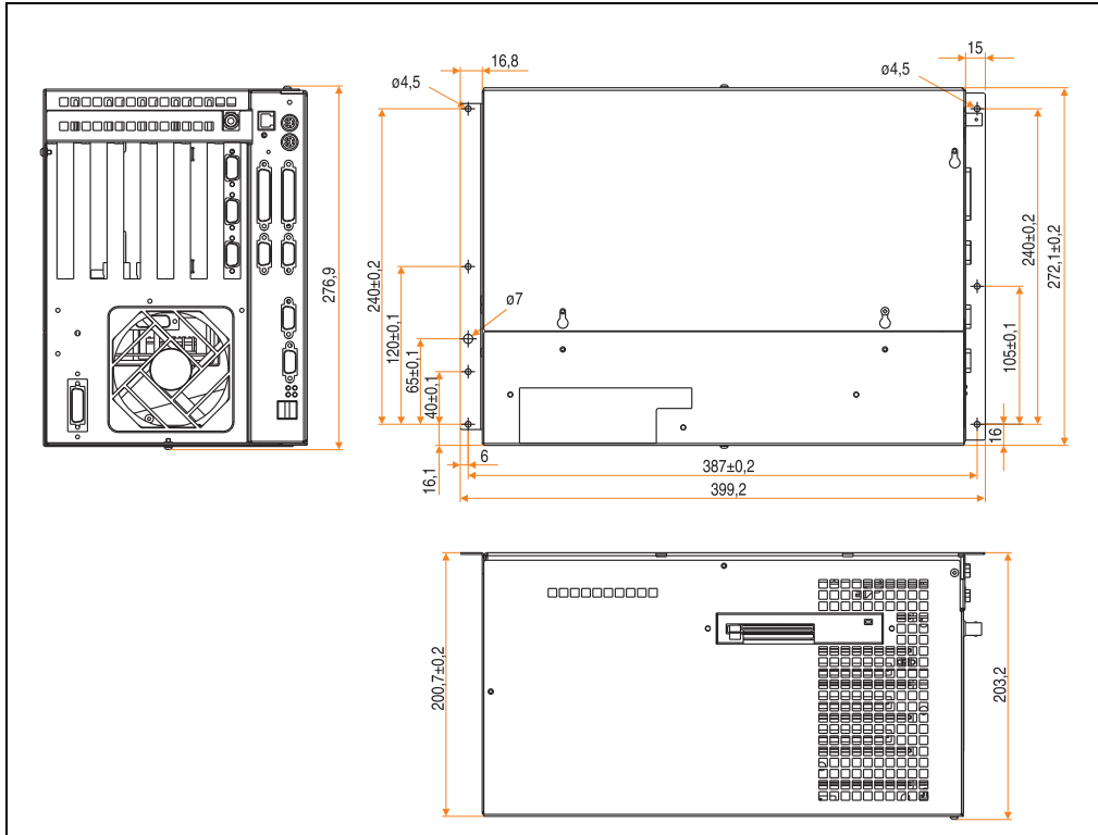
Abbildung 16: Abmessungen IPC5600 (6-Slot-Ausführung)
