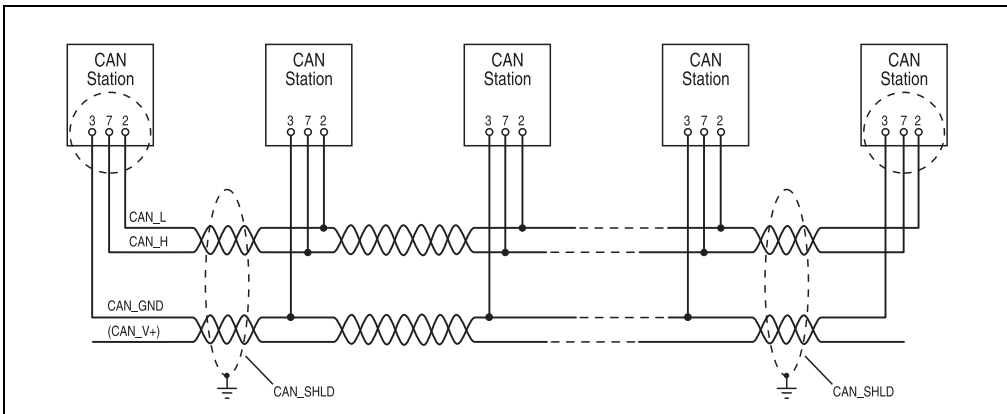
Abbildung 103: Verbindung Buskabel - Station
