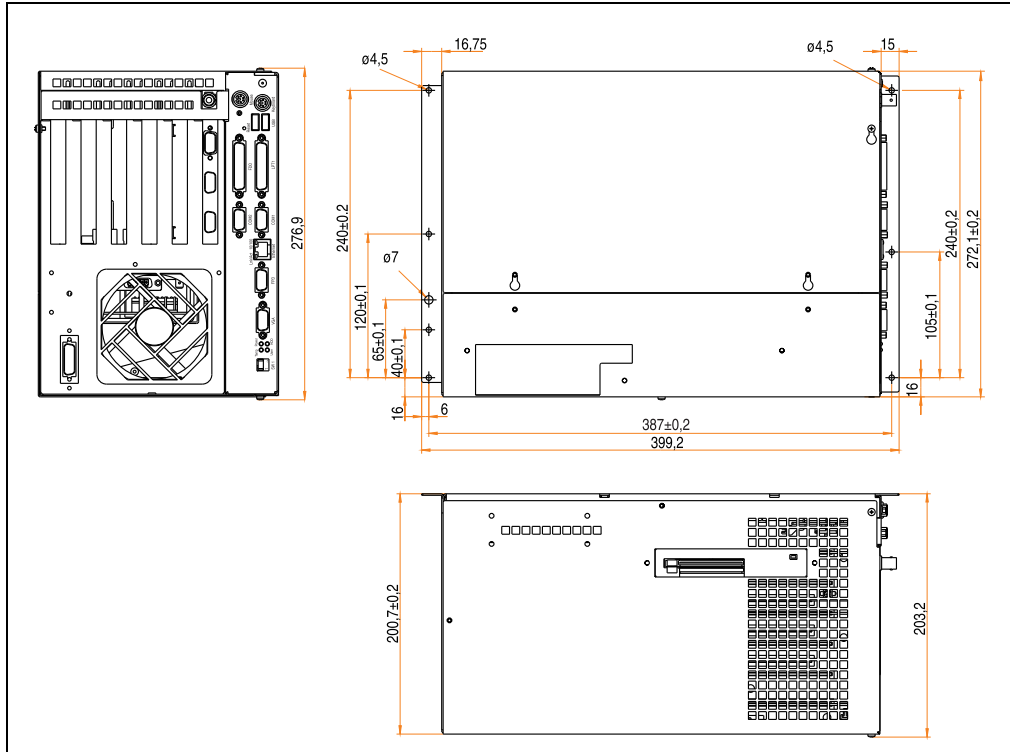
Abbildung 17: Abmessungen IPC5600C (6-Slot-Ausführung)
