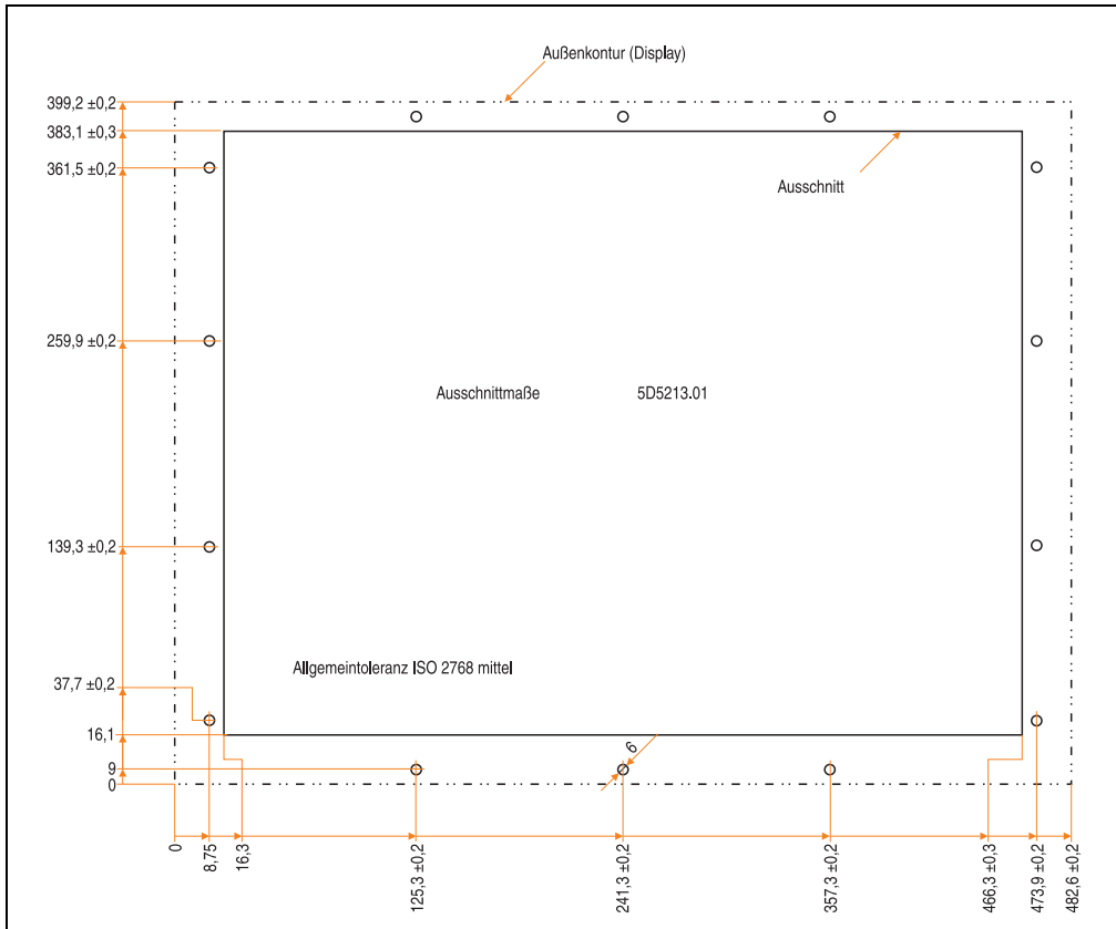
Abbildung 158: Einbau in Wanddurchbrüche 5D5213.01
