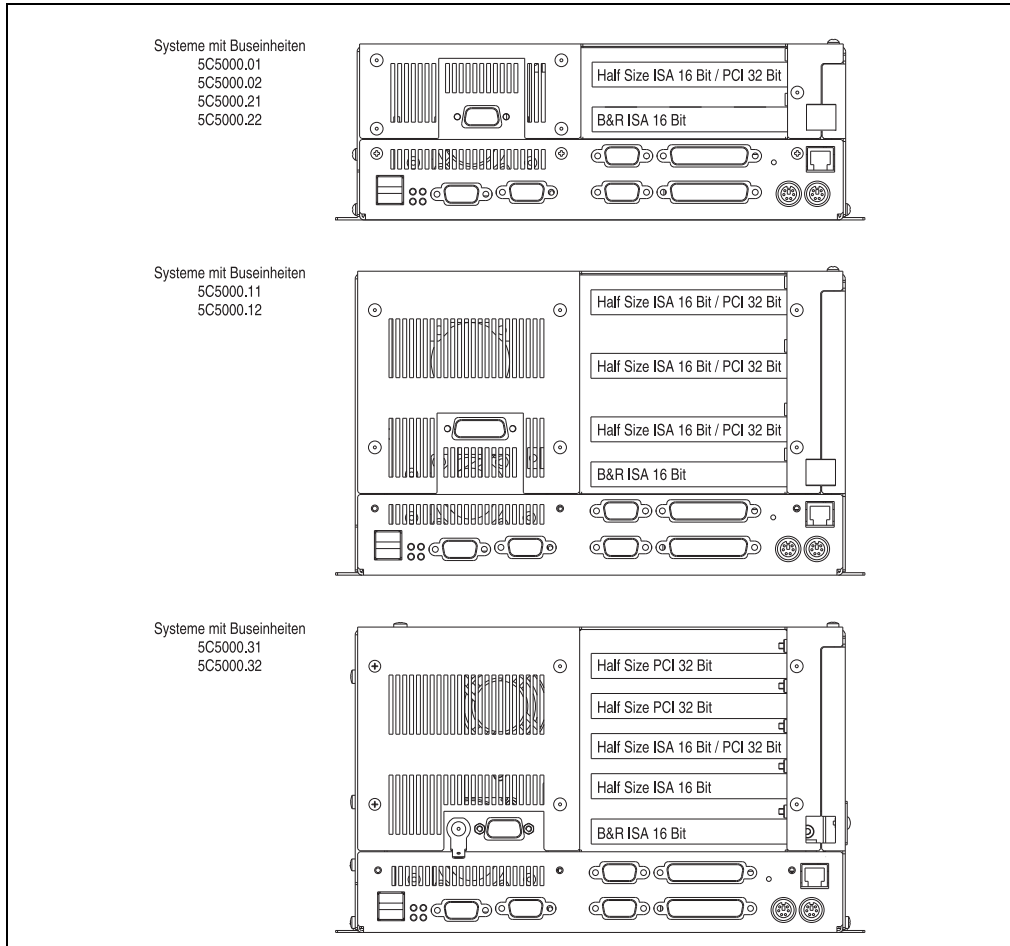
Abbildung 82: Steckplatzbelegung Provit 5000 Einheiten
