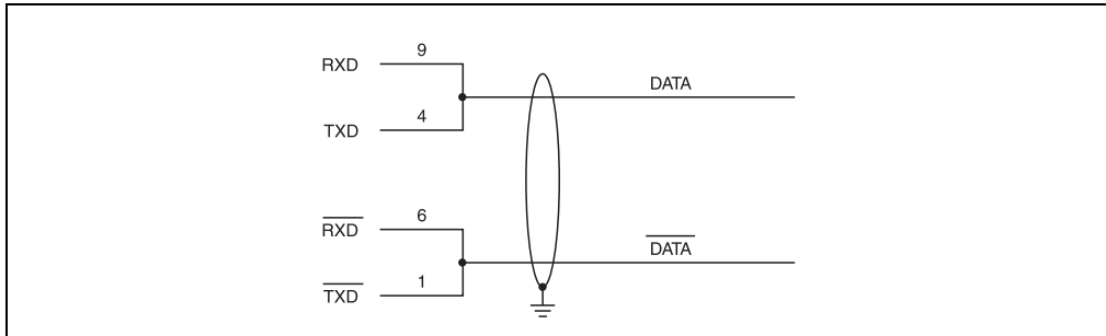
Abbildung 102: Betrieb der COM3 oder COM4 Schnittstelle im RS485 Modus
