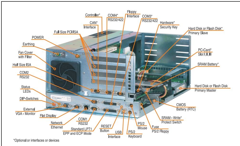
Abbildung 28: Komponenten des IPC5600C (Buseinheit mit 5 Steckplätzen)
