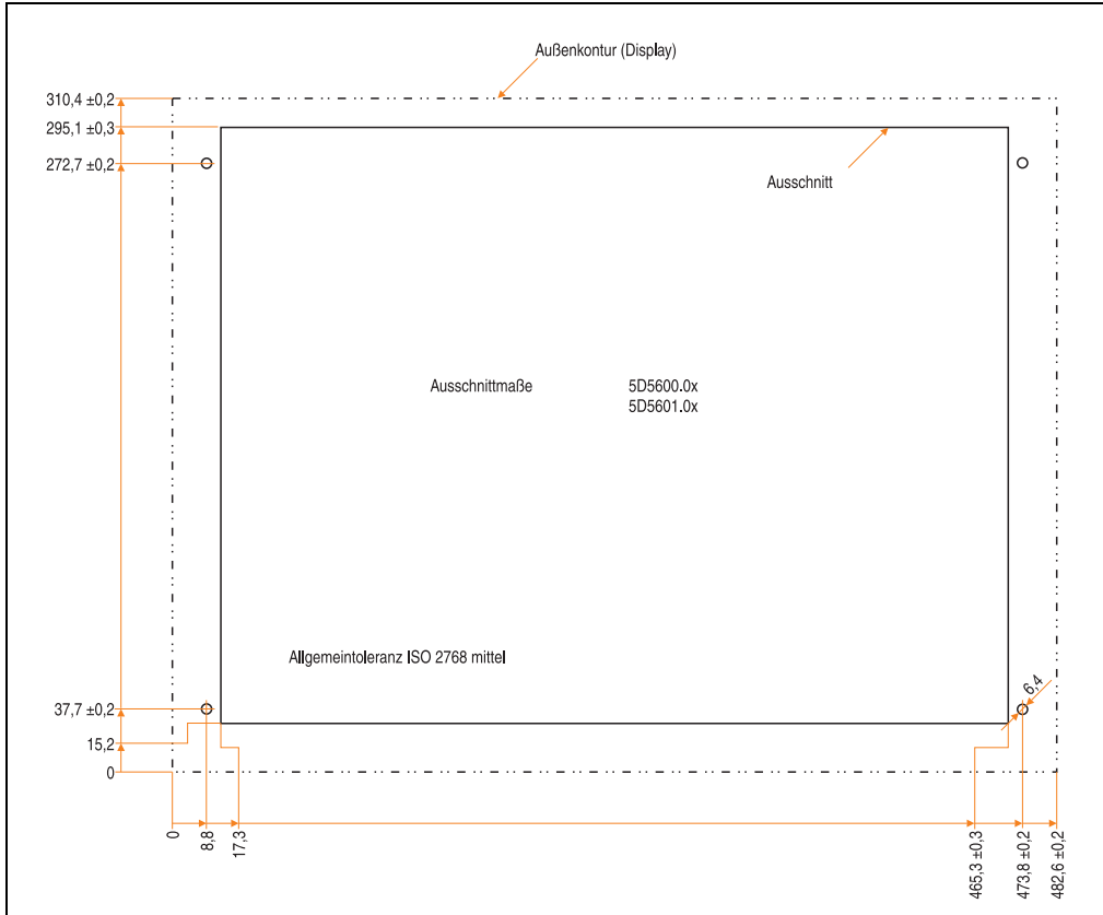
Abbildung 174: Einbau in Wanddurchbrüche 5D5600.0x und 5D5601.0x
