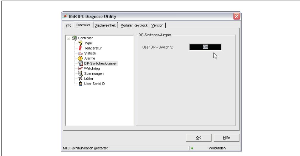
Abbildung 237: B&R IPC Diagnose Utility - Registerkarte Controller - DIP Switch
