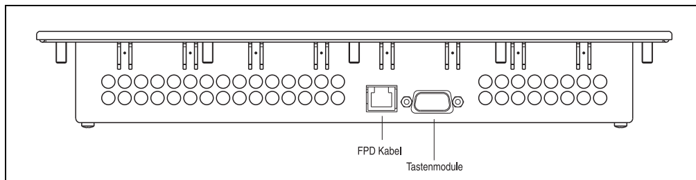
Abbildung 113: Anschlüsse 5D5100.01 und 5D5100.04
