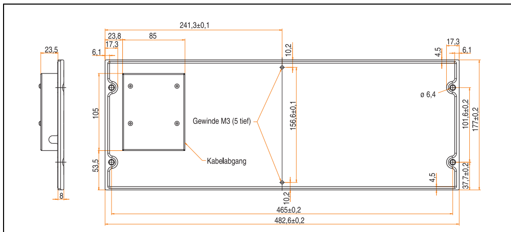
Abbildung 42: Einbaumaße 19" AT-Tastatur (Abbildung rückseitig)
