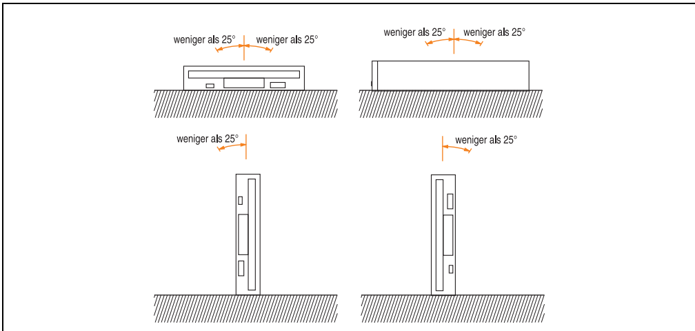
Abbildung 37: Montagevorschriften 5A5600.03
