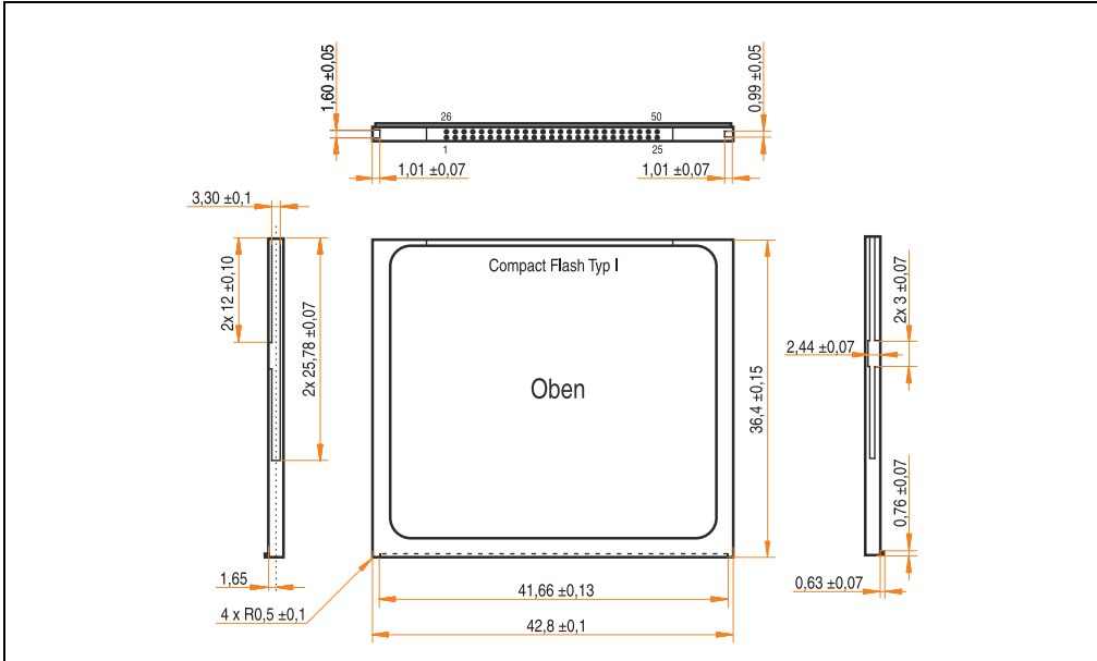
Abbildung 94: Abmessungen Compact Flash Karte Typ I
