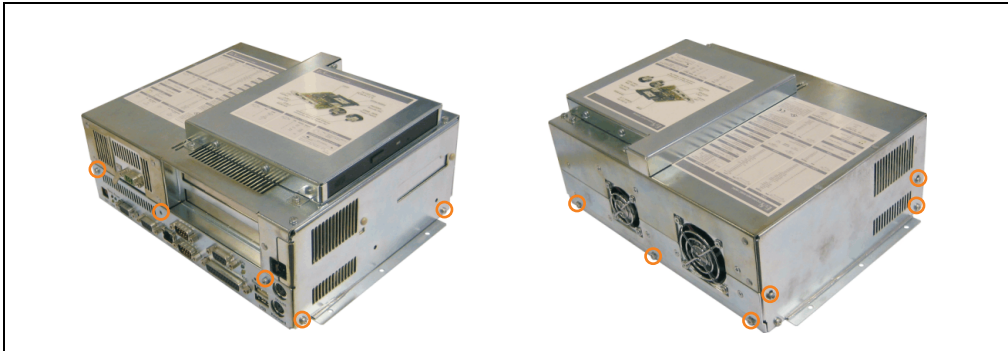
Abbildung 69: Lösen der Schrauben
