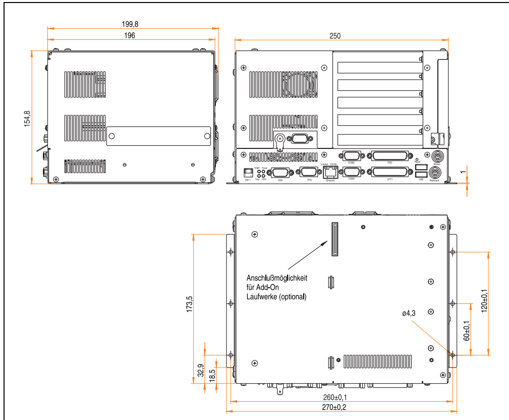
Abbildung 10: Abmessungen IPC5000C (5-Slot-Ausführung + Add-On-Laufwerksmontagemöglichkeit)
