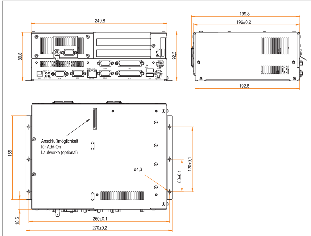
Abbildung 6: Abmessungen IPC500C (2-Slot-Ausführung + Add-On-Laufwerksmontagemöglichkeit)
