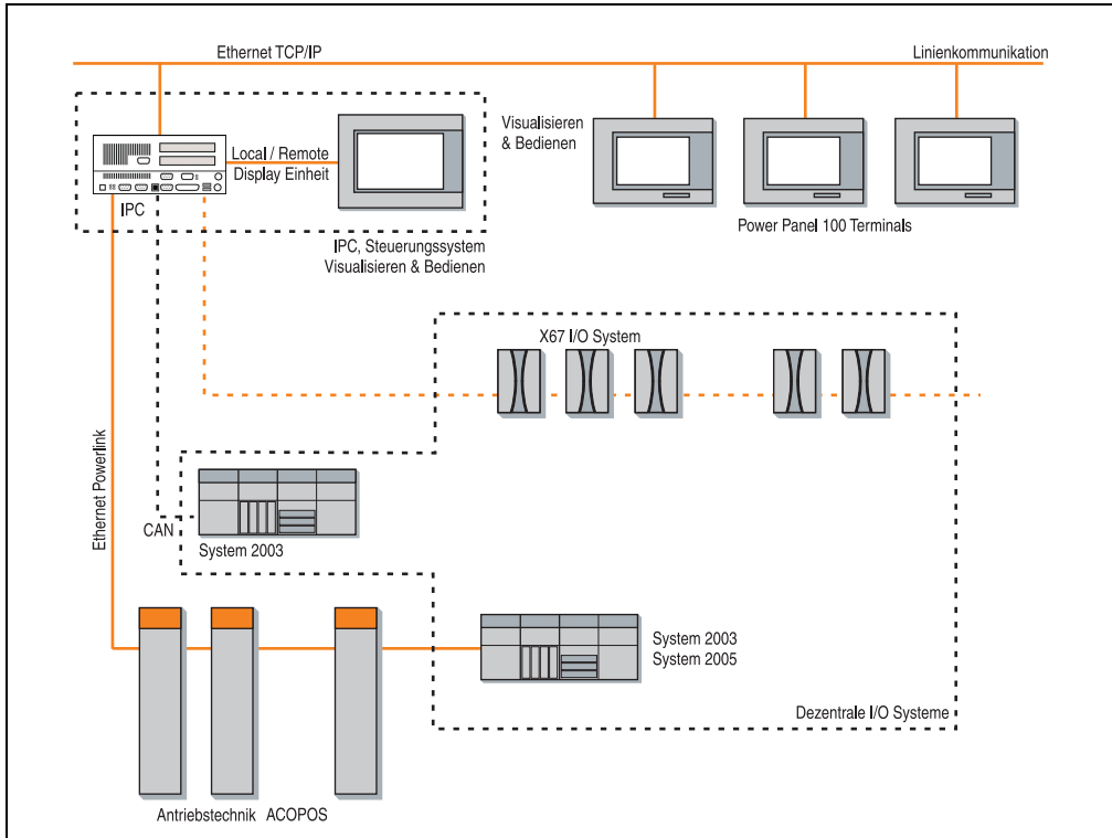
Abbildung 1: Industrie PC als zentrale Steuerung und Visualisierung
