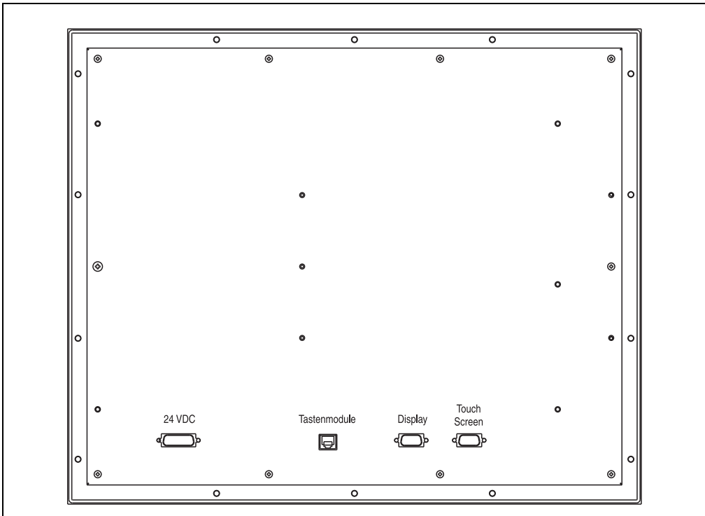
Abbildung 160: Anschlüsse 5D5213.01 Rev. < F0
