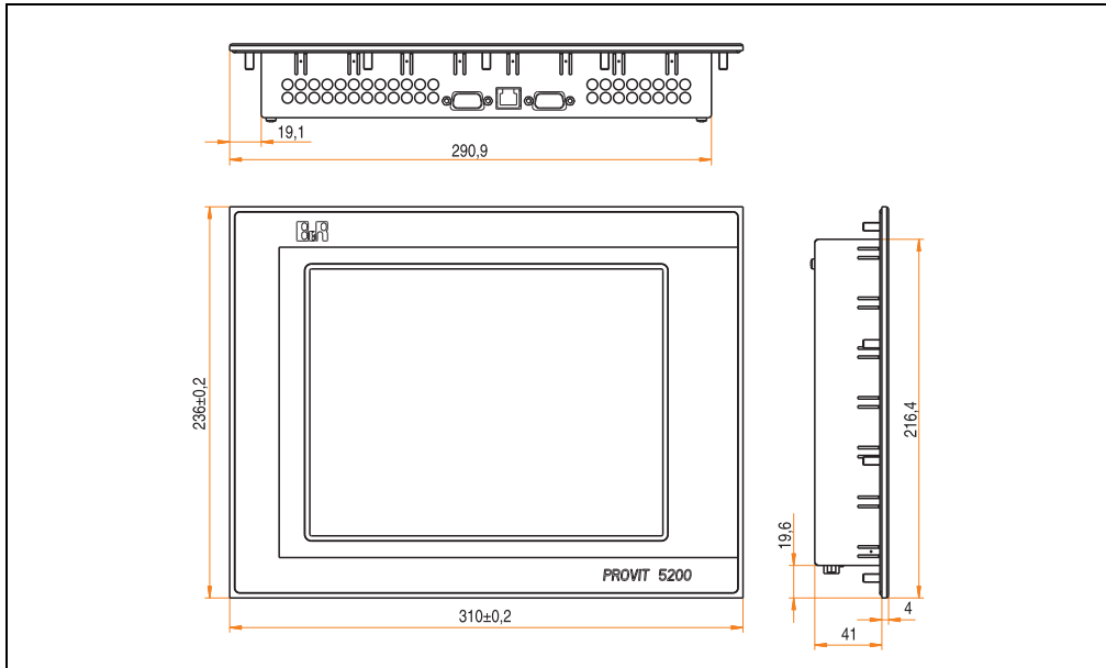
Abbildung 125: Abmessungen 5D5211.02 Rev. >= F0
