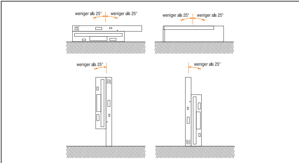
Abbildung 43: Montagevorschriften 5A5600.07
