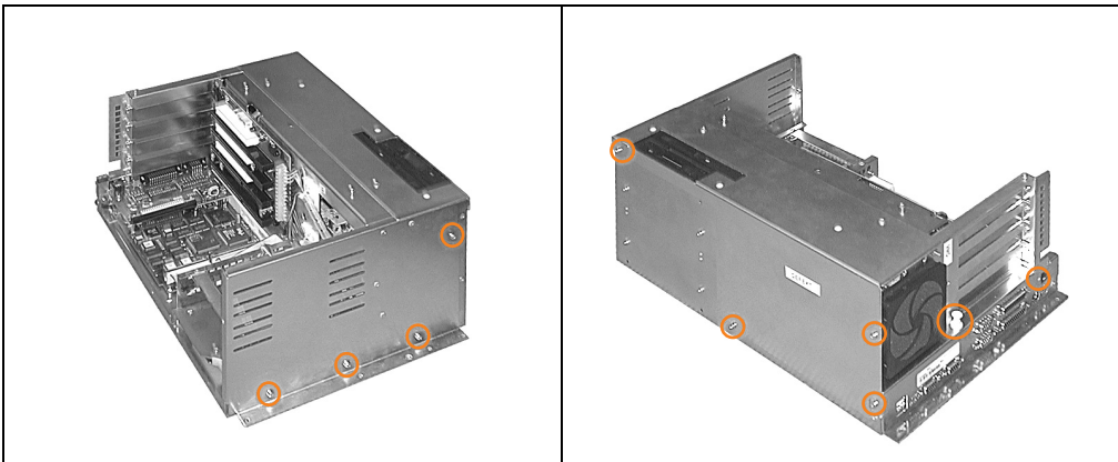
Abbildung 50: Lösen der Schrauben
