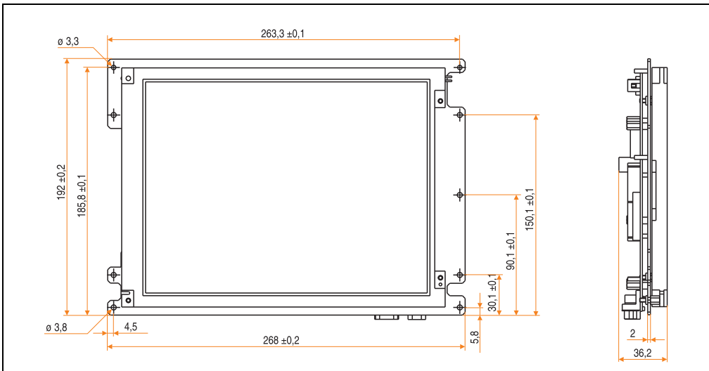
Abbildung 181: Abmessungen 5D5000.10
