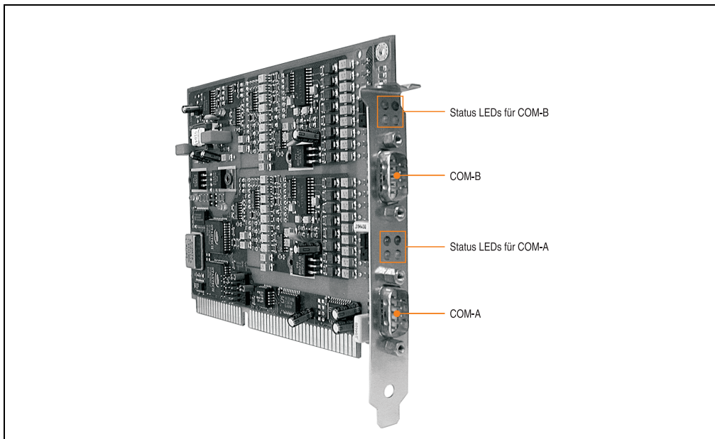
Abbildung 1: RS232-Schnittstellenkarte
