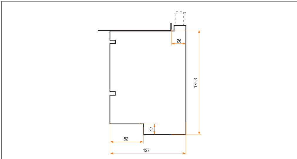
Abbildung 101: Abmessungen Interface-Karte
