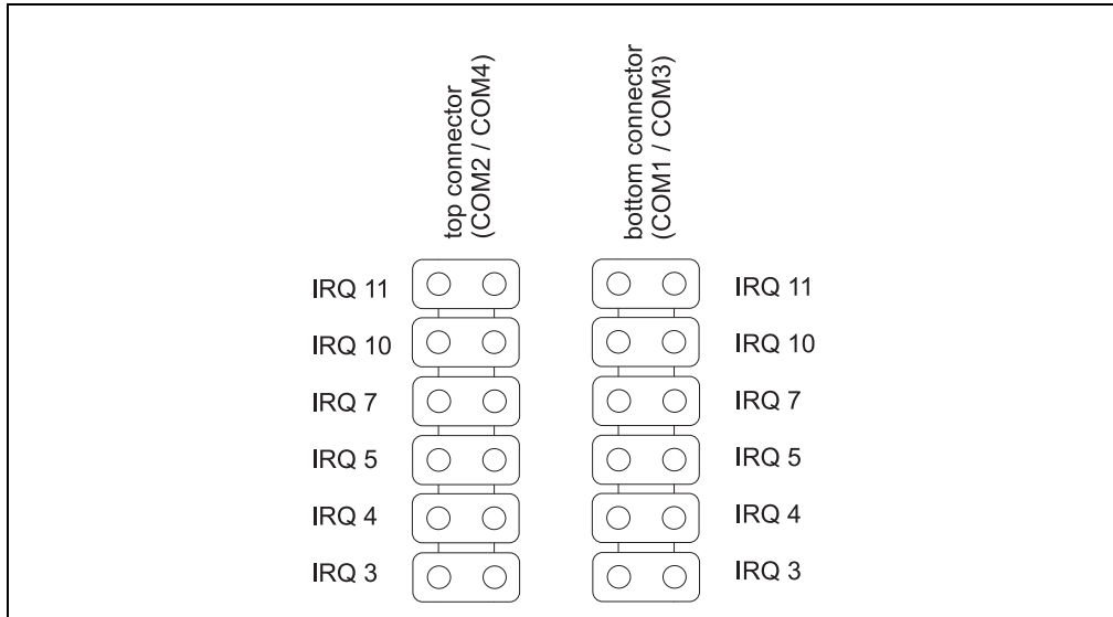
Abbildung 4: IRQ-Jumper
