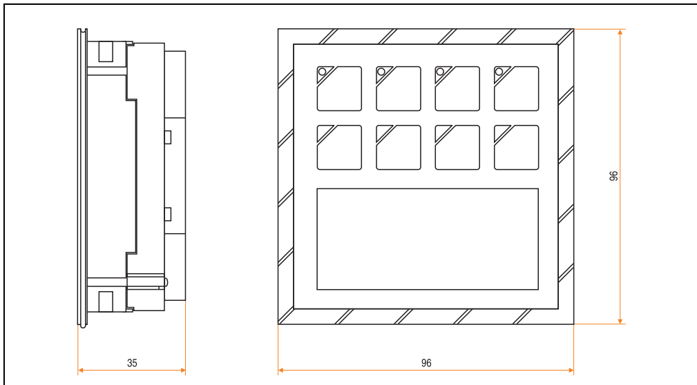
Abbildung 193: Abmessungen Tastenmodul mit 8 Tasten
