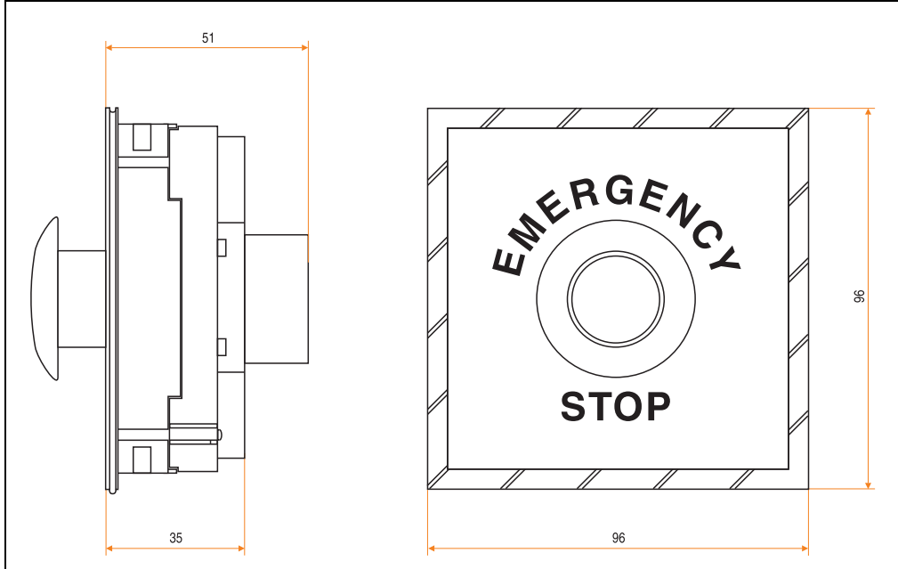
Abbildung 196: Abmessungen Tastenmodul mit Notaus-Schalter
