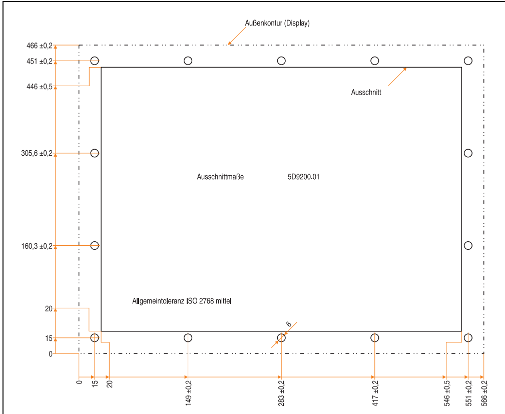
Abbildung 163: Einbau in Wanddurchbrüche 5D9200.01
