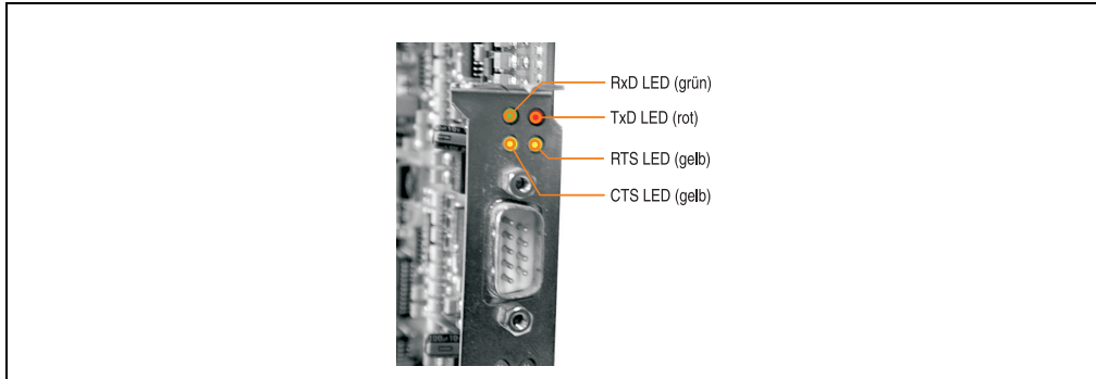
Abbildung 2: RS232-Schnittstellenkarte LEDs
