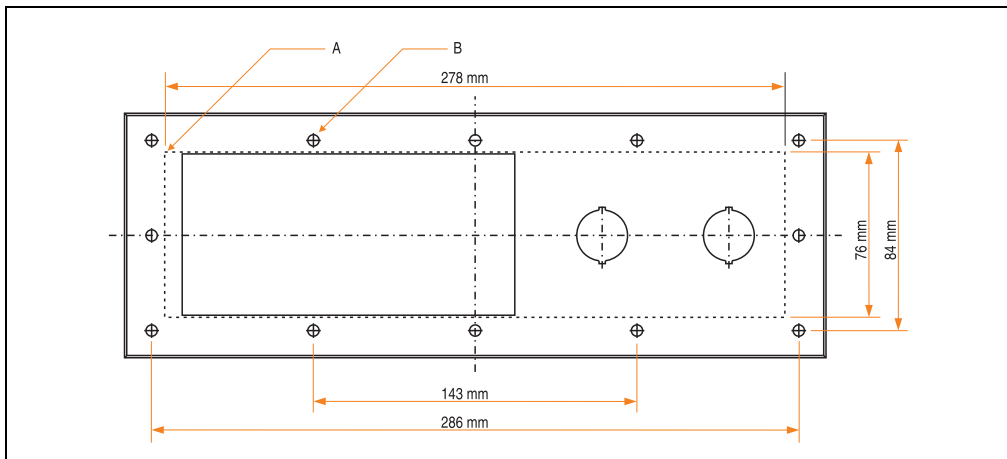
Abbildung 8: Frontplatte für externes Diskettenlaufwerk
