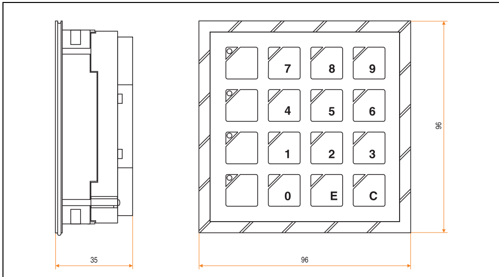
Abbildung 192: Abmessungen Tastenmodul mit 12+4 Tasten
