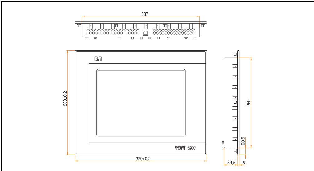
Abbildung 131: Abmessungen 5D5211.03 Rev. I0
