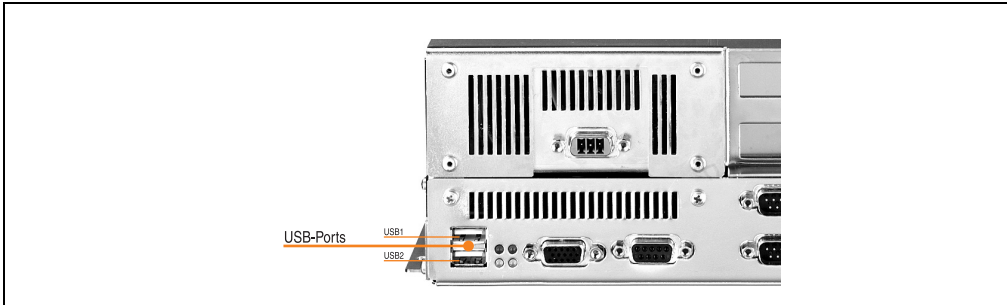
Abbildung 61: USB Ports (5C5001.01, 5C5001.03 und 5C5601.01)
