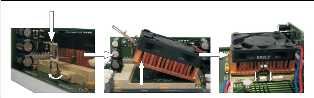
Abbildung 75: Kühlkörper abnehmen
