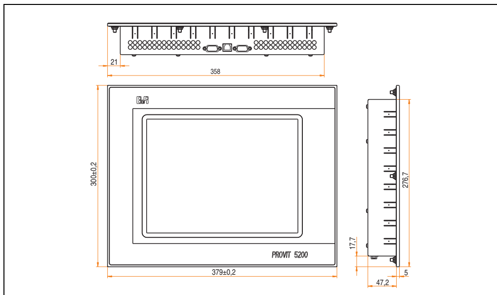
Abbildung 138: Abmessung 5D5211.06
