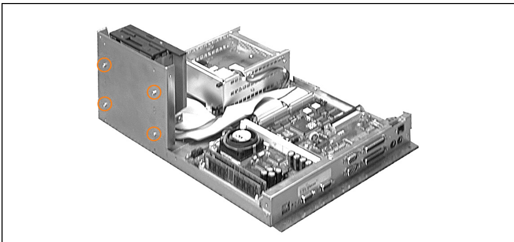
Abbildung 52: Lösen der Laufwerke
