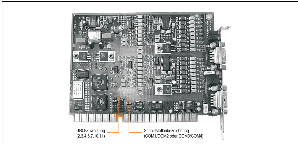
Abbildung 3: Lage der Jumper
