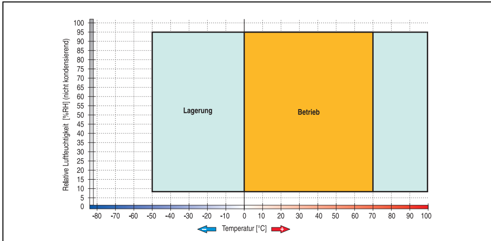
Abbildung 95: Temperatur Luftfeuchtediagramm Compact Flash Karten 5CFCRD.xxxx-03
