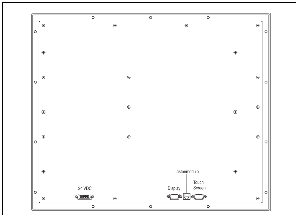
Abbildung 159: Anschlüsse 5D5213.01 Rev. >= F0
