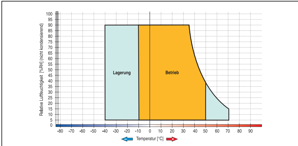
Abbildung 68: Temperatur Luftfeuchtediagramm Elo Accu Touch Screen 5 Draht
