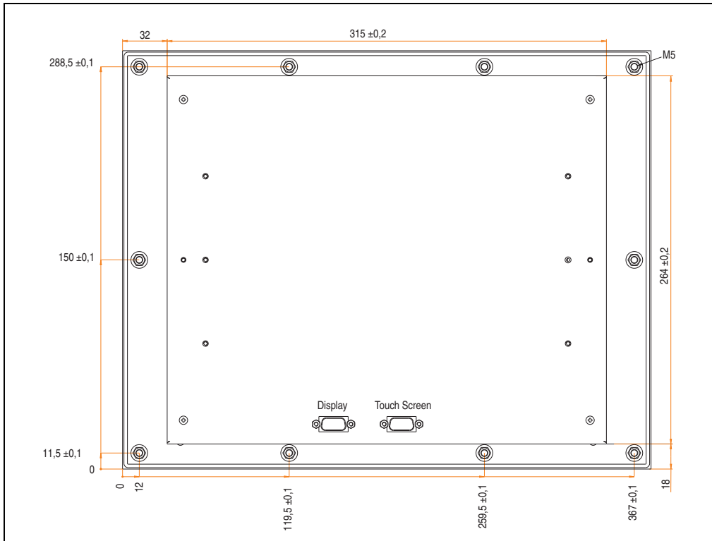
Abbildung 139: Einbau in Wanddurchbrüche 5D5211.06
