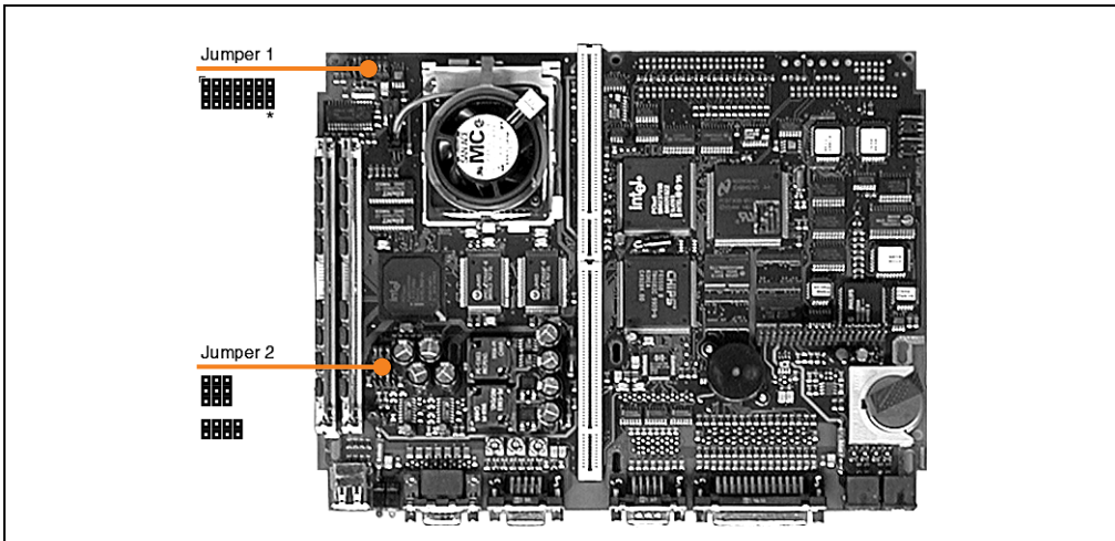
Abbildung 57: JumperEinstellungen an Mainboards mit Socket 7 (ZIF)
