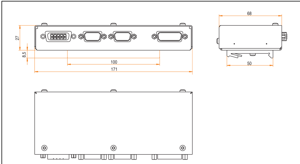
Abbildung 36: Remote Display Adapter - Local Unit 5A5010.01 Abmessungen
