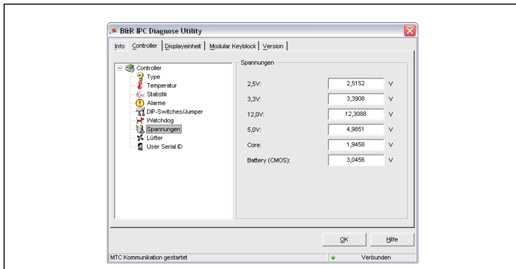
Abbildung 241: B&R IPC Diagnose Utility - Registerkarte Controller - Spannungen
