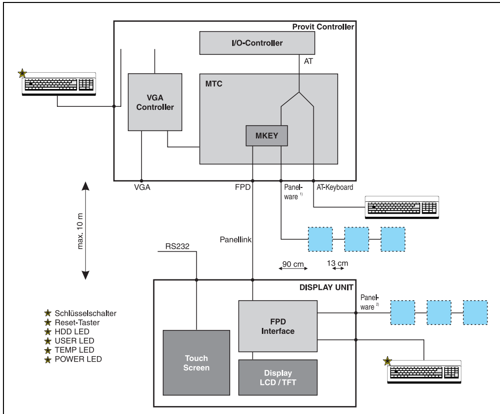
Abbildung 109: Schaltungsschema von Controller, Display und Peripherie
