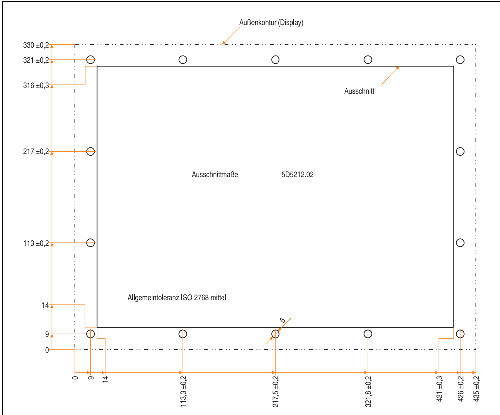
Abbildung 147: Einbau in Wanddurchbrüche 5D5212.02
