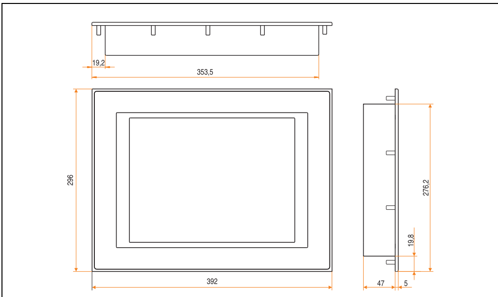
Abbildung 120: Abmessungen 5D5200.04
