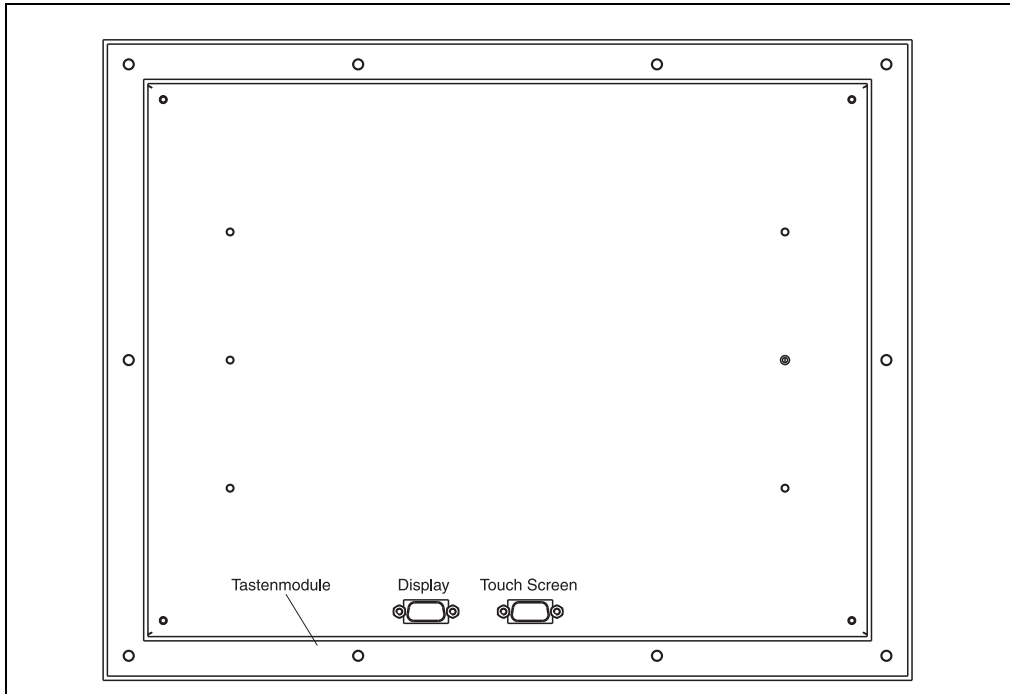
Abbildung 134: Anschlüsse 5D5201.03 und 5D5211.03
