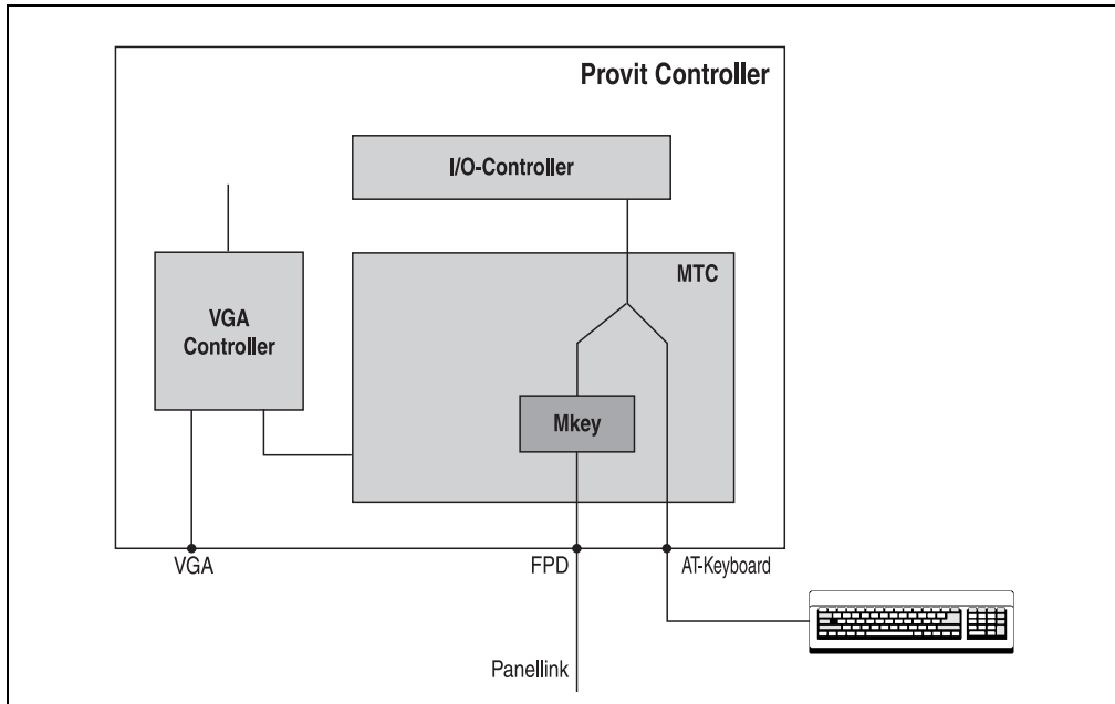
Abbildung 78: Schema MTC
