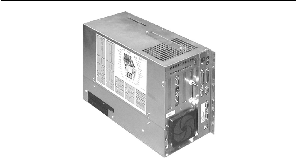
Abbildung 46: Laufwerke an der Rückseite des IPC zugänglich
