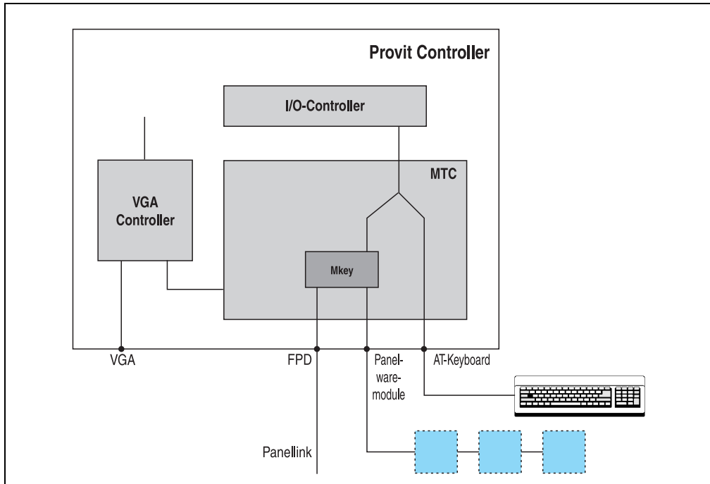
Abbildung 67: Schema Maintenance Controller (MTC)
