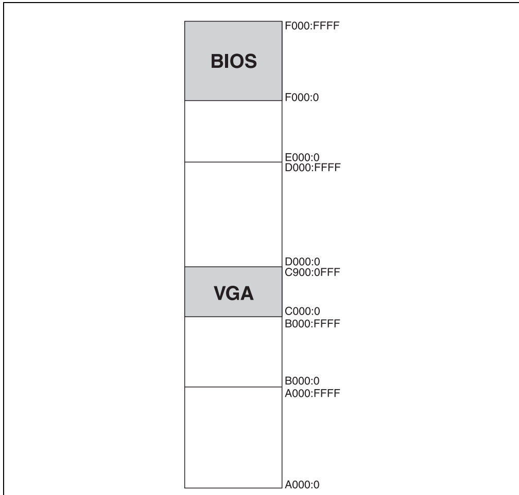
Abbildung 253: UMA-Speicheraufteilung
