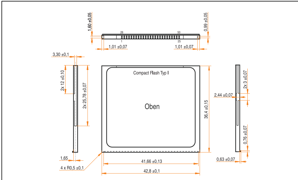
Abbildung 96: Abmessungen Compact Flash Karte Typ I
