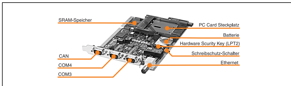
Abbildung 100: Interface-Karte
