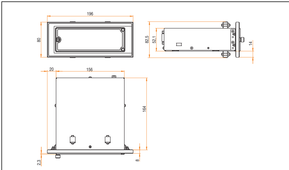
Abbildung 16: Abmessungen 5A5003.07 mit Frontklappe 5A5003.03
