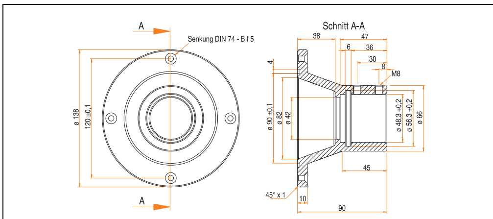
Abbildung 44: Abmessungen Panel Flansch Adapter 5A5007.01
