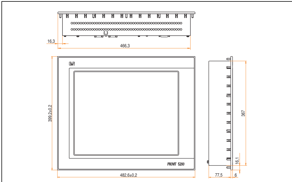
Abbildung 156: Abmessungen 5D5213.01 ab Rev. >= F0
