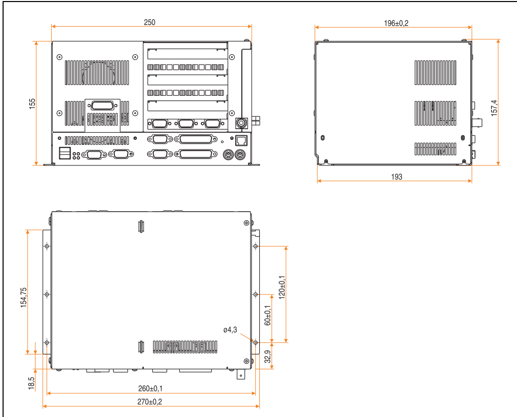
Abbildung 8: Abmessungen IPC5000 (4-Slot-Ausführung)
