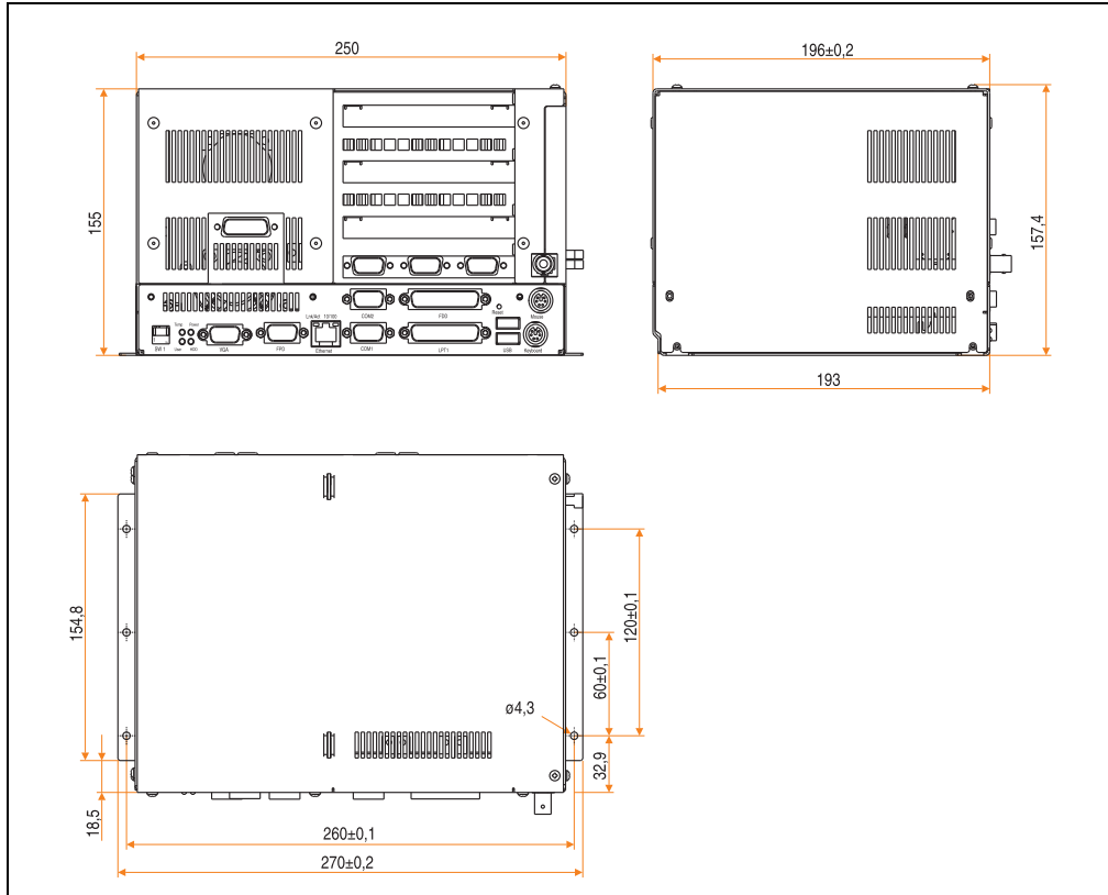
Abbildung 9: Abmessungen IPC5000C (4-Slot-Ausführung)
