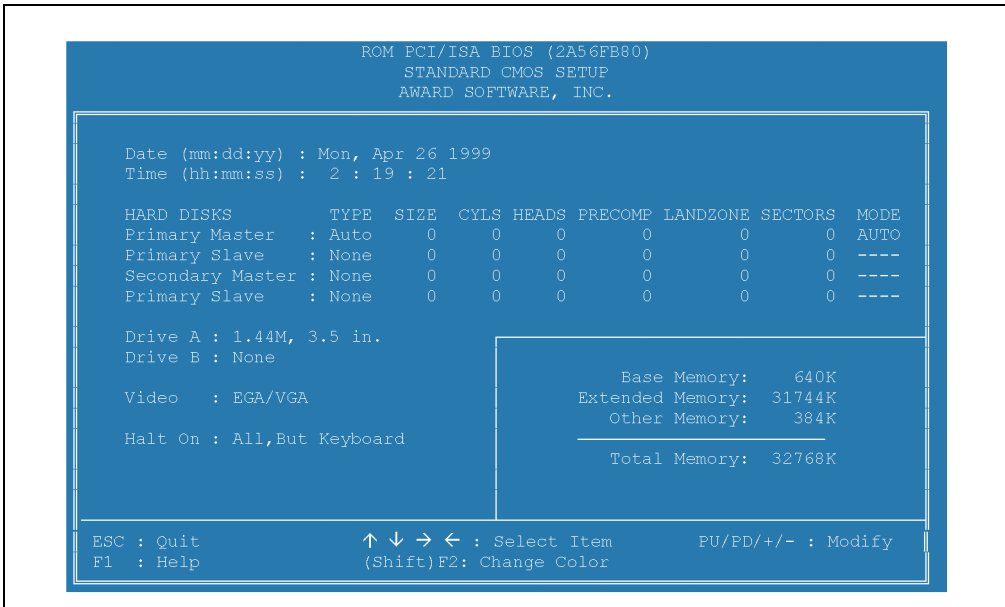
Abbildung 201: Standard CMOS Setup
