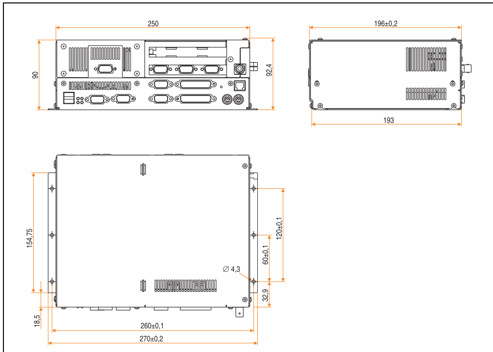
Abbildung 4: Abmessungen IPC5000 (2-Slot-Ausführung)
