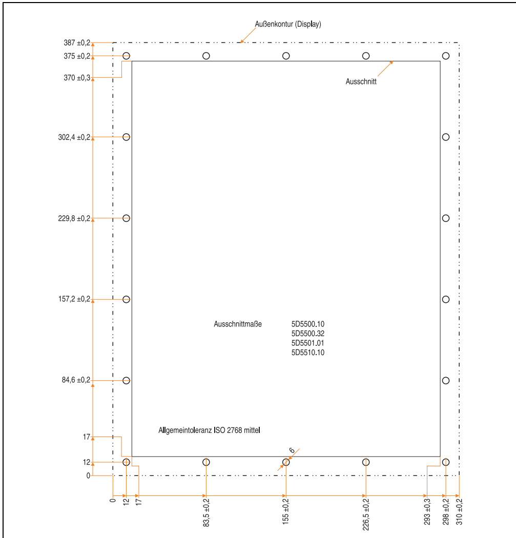
Abbildung 168: Einbau in Wanddurchbrüche 5D55xx.xx
