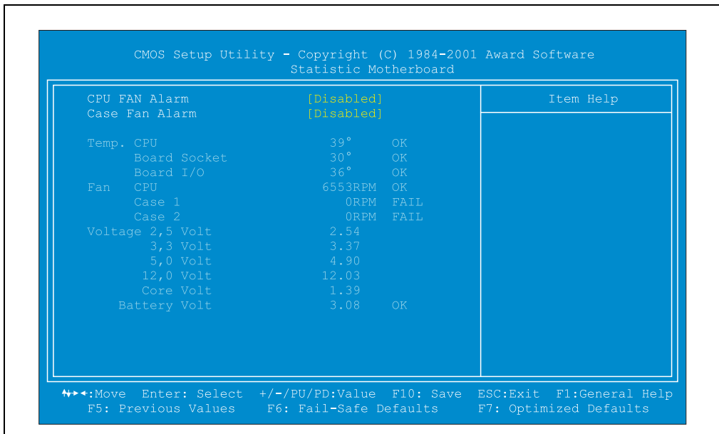
Abbildung 219: Special OEM Features - Statistik Motherboard Einstellungen
