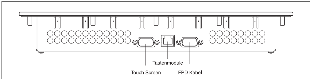
Abbildung 117: Anschlüsse 5D5200.01 und 5D5210.01 Rev. >= G0
