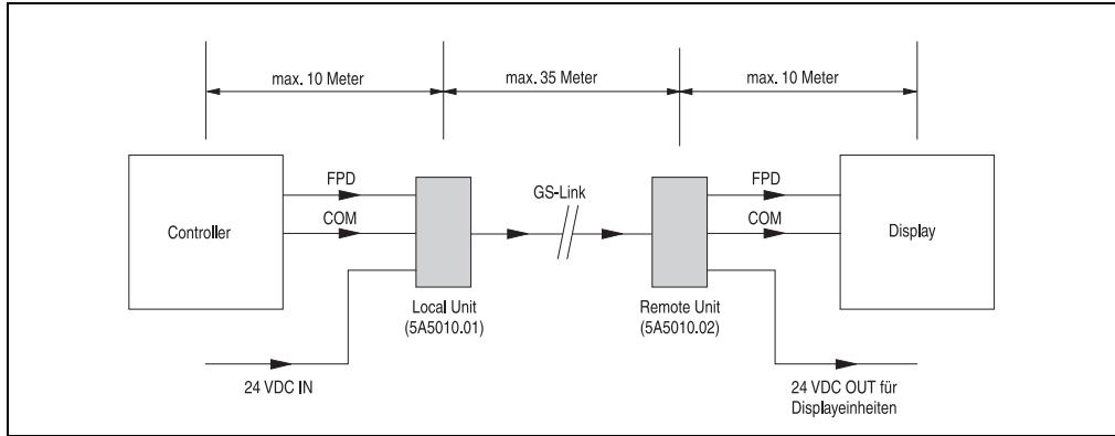
Abbildung 37: Montagekonzept
