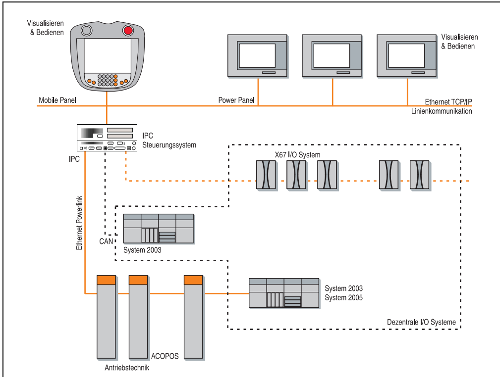
Abbildung 3: Industrie PC als Server
