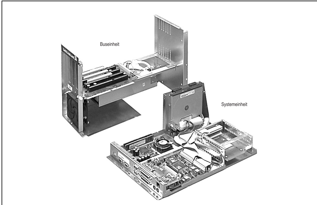
Abbildung 51: Abtrennen der Buseinheit
