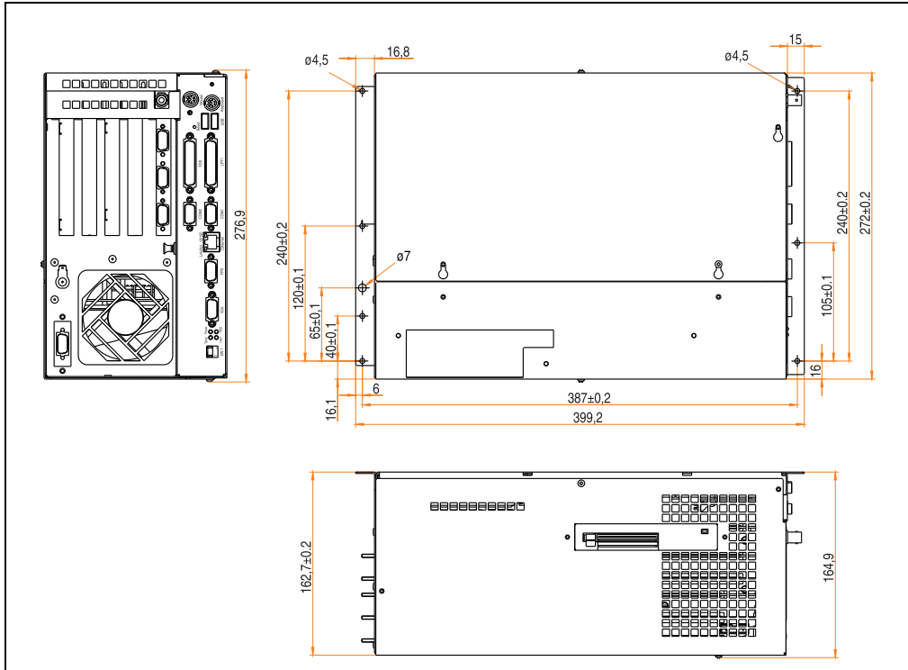
Abbildung 15: Abmessungen IPC5600C (5-Slot-Ausführung)
