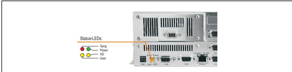
Abbildung 74: Status-LEDs IPC5000C und IPC5600C
