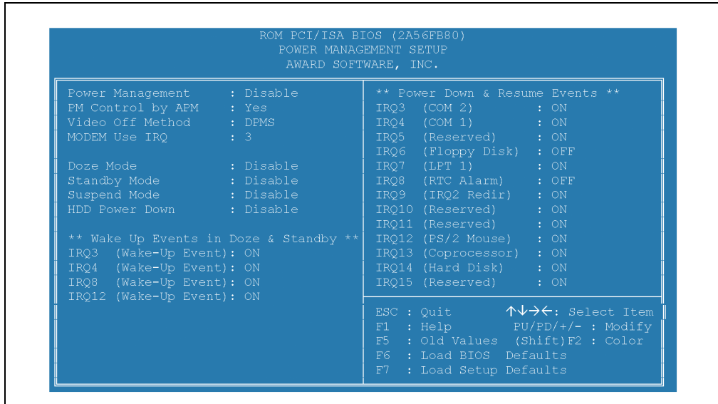
Abbildung 204: Power Management Setup
