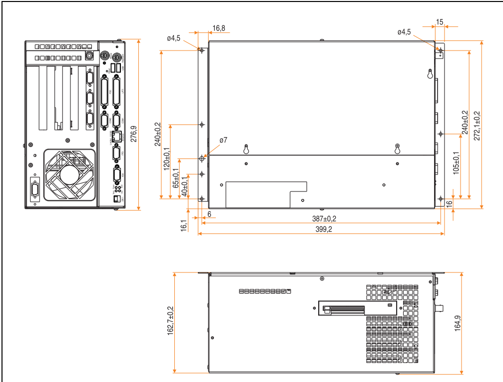
Abbildung 13: Abmessungen IPC5600C (4-Slot-Ausführung)
