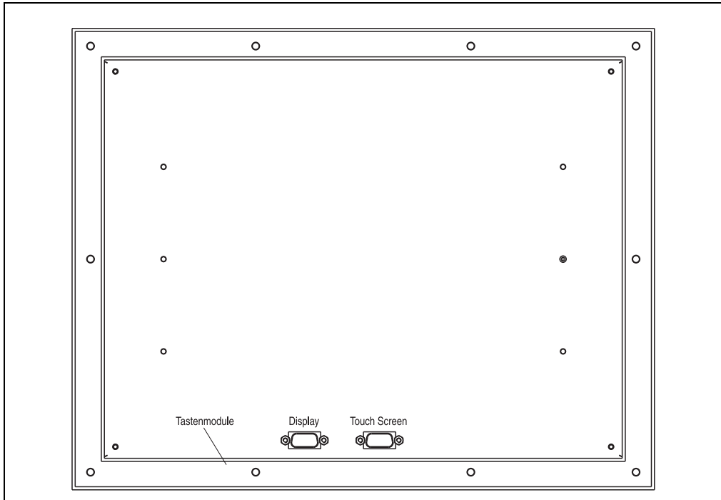
Abbildung 143: Anschlüsse 5D5202.01, 5D5202.03 und 5D5212.01
