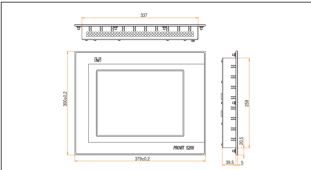
Abbildung 132: Abmessungen 5D5211.03 ab Rev. J0
