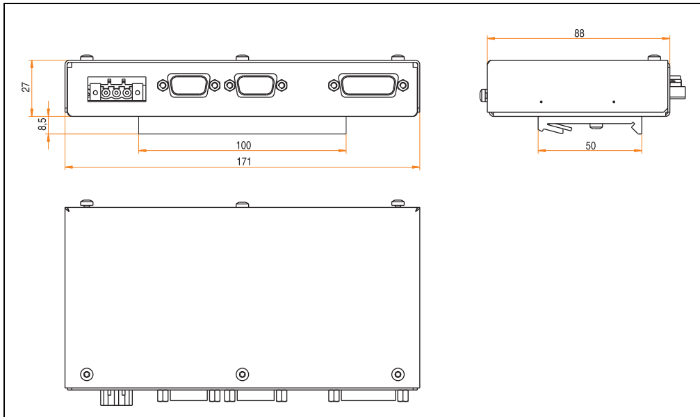
Abbildung 39: GS Link Remote Unit 5A5010.02 Abmessungen
