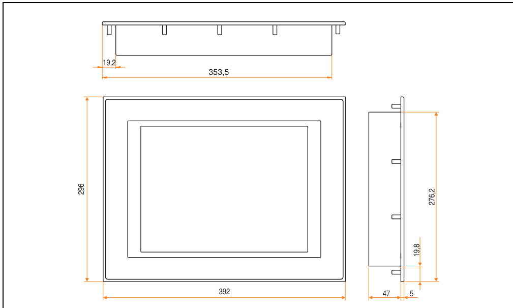
Abbildung 141: Abmessungen 5D5202.01, 5D5202.03 und 5D5212.01
