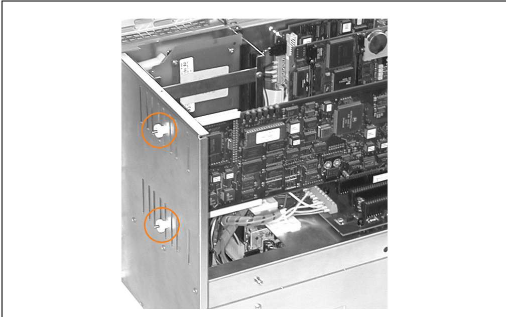
Abbildung 84: Halterungen für Full Size Steckkarten
