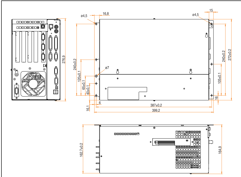
Abbildung 14: Abmessungen IPC5600 (5-Slot-Ausführung)
