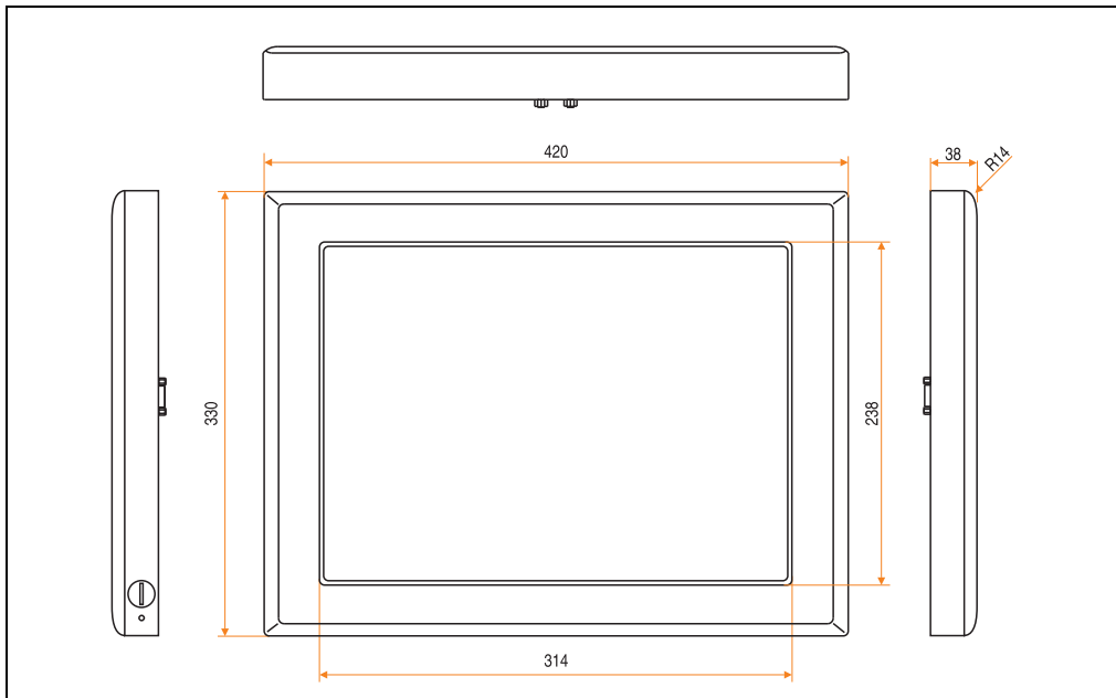
Abbildung 151: Abmessungen 5D5212.04
