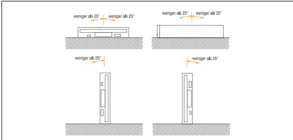
Abbildung 31: Montagevorschriften 5A5600.01
