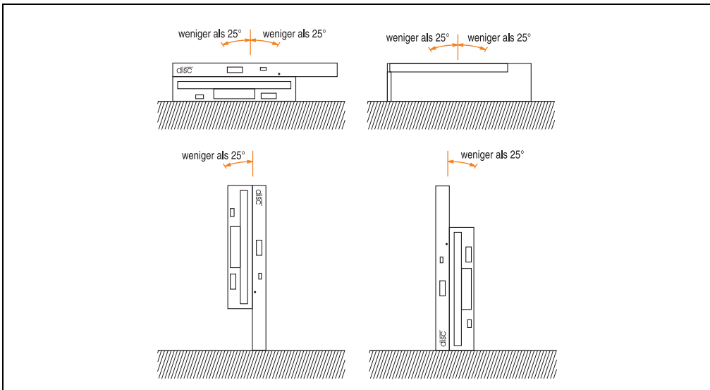
Abbildung 33: Montagevorschriften 5A5600.02
