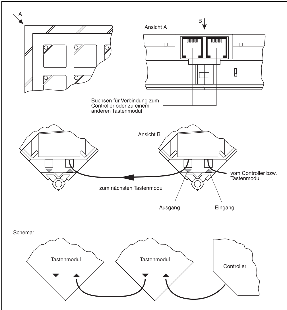
Abbildung 190: Verbindung mit dem Controller oder anderen Tastenmodulen
