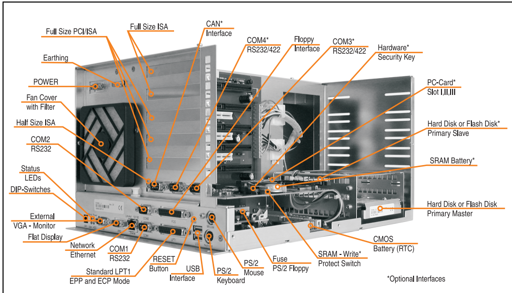
Abbildung 29: Komponenten des IPC5600C (Buseinheit mit 6 Steckplätzen)
