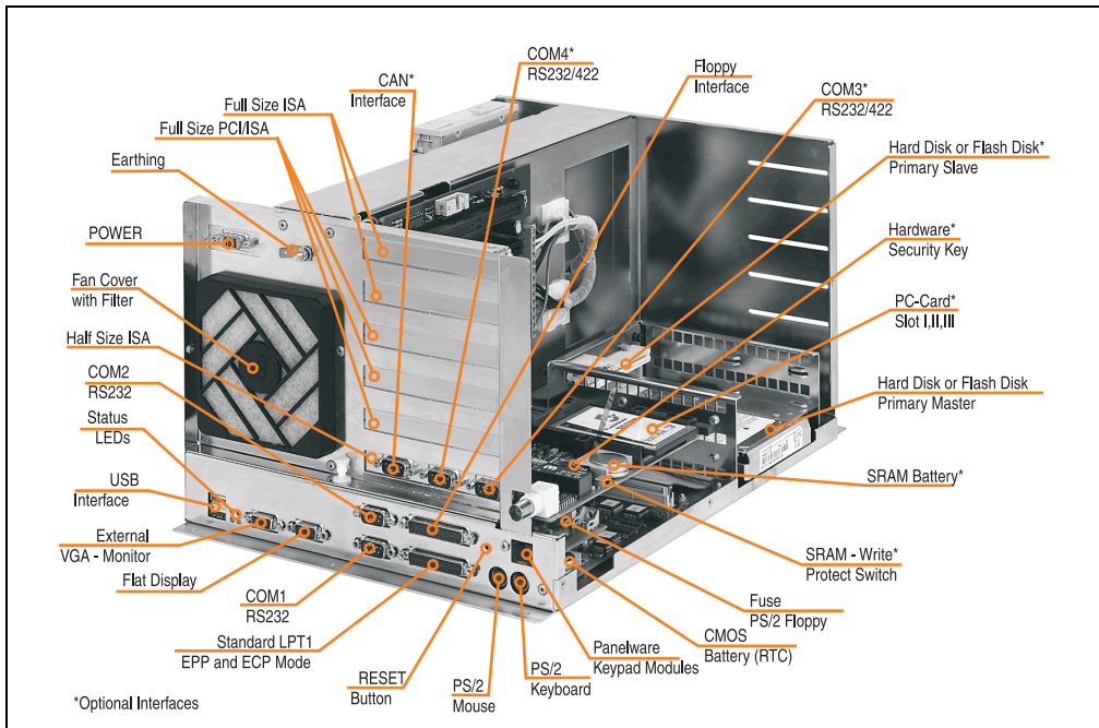
Abbildung 22: Komponenten des IPC5600 (Buseinheit mit 6 Steckplätzen)
