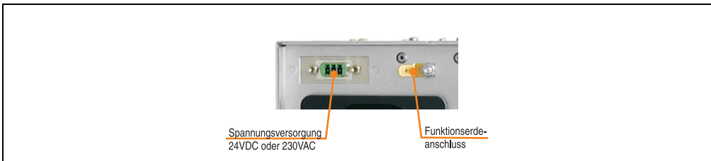
Abbildung 88: Funktionserdeanschluss IPC5600 und IPC5600C (jeweils 4, 5 und 6 Slot Ausführung)
