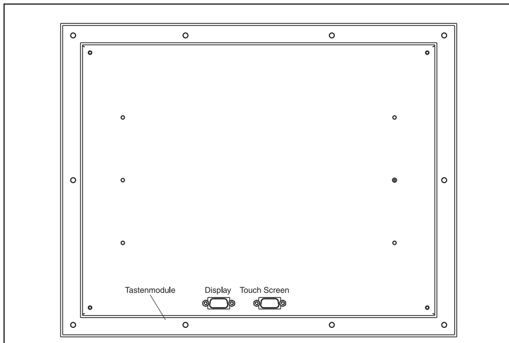
Abbildung 122: Anschlüsse 5D5200.04
