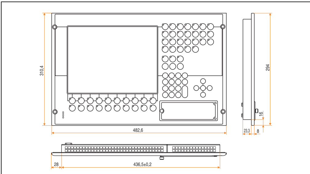
Abbildung 173: Abmessungen 5D5600.0x und 5D5601.0x
