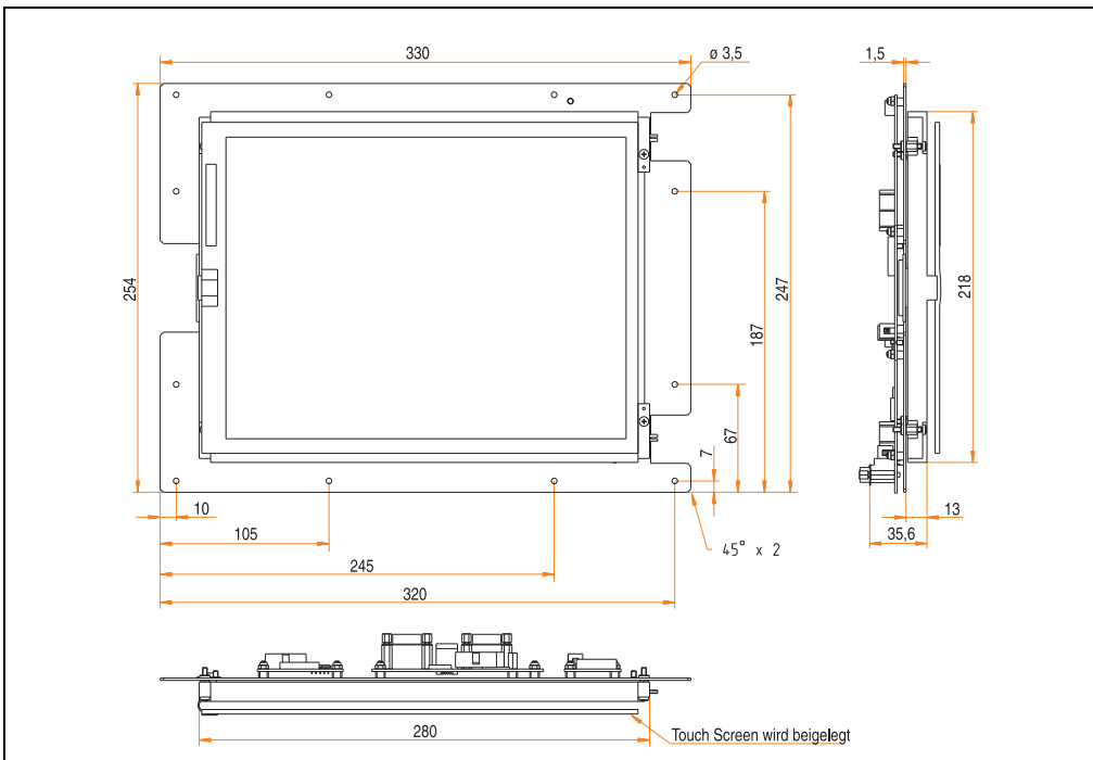
Abbildung 187: Abmessungen 5D5001.03
