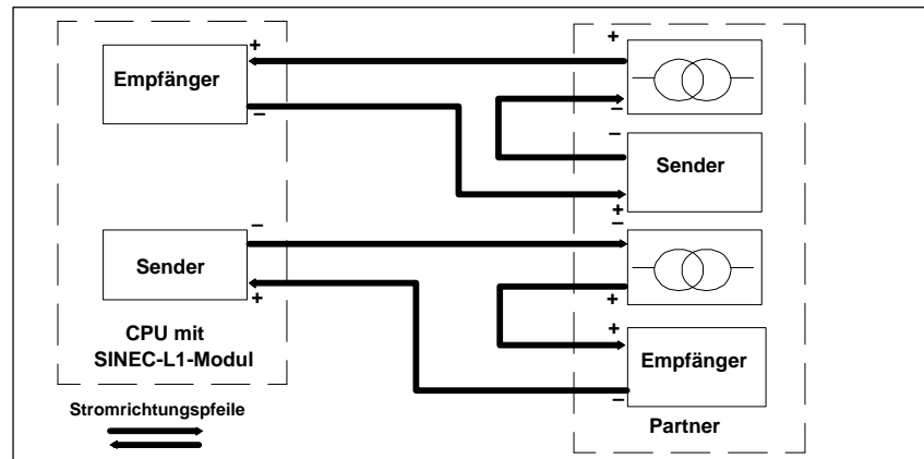
Bild 5-28 SINEC-L1-Modul: Linienstromrichtung
