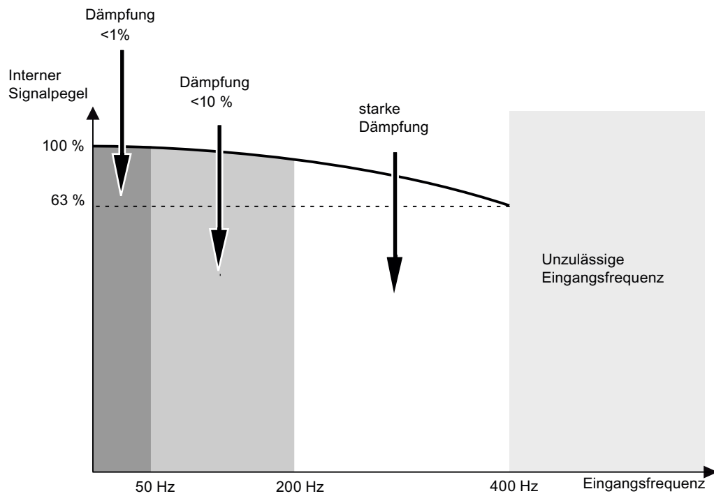
Bild 8-3 Durchlassverhalten des integrierten Tiefpassfilters
