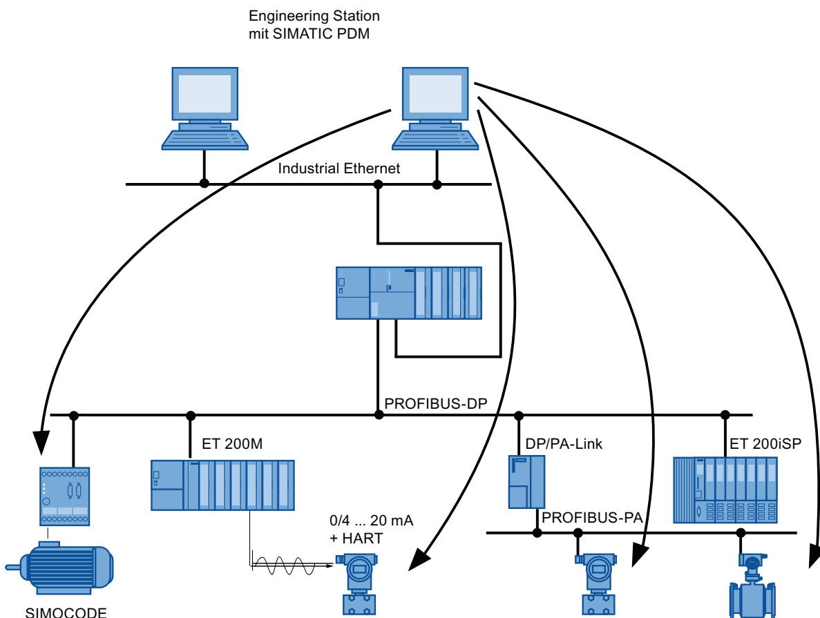
Bild 3-1 Datensatz-Routing
