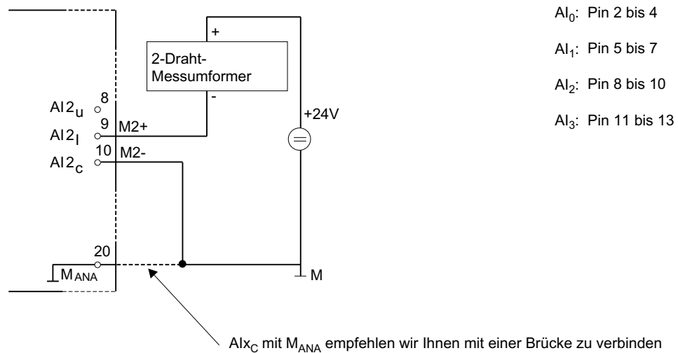
Bild 8-1 Beschaltung eines analogen Strom-/Spannungseingangs der CPU 313C/314C-2 mit 2-Draht-Messumformer
