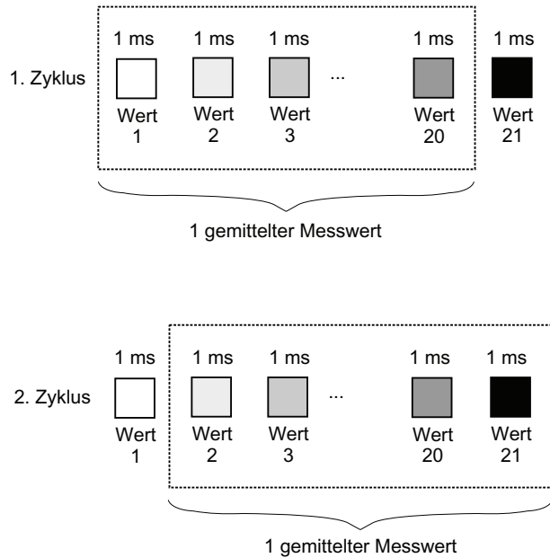
Bild 8-5 50 Hz-Störfrequenzunterdrückung
