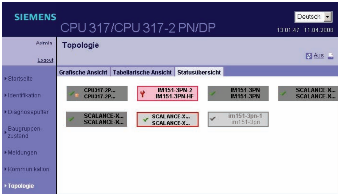
Bild 3-16 Topologie - Statusübersicht
