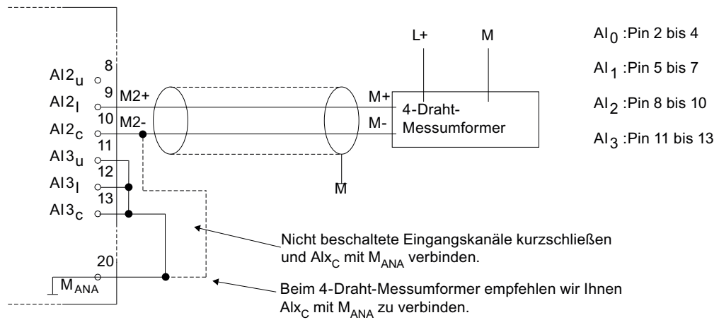
Bild 8-2 Beschaltung eines analogen Strom-/Spannungseingangs der CPU 313C/314C-2 mit 4-Draht-Messumformer
