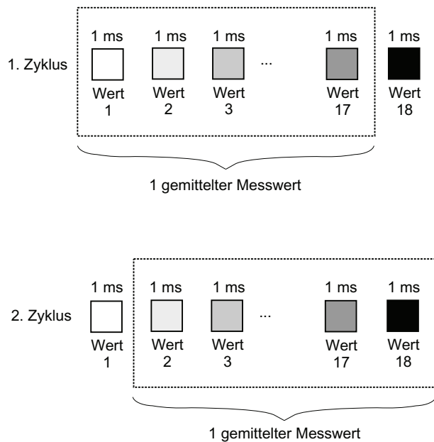
Bild 8-6 60 Hz-Störfrequenzunterdrückung
