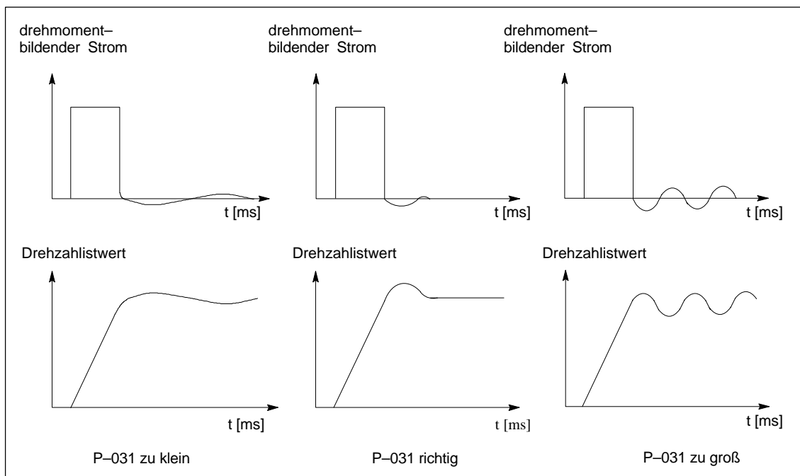
Bild 4-3 Optimierung Drehzahlregler
