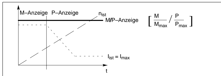
Bild 5-5 Anzeige |M/P|
