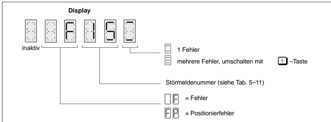
Bild 5-2 Fehleranzeige
