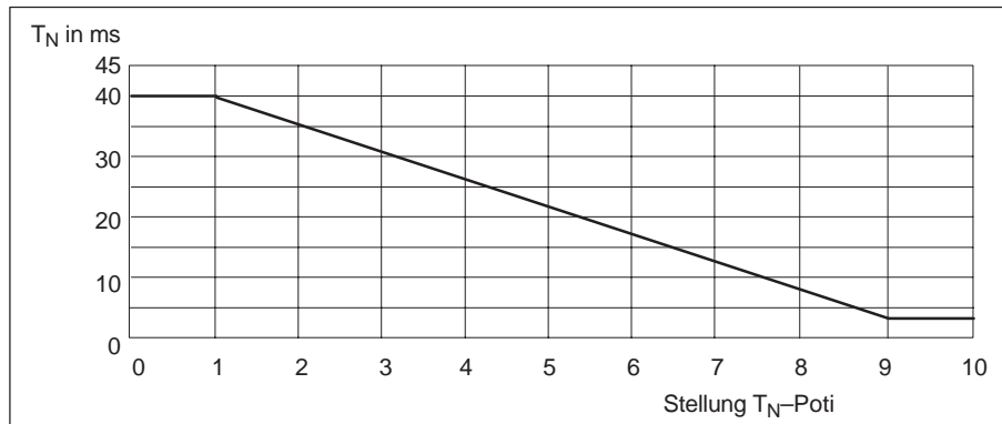
Bild 2-3 Nachstellzeit T_N in Abhängigkeit vom T_N -Poti
