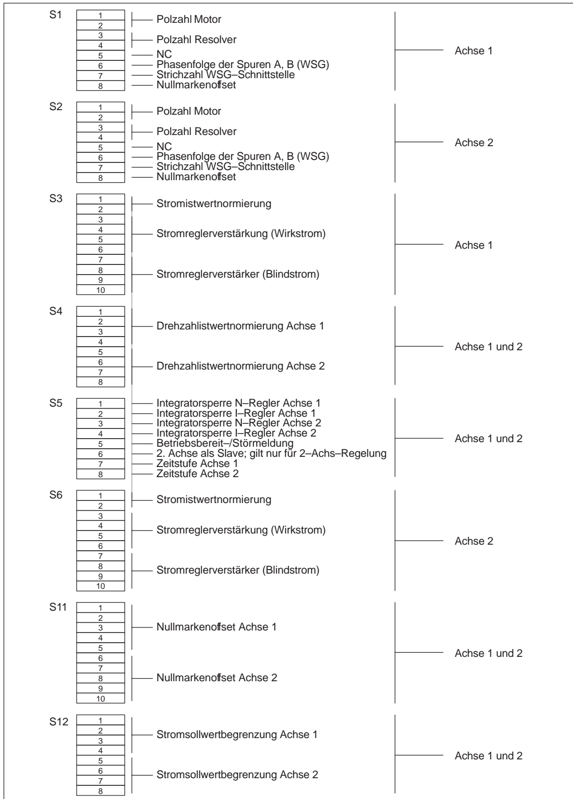
Bild 9-3 DIL-Schalter
