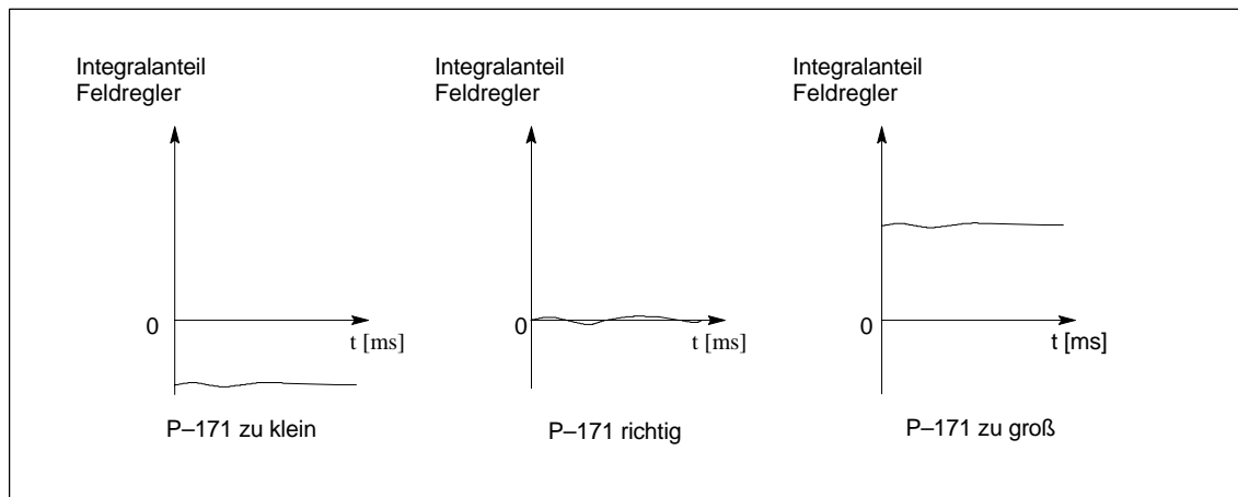
Bild 4-5 Optimierung Hauptfeldreaktanzen
