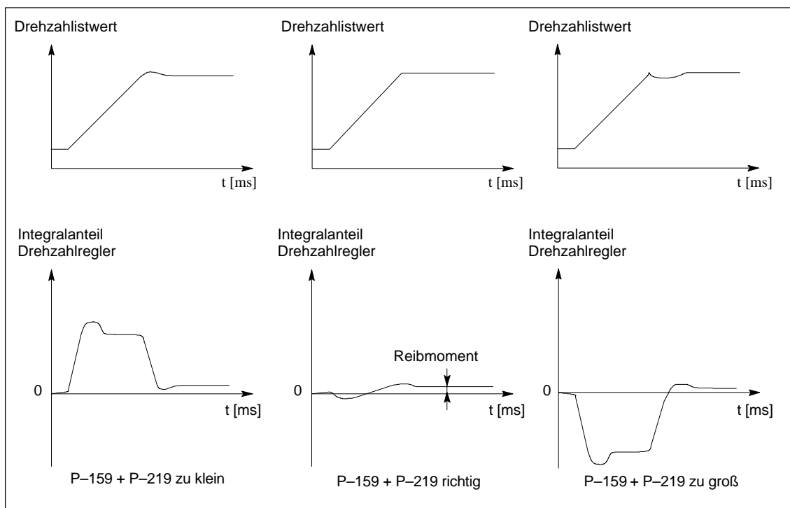
Bild 4-6 Optimierung Trägheitsmoment
