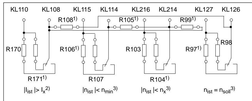
Bild 5-2 Relaisfunktionen
