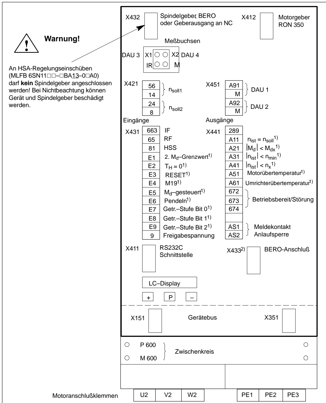
Bild 1-3 Anschlußoberfläche
