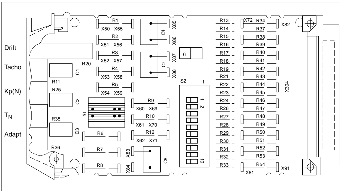
Bild 9-2 Übersichtsbild Einstellbaugruppe
