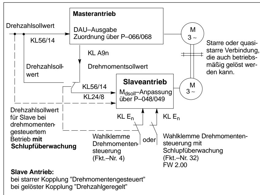
Bild 2-2 Master/Slavebetrieb
