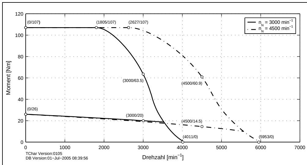
Abbildung 49: Drehzahl-Drehmomentkennlinie 8LSA73.eennnffgg-0
