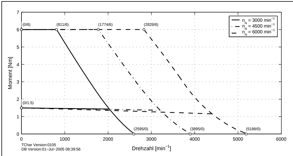
Abbildung 20: Drehzahl-Drehmomentkennlinie 8LSA34.eennnffgg-0
