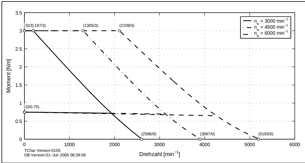
Abbildung 19: Drehzahl-Drehmomentkennlinie 8LSA33.eennnffgg-0
