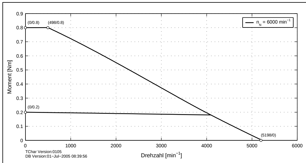
Abbildung 11: Drehzahl-Drehmomentkennlinie 8LSA23.eennnffgg-0
