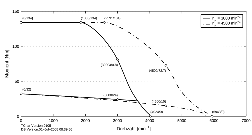
Abbildung 50: Drehzahl-Drehmomentkennlinie 8LSA74.eennnffgg-0
