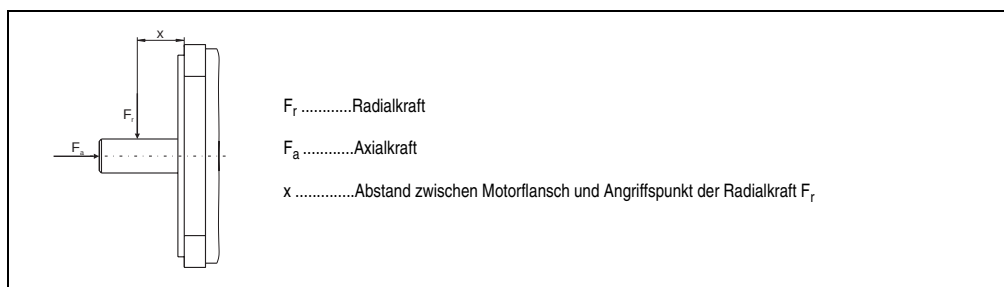
Abbildung 6: Definitionen für Diagramme zur zulässigen Wellenbelastung
