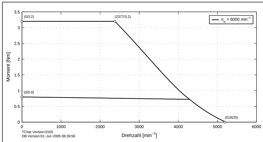
Abbildung 14: Drehzahl-Drehmomentkennlinie 8LSA26.eennnffgg-0
