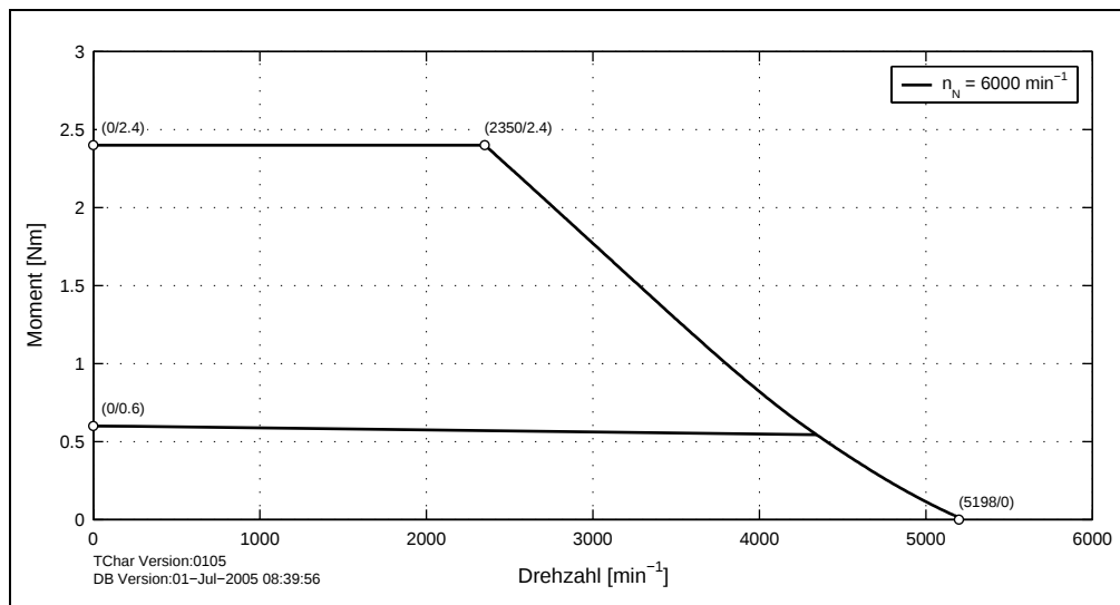
Abbildung 13: Drehzahl-Drehmomentkennlinie 8LSA25.eennnffgg-0
