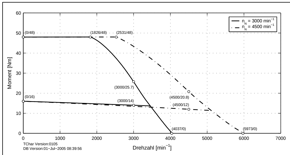
Abbildung 34: Drehzahl-Drehmomentkennlinie 8LSA56.eennnffgg-0
