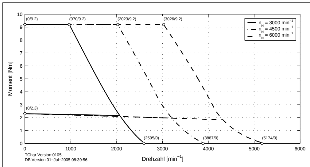
Abbildung 21: Drehzahl-Drehmomentkennlinie 8LSA35.eennnffgg-0
