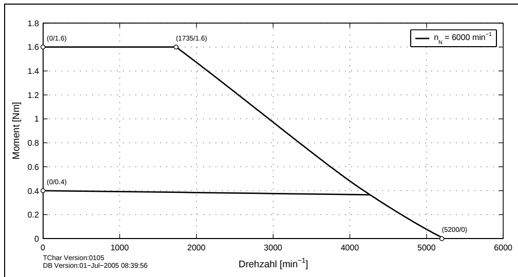
Abbildung 12: Drehzahl-Drehmomentkennlinie 8LSA24.eennnffgg-0
