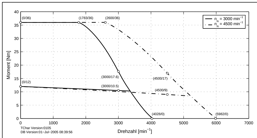
Abbildung 33: Drehzahl-Drehmomentkennlinie 8LSA55.eennnffgg-0
