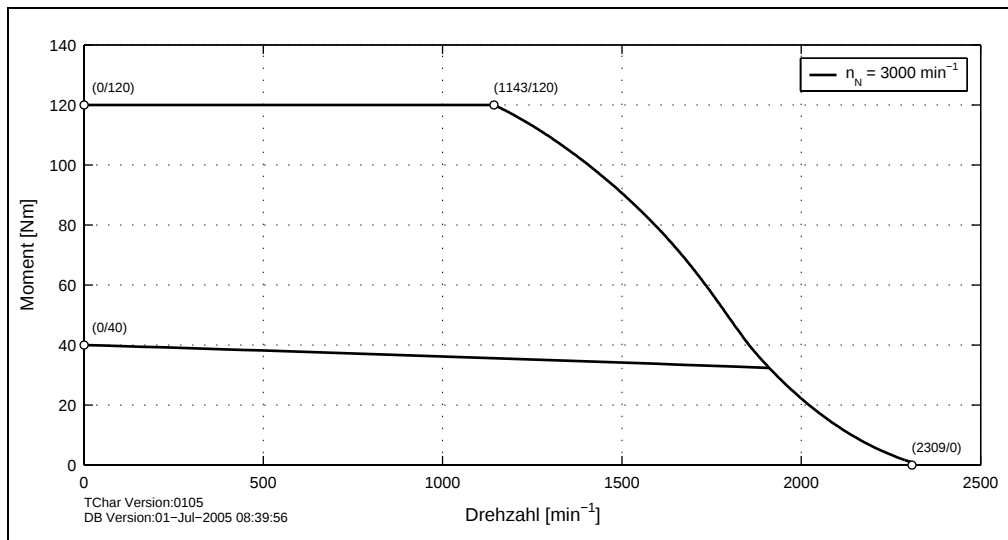
Abbildung 59: Drehzahl-Drehmomentkennlinie 8LSA83.eennnffgg-0
