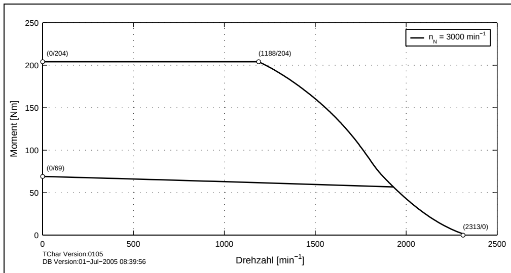
Abbildung 60: Drehzahl-Drehmomentkennlinie 8LSA84.eennnffgg-0
