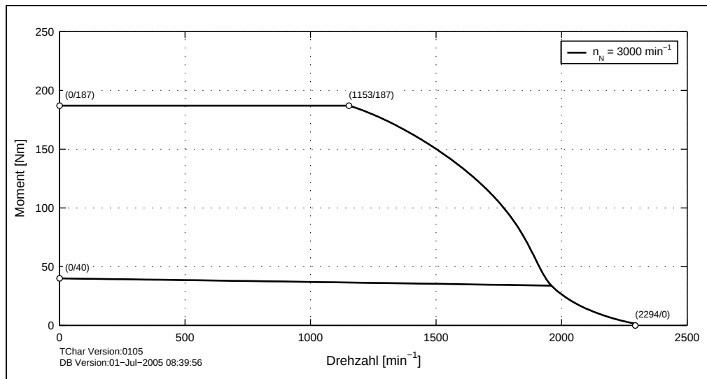
Abbildung 54: Drehzahl-Drehmomentkennlinie 8LSA75.eennnffgg-0
