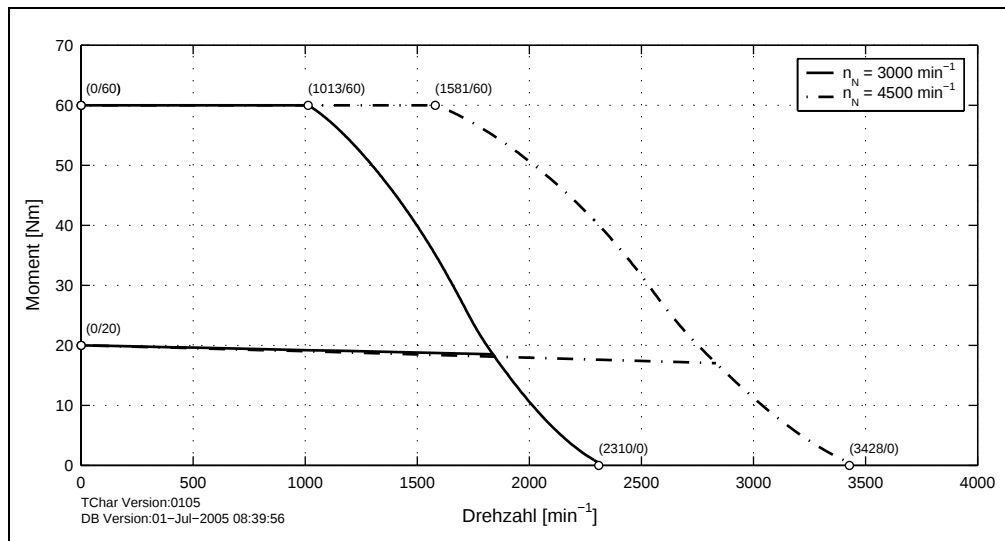
Abbildung 40: Drehzahl-Drehmomentkennlinie 8LSA57.eennnffgg-0
