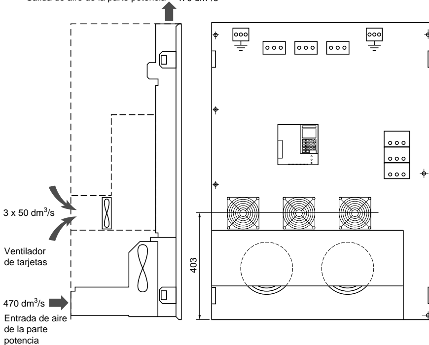
Apertura de entrada de aire parte potencia
