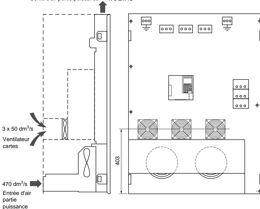
Ouverture de l'entrée d'air partie puissance
