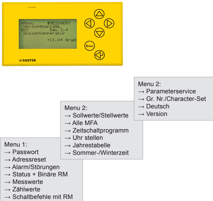
Abb. 2 Lokales Bediengerät modu240
