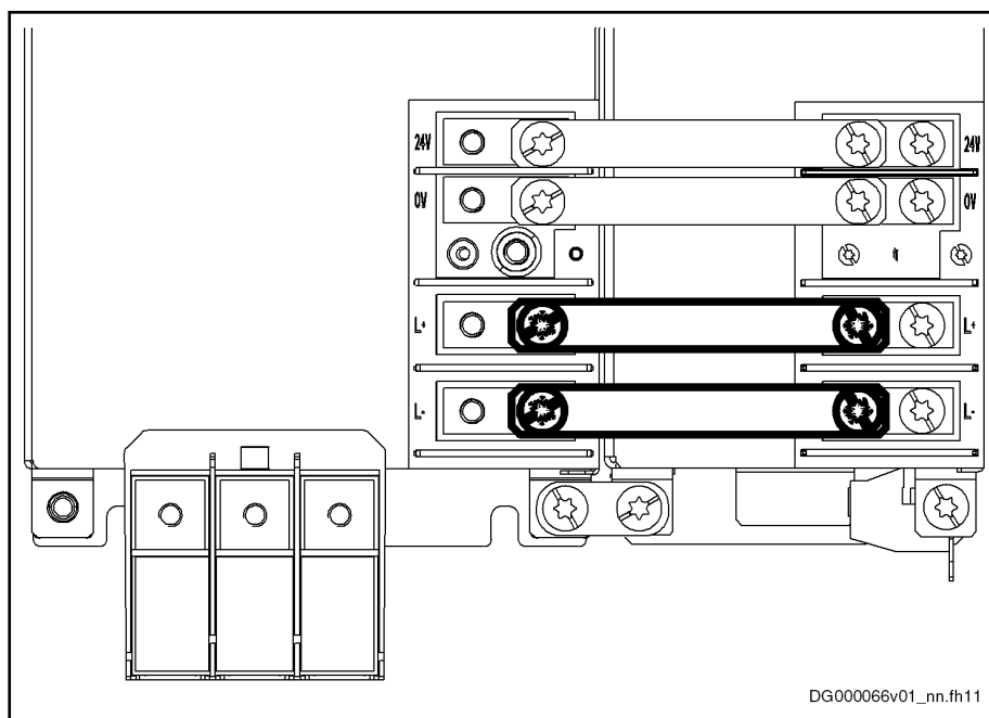
Abb.5-16: Zwischenkreisanschluss mit Stromschiene
