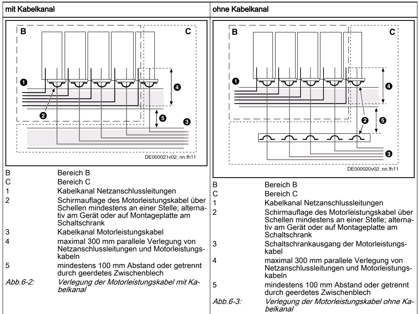
Abb.6-4: Verlegung der Kabel für Umrichter
