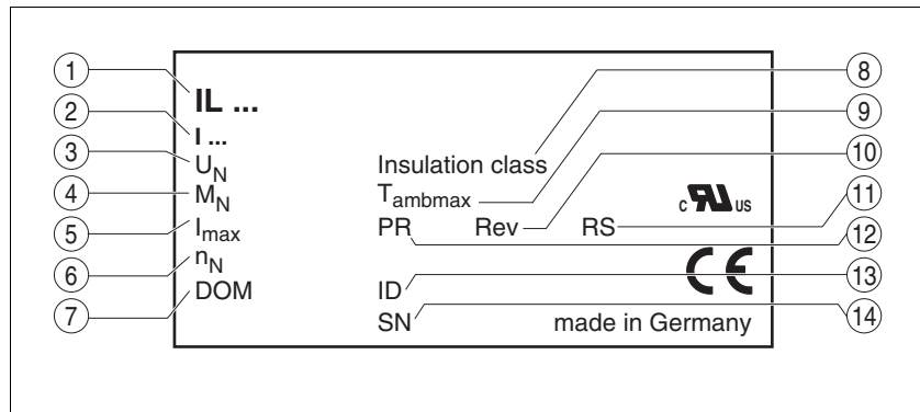
Bild 1.4 Typenschild
