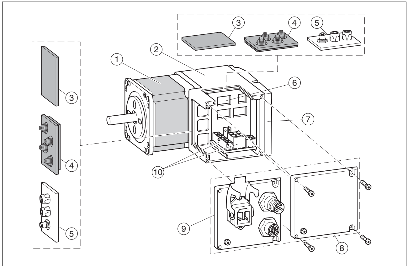
Bild 1.3 Komponenten und Schnittstellen
