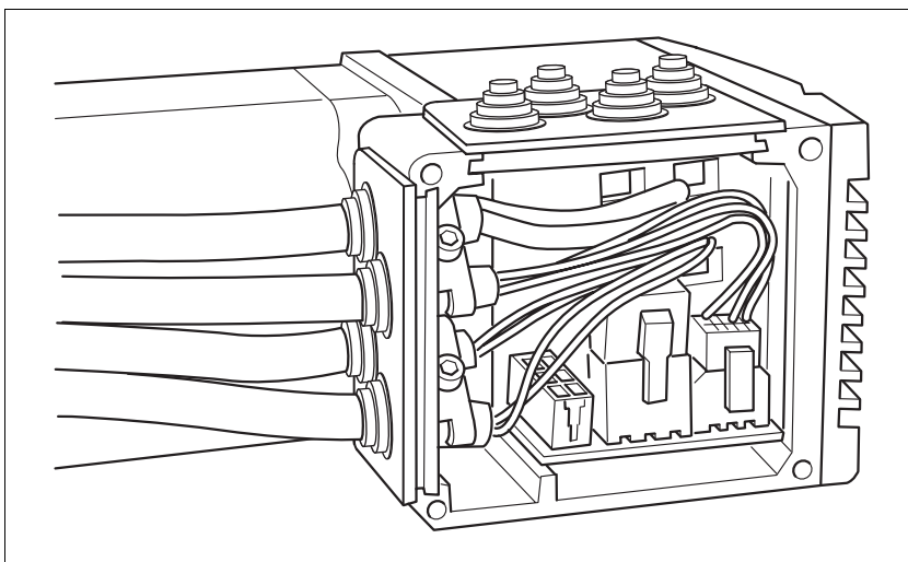
Bild 6.5 Kabeldurchführungen einstecken
