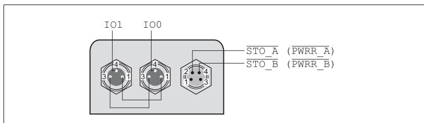
Bild 6.21 Pin-Belegung
