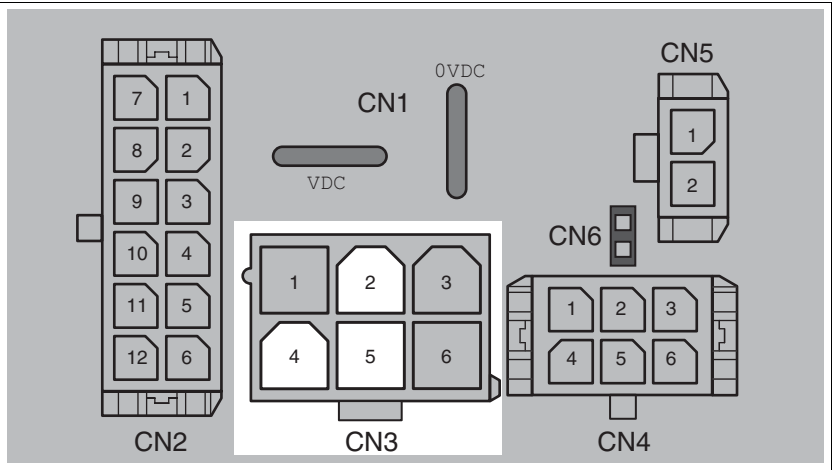
Bild 6.16 Pin-Belegung RS485
