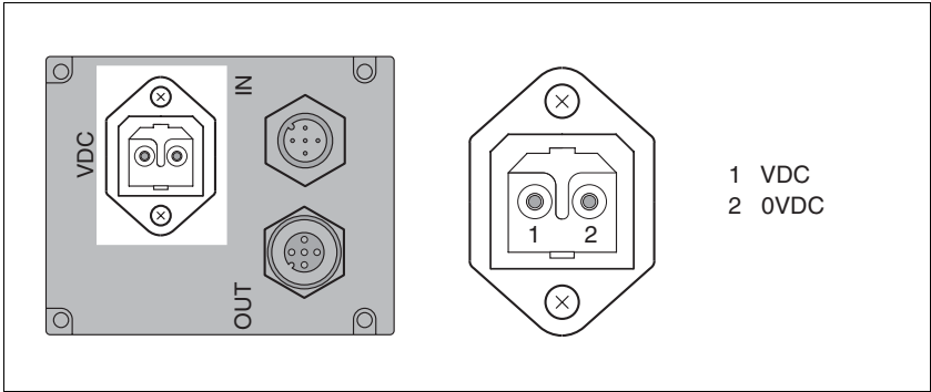
Bild 6.7 Pin-Belegung der Versorgungsspannung
