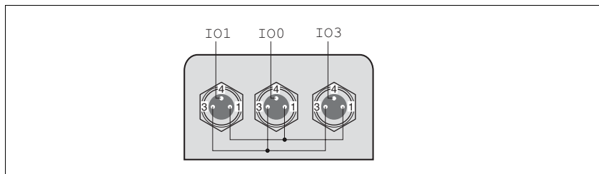
Bild 6.20 Pin-Belegung
