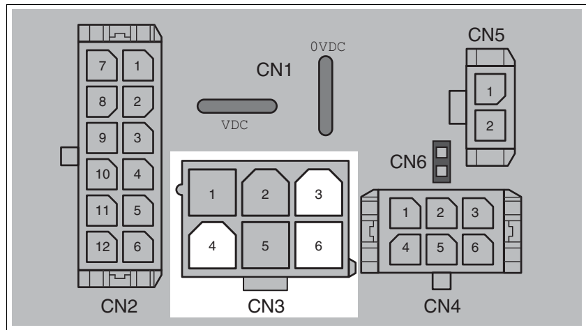
Bild 6.13 Pin-Belegung der Feldebusschnittstelle CAN
