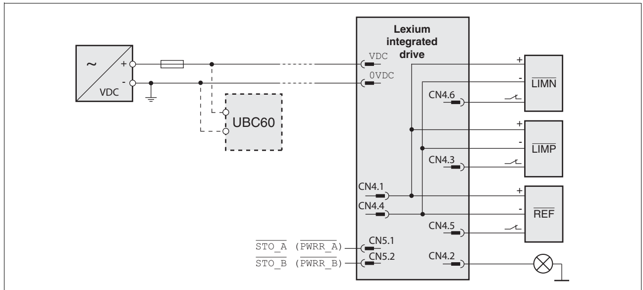
Bild 6.1 Verdrahtungsbeispiel
