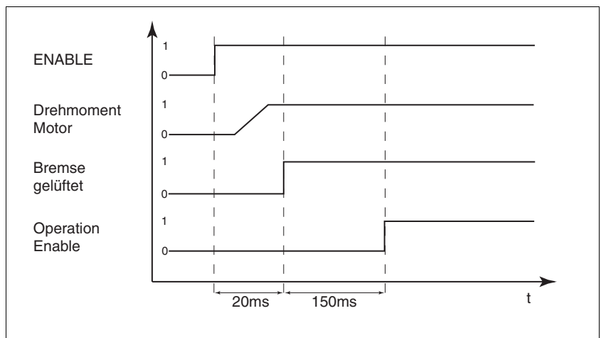
Bild 8.8 Lüften der Haltebremse
