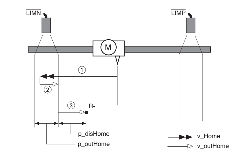
Bild 8.4 Referenzfahrt auf den negativen Endschalter
