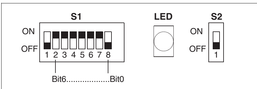
Bild 6.9 Parameterschalter
