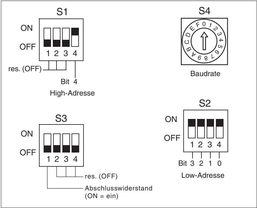
Bild 6.15 Parameterschalter
