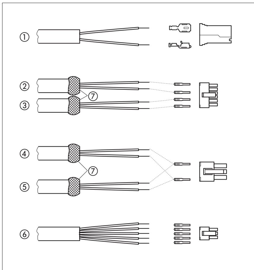
Bild 6.4 Stecker, Kabelschuhe und Crimpkontakte
