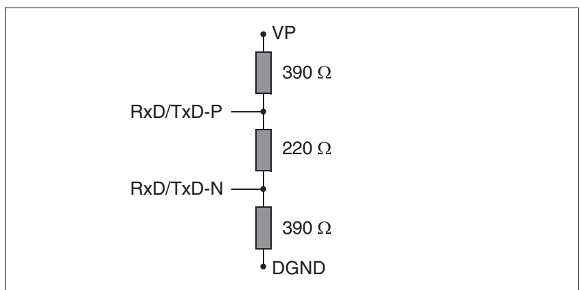
Bild 6.8 Abschlusswiderstand
