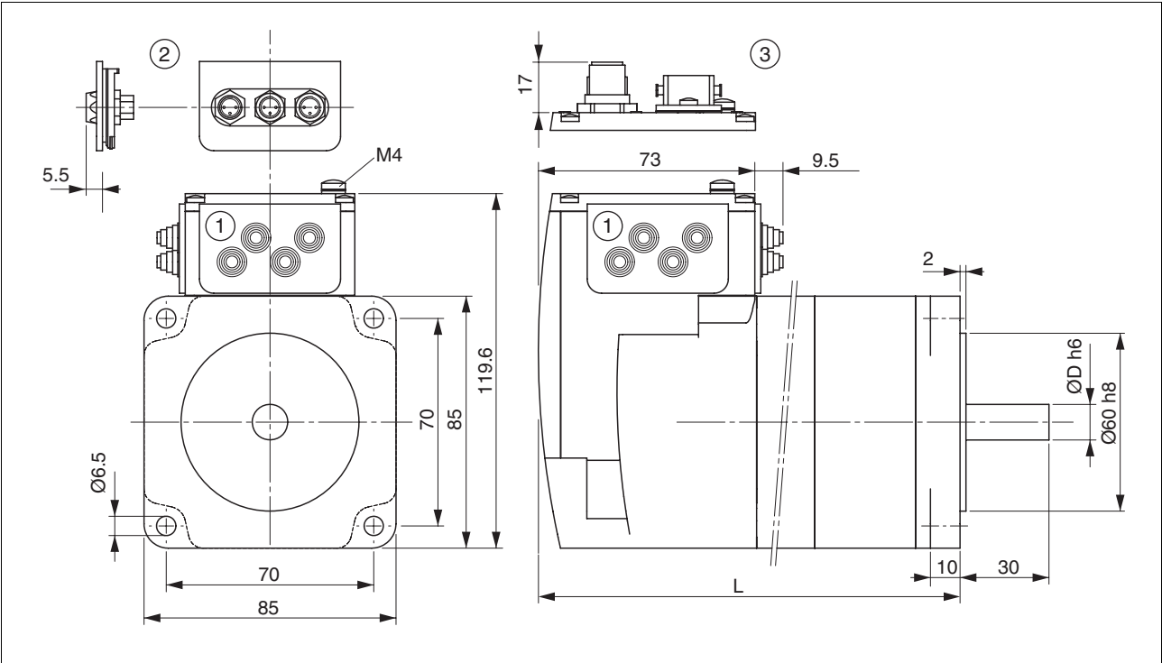
Bild 3.3 Abmessungen
