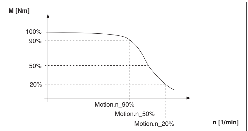
Bild 7.1 Typische Drehmomentkennlinie eines Schrittmotors
