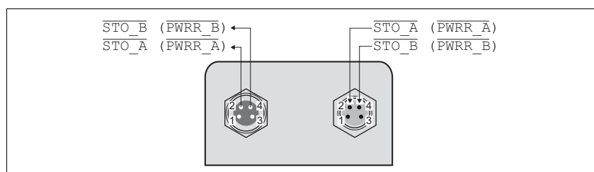
Bild 6.22 Pin-Belegung
