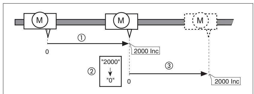
Bild 8.7 Positionierung um 4000 Inkremente mit Maßsetzen
