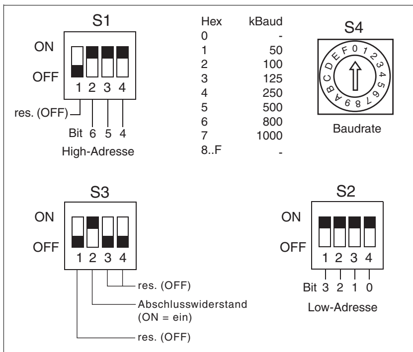
Bild 6.12 Parameterschalter
