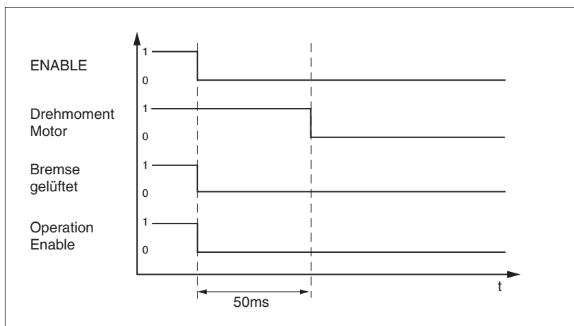
Bild 8.9 Schließen der Haltebremse
