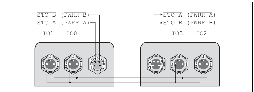
Bild 6.23 Pin-Belegung
