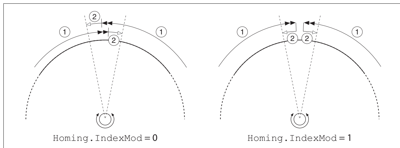
Bild 8.6 Referenzfahrt auf Indexpuls
