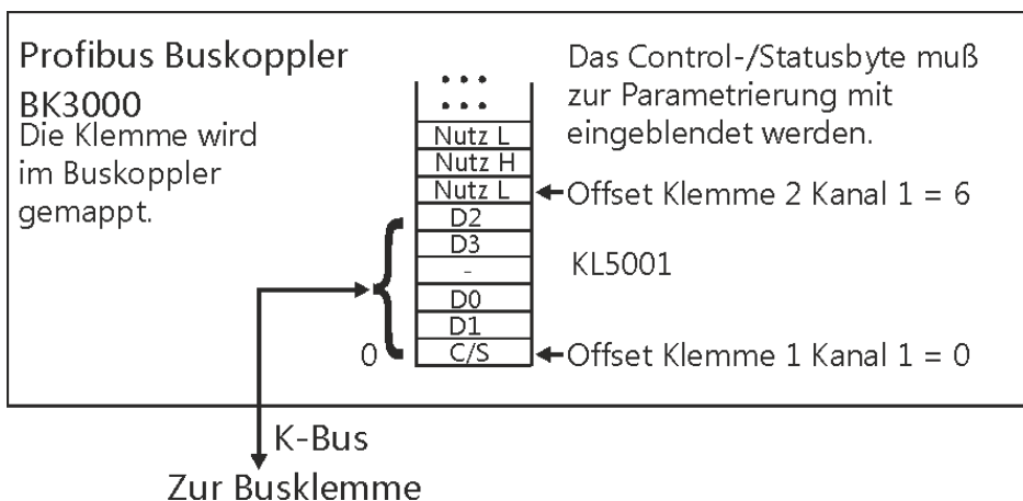
Abb. 14: Mapping im Profibus-Koppler - Beispiel für KL5001
