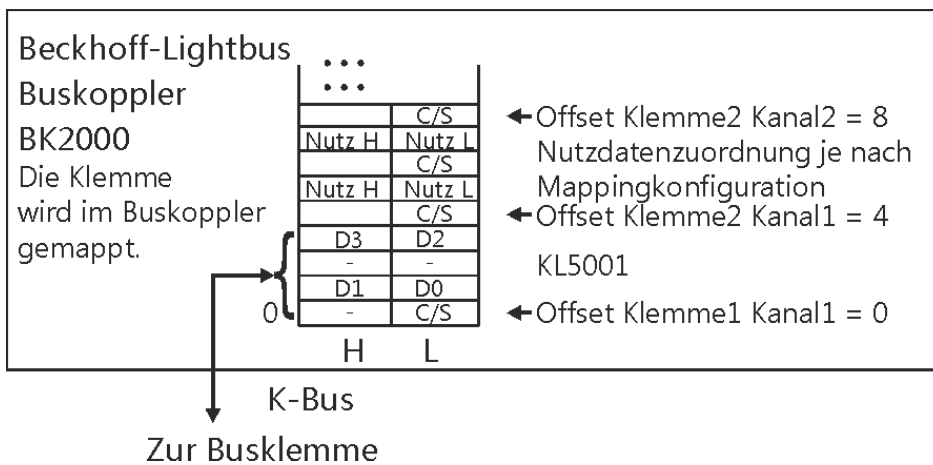
Abb. 13: Mapping im Lightbus-Koppler - Beispiel für KL5001
