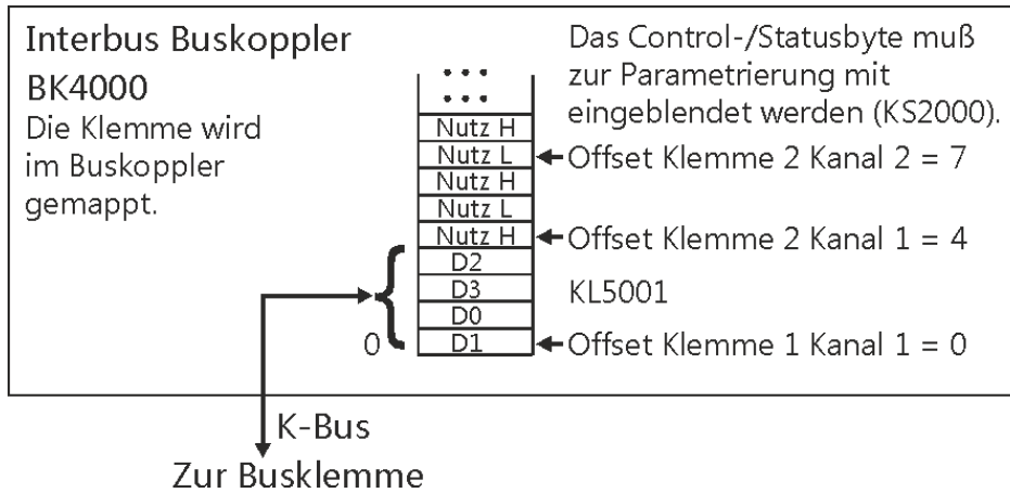
Abb. 15: Mapping im Interbus-Koppler - Beispiel für KL5001
