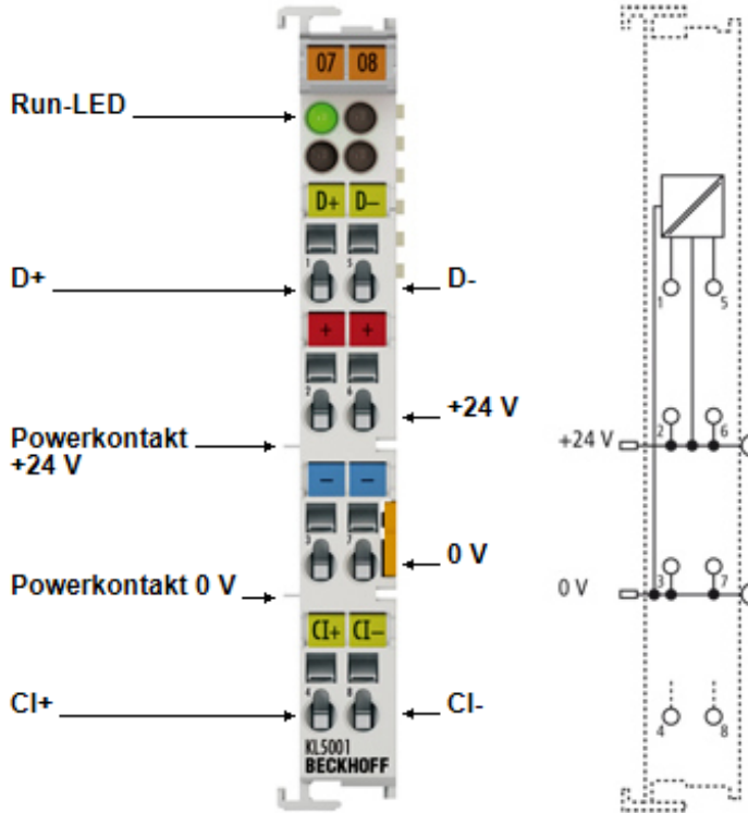
Abb. 11: KL5001 - Anschluss und LEDs
