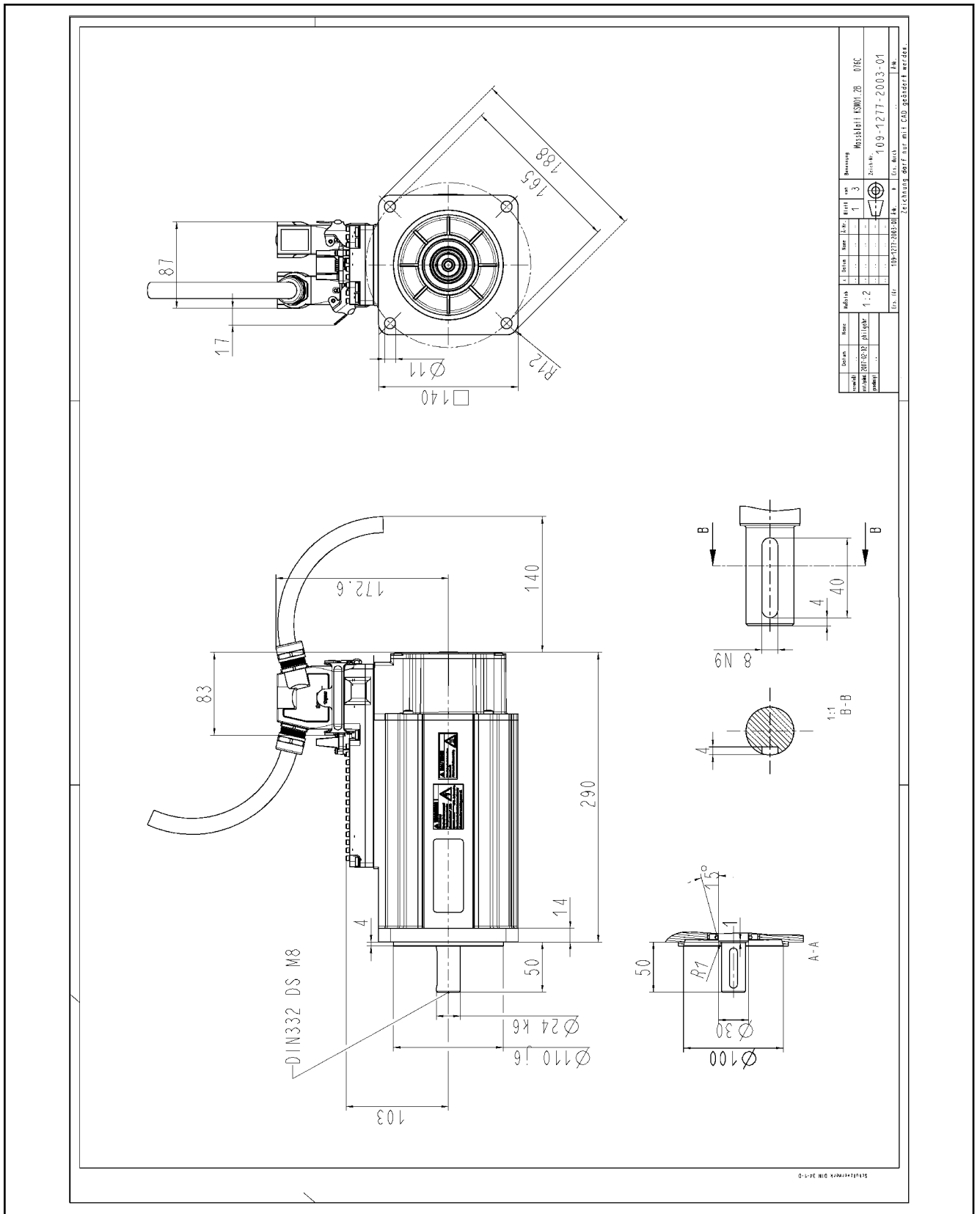
Abb.3-6: Abmessungen KSM01.2-076
