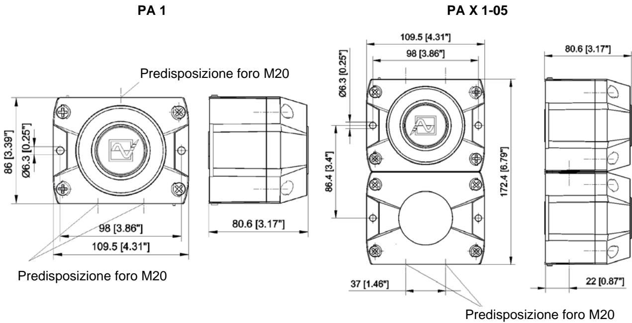
Schema forature interne all'alloggiamento (PA X 1-05)
