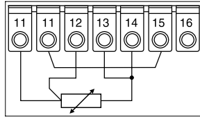
Conexión a 3 hilos
