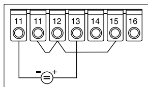
Entrée tension \pm 100 mV
