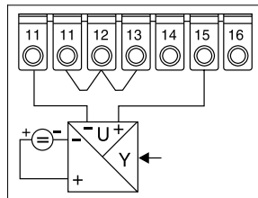
Connessione tensione 4 conduttori
