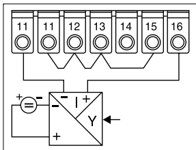
Connessione corrente 4 conduttori
