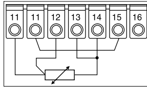
Connessione con 3 conduttori
