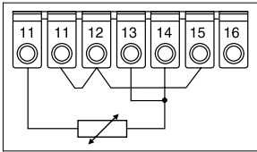
2-draads-aansluiting
