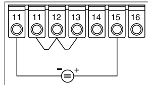
Spannungseingang +/- 10 V, 0...1/10 V
