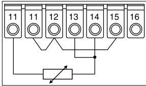
2-Leiter-Anschluss
