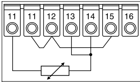
Connessione bifilare
