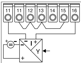
4-Leiter Strom-Anschluss
