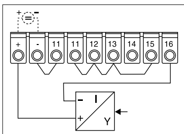
Conexión de intensidad con 2 hilos (alimentado por lazo)
