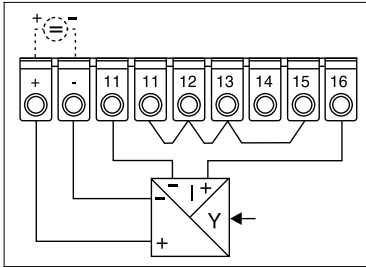
Raccordement courant 4 fils
