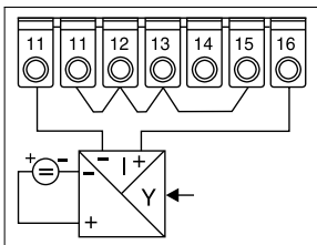
Raccordement courant 4 fils
