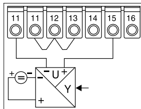
Conexión de intensidad a 4 hilos
