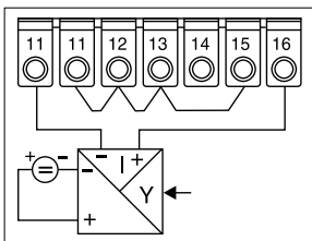
4-draads stroomaansluiting
