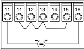
Stromeingang +/- 20 mA, 0/4...20 mA
