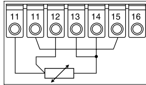
3-Leiter-Anschluss
