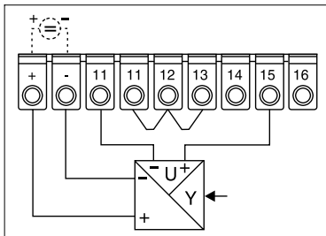
Connessione tensione 4 conduttori
