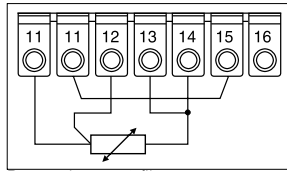
Raccordement 3 fils
