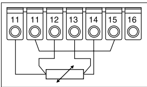
4-draads-aansluiting
