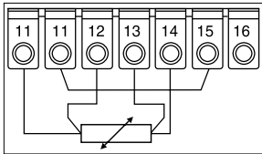
4-Leiter-Anschluss
