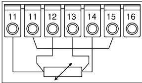
Conexión a 4 hilos
