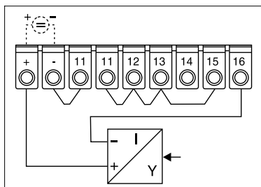
Connessione corrente bifilare (alimentazione del circuito)
