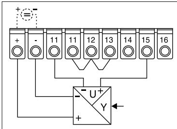
Raccordement tension 4 fils
