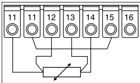
Connessione con 4 conduttori
