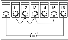
Entrada de intensidad \pm 20 mA, 0/4...20 mA
