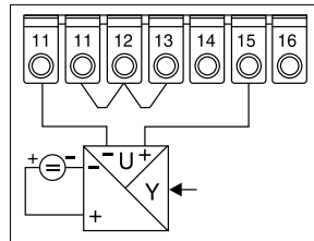
Raccordement tension 4 fils
