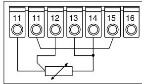
3-draads-aansluiting
