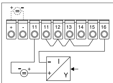
Conexión de intensidad con 2 hilos (alimentación externa)
