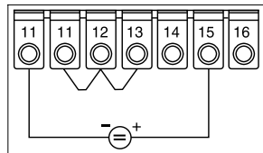
Entrada de tensión \pm 10 V, 0...1/10V
