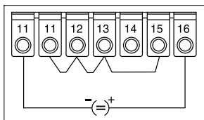
Entrée courant \pm 20 mA, 0/4 à 20 mA
