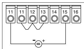
Entrée tension \pm 10 V, 0 à 1/10 V
