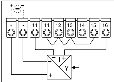
4-draads stroomaansluiting
