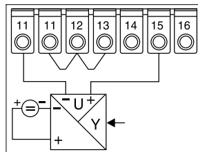
4-Leiter Spannungs-Anschluss
