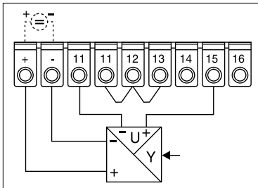
4-Leiter-Spannungsanschluss
