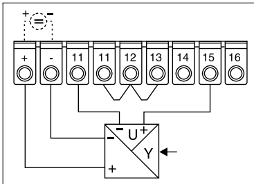
Conexión de intensidad a 4 hilos
