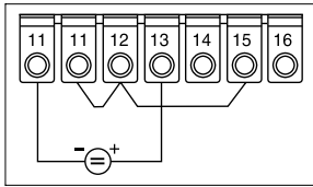
Spanningsingang \pm 100\text{mV}
