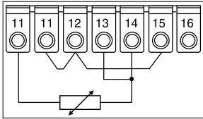
Conexión a 2 hilos
