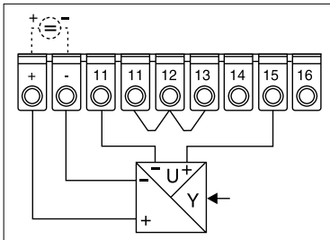
4-draads spanningsaansluiting
