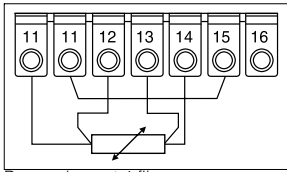
Raccordement 4 fils
