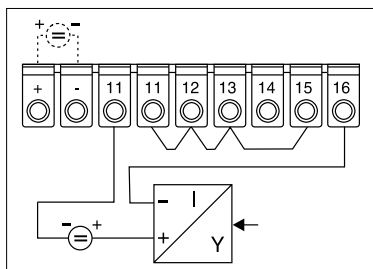
Connessione corrente bifilare (alimentazione esterna)
