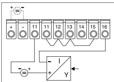
2-draads stroomaansluiting (Loop powered)
