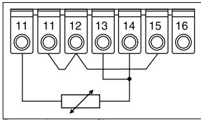
Raccordement 2 fils
