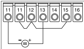
Spannungseingang +/- 100 mV
