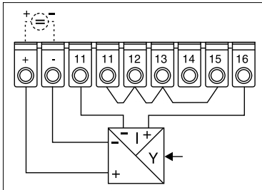
4-Leiter Strom-Anschluss
