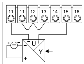
4-draads spanningsaansluiting
