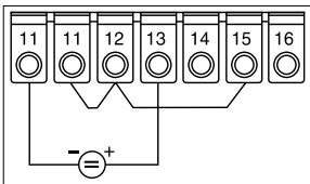
Entrada de tensión \pm 100 mV
