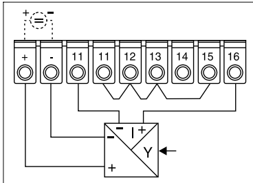
Connessione corrente 4 conduttori
