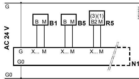
Schaltplan 1: Messteil mit passiven Haupt- und Hilfsfühlern und passivem Geber
