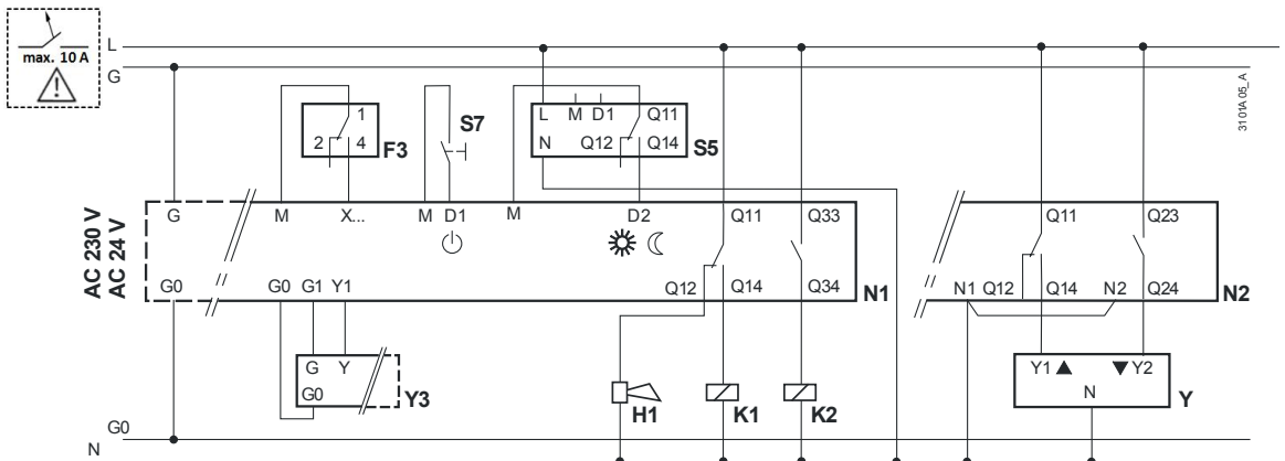
Schaltplan 5:
