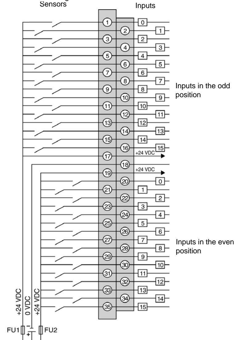
TSX DEZ 32D2 diagram: Sensors
